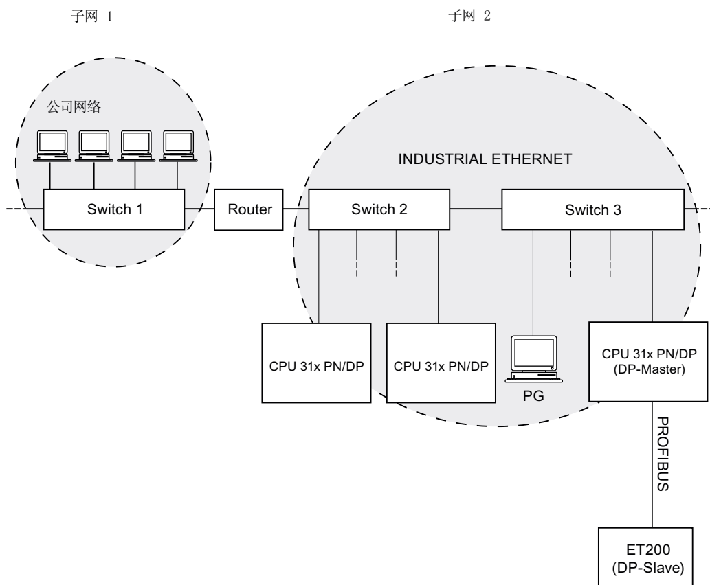
图 4-8 PROFINET 子网实例
