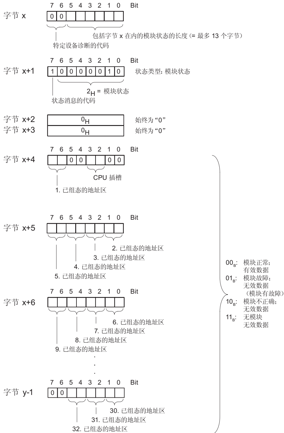
图 10-6 CPU 31xC 的模块状态的结构
