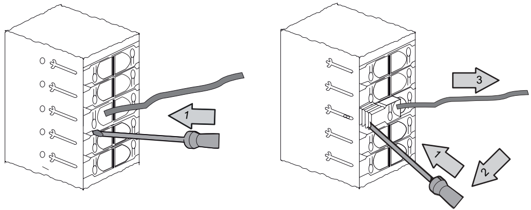
图 6-2 断开使用 40 针快速连接连接器进行的接线
