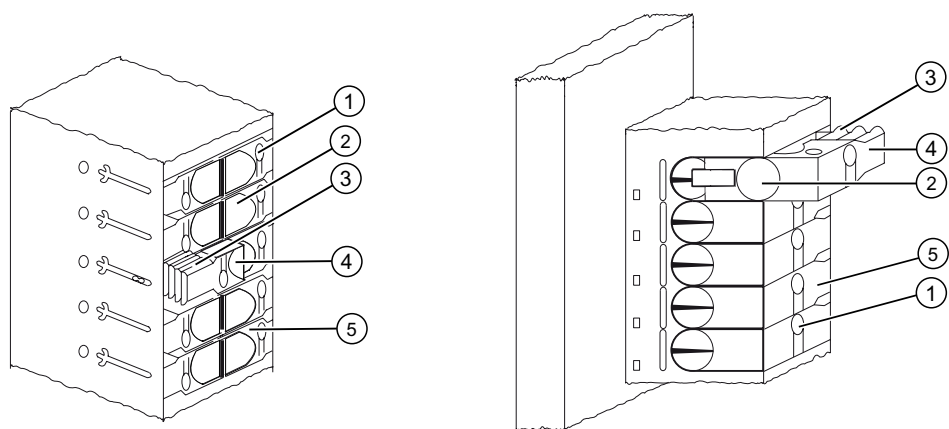
图 6-1 “快速连接”连接器的原理图表示
