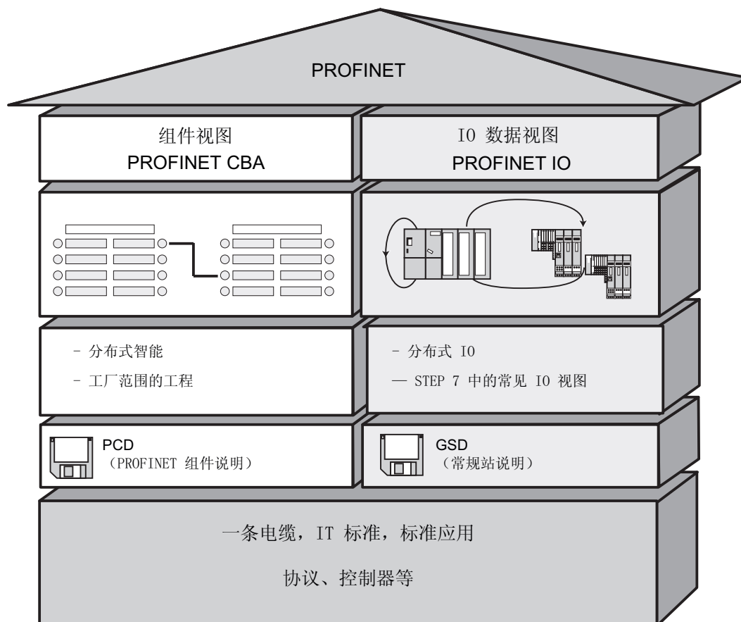
图 4-7 PROFINET CBA 和 PROFINET IO 的范围
