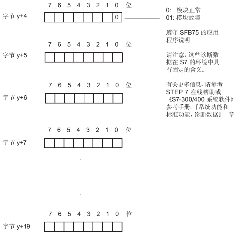
图 10-9 诊断中断的字节 y+4 到 y+19 ( SFB75 )
