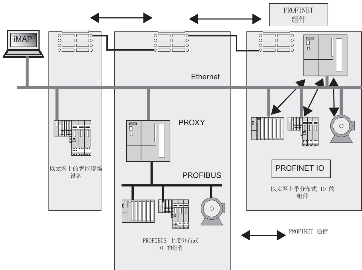
图 4-6 PROFINET CBA — 模块化概念
