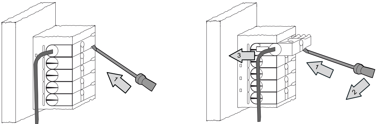
图 6-3 断开使用 20 针快速连接连接器进行的接线
