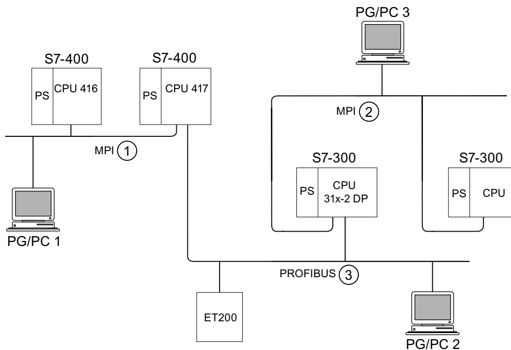
图 4-9 对远程网络的访问
