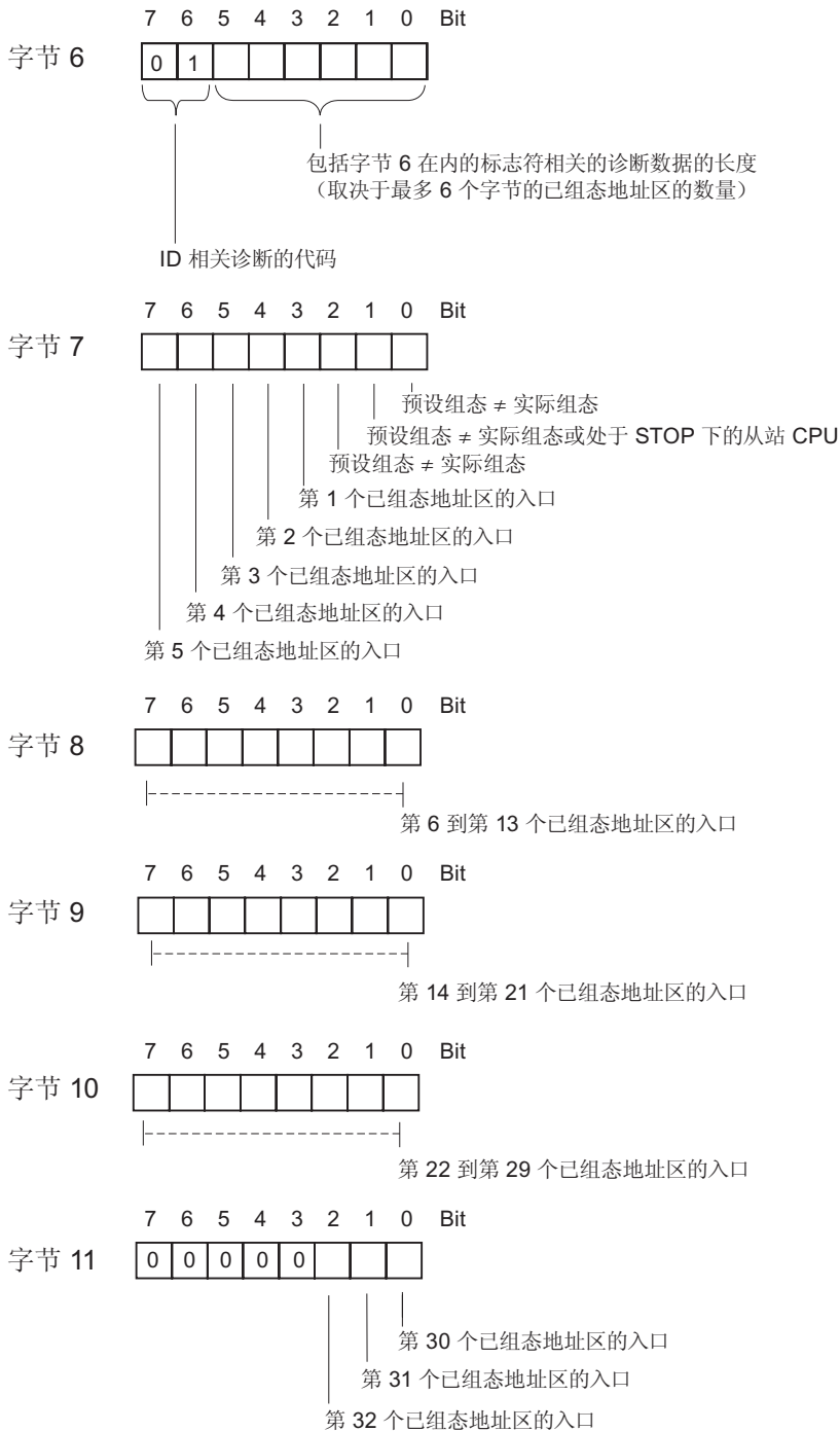
图 10-5 标识符相关的诊断数据
