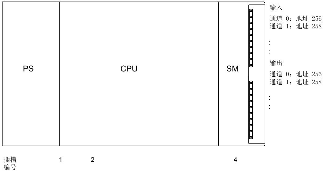
图 7-1 位于插槽 4 的模拟模块的 I/O 地址
