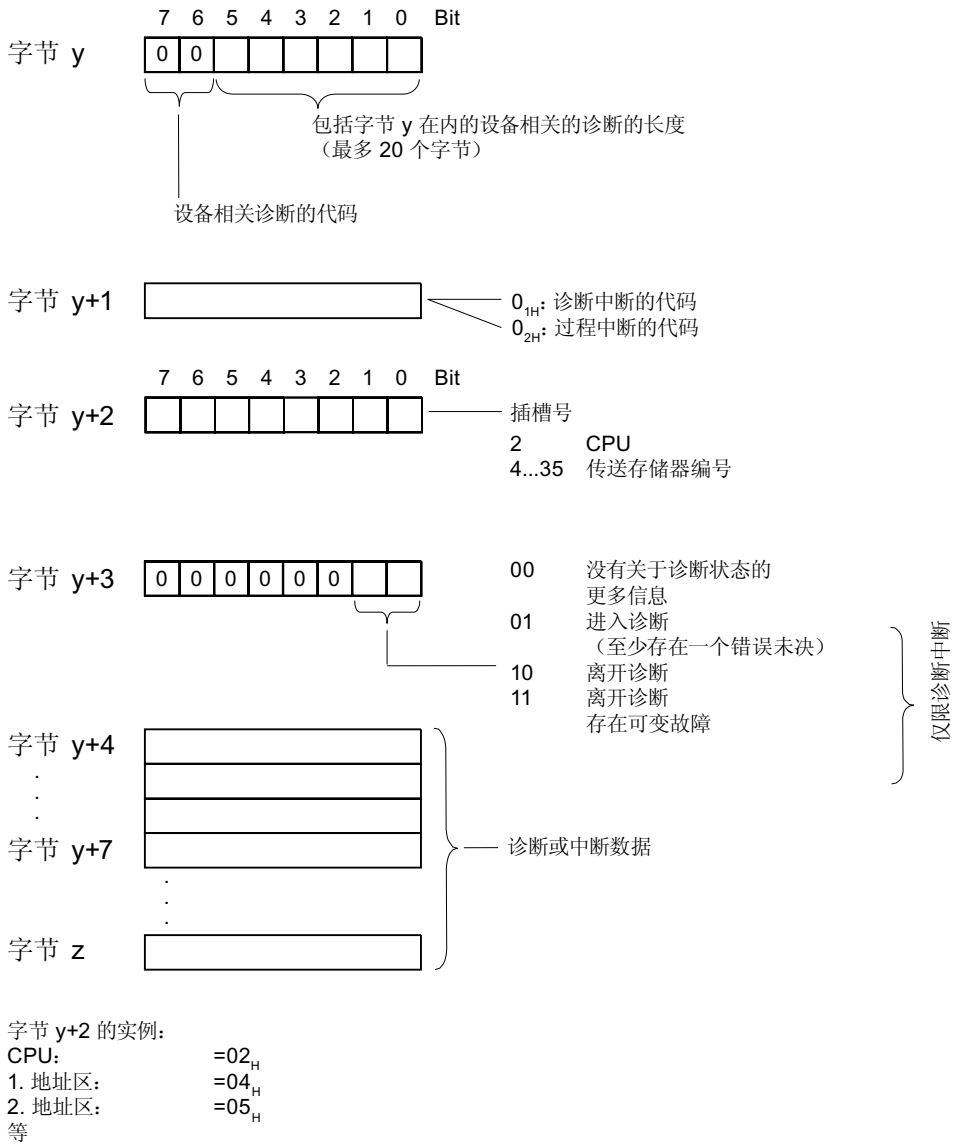
图 10-7 设备专用的诊断信息
