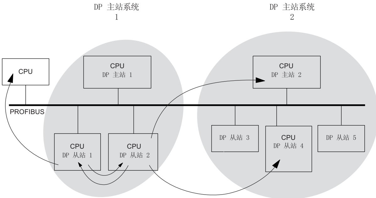
图 8-1 通过 DP CPU 进行直接数据交换
