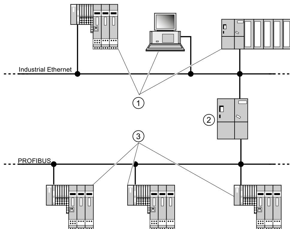
图 4-5 PROFINET 设备、PROFIBUS 设备和代理
