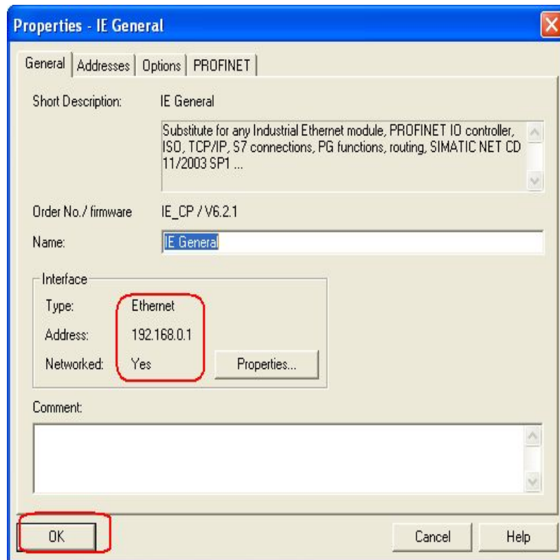
图 14: 以太网卡参数设置
