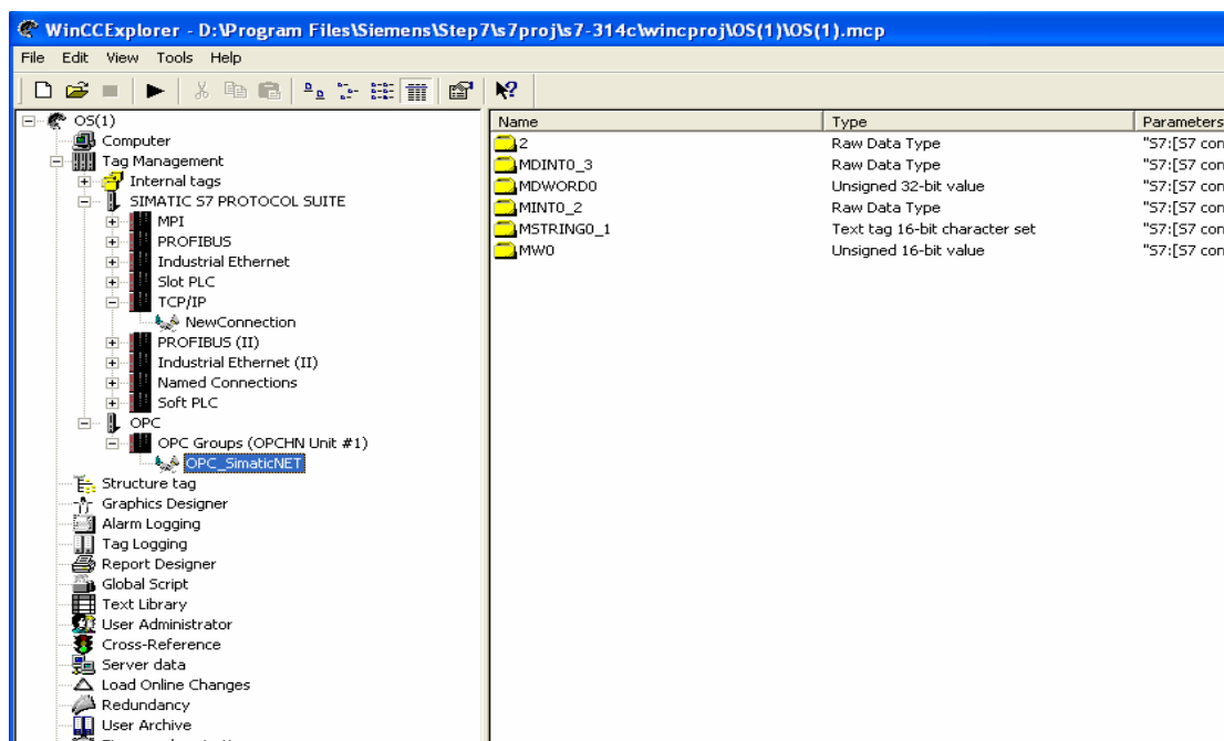
图 35 完成 OPC 过程变量的添加
