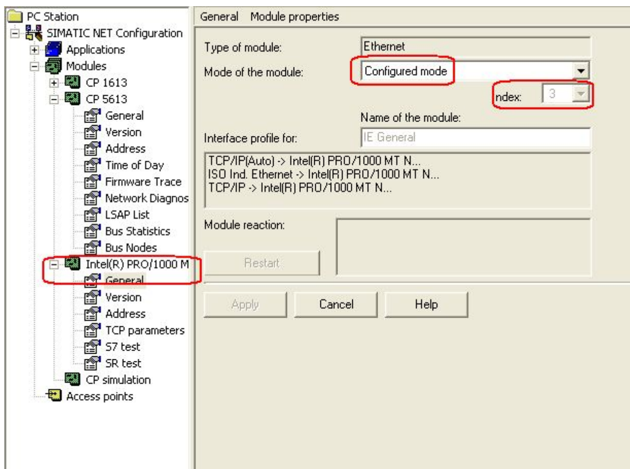
图 10 配置控制台（Configuration Console）
