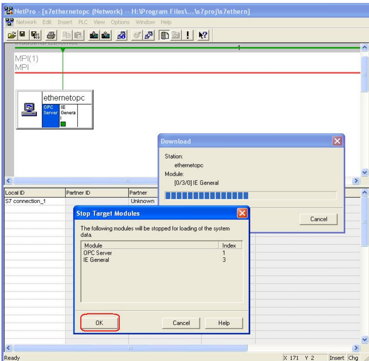
图 21：组态下载
