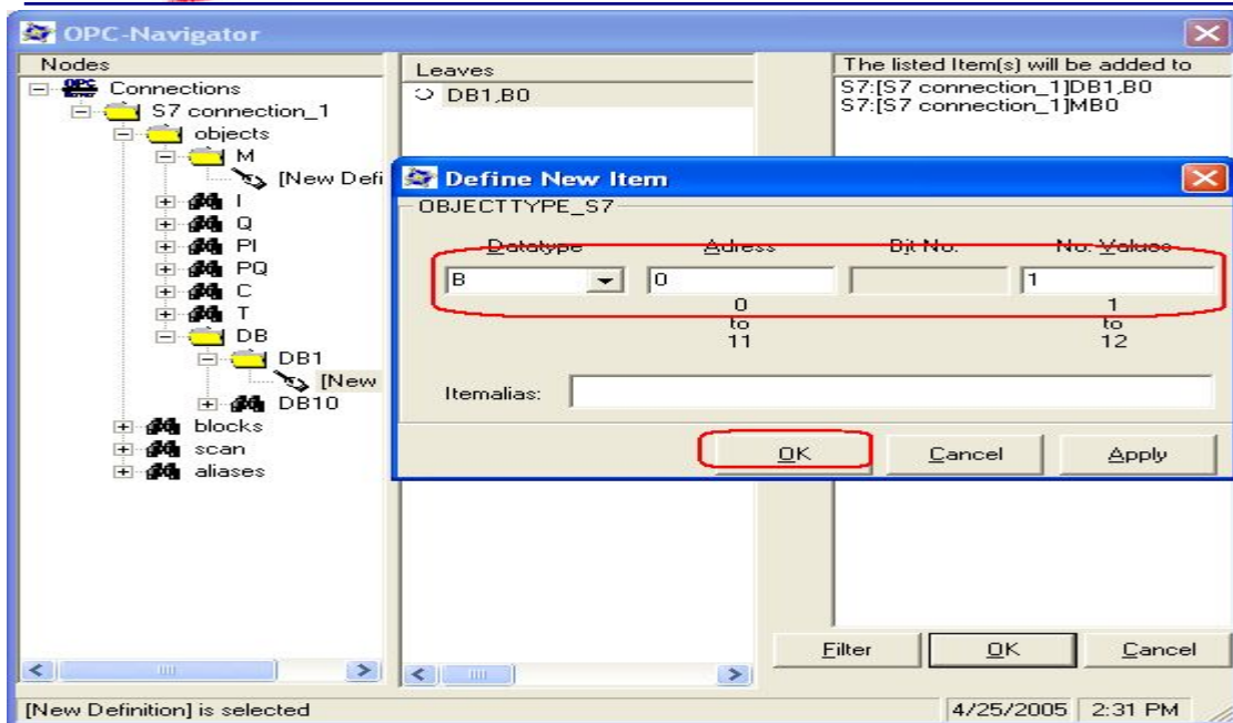
图 25: 定义条目及标签变量
