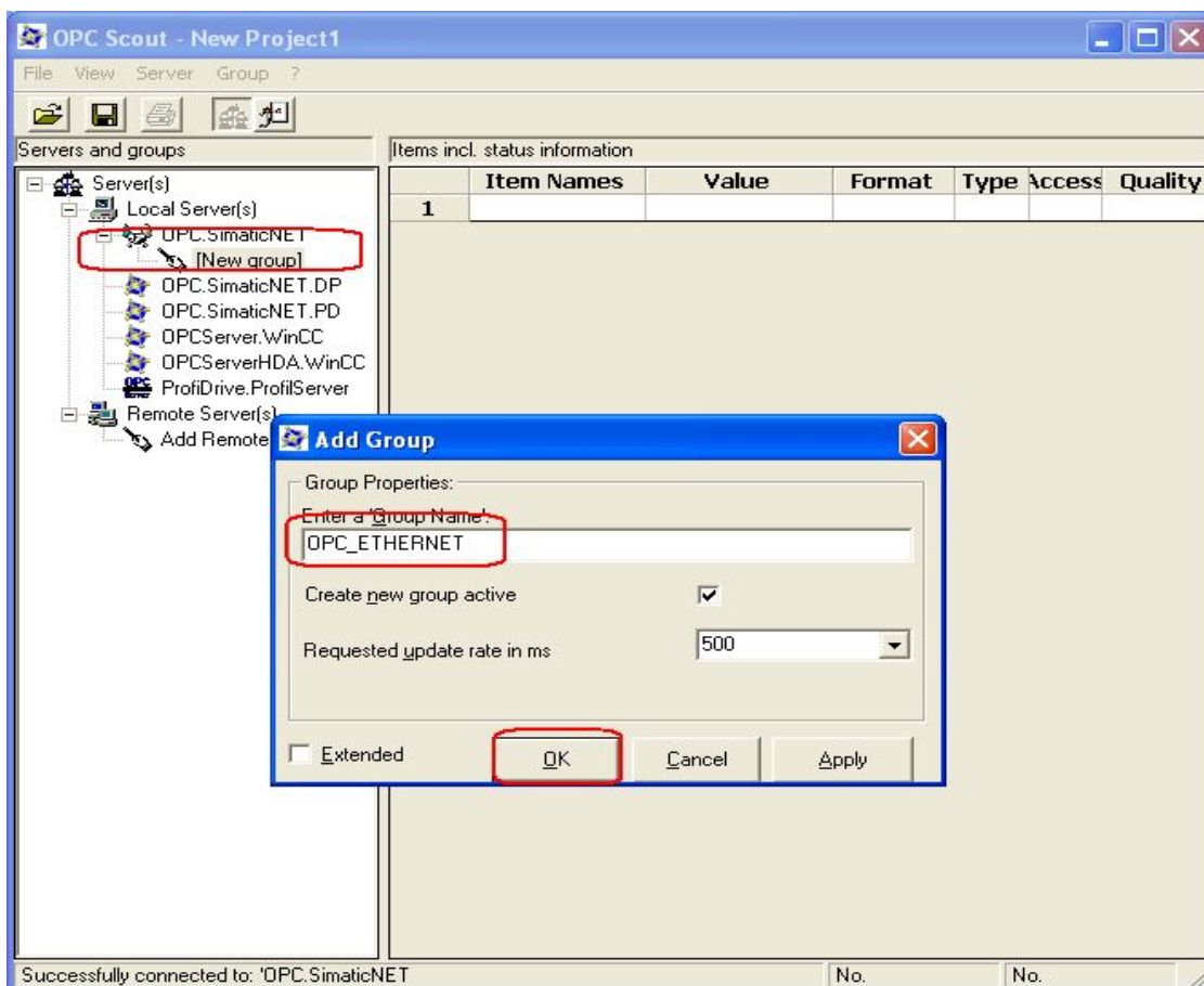
图 23： 在 OPC Scout 中添加一个组“OPC_ETHERNET”
