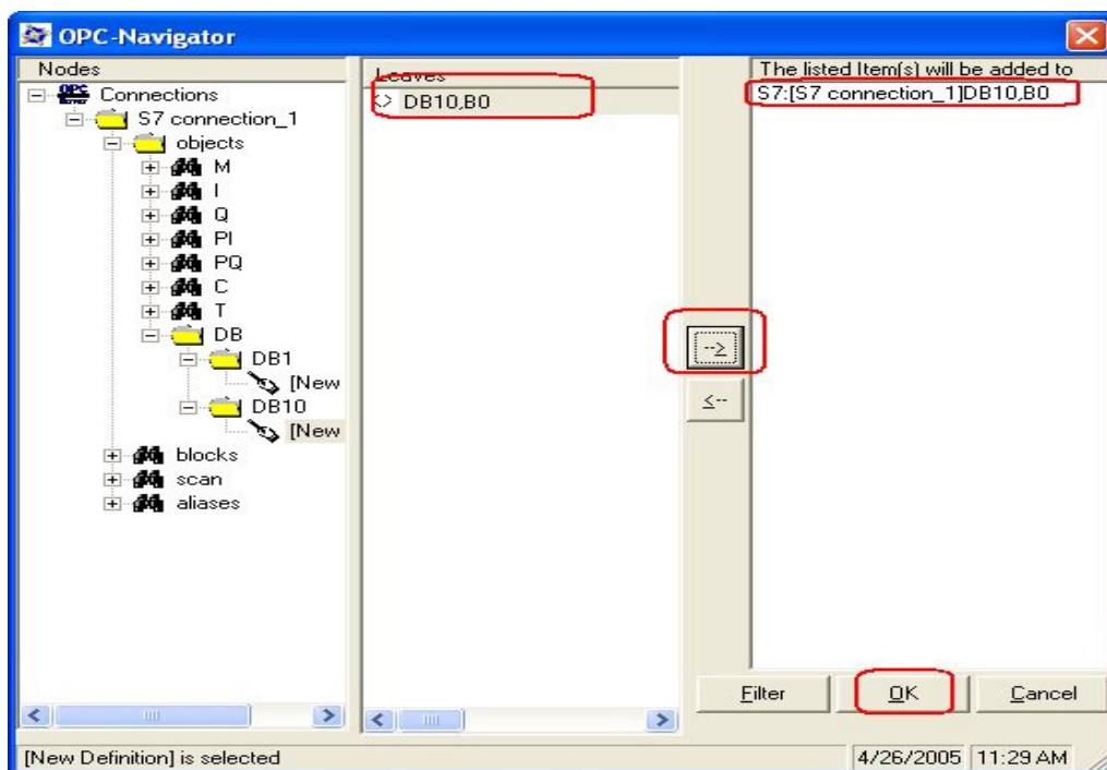
图 26: 建立定义条目与 OPC Server 连接
