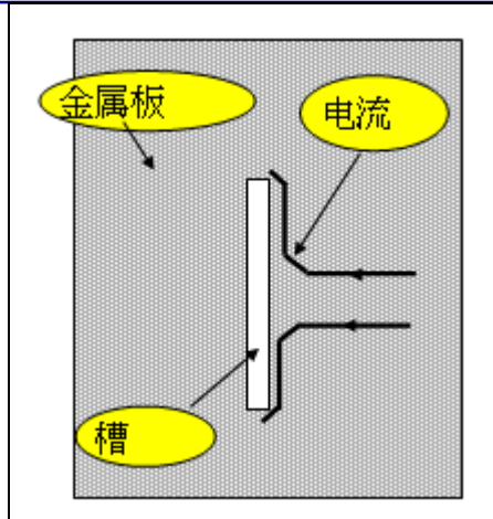
图 1-23 缝隙天线
