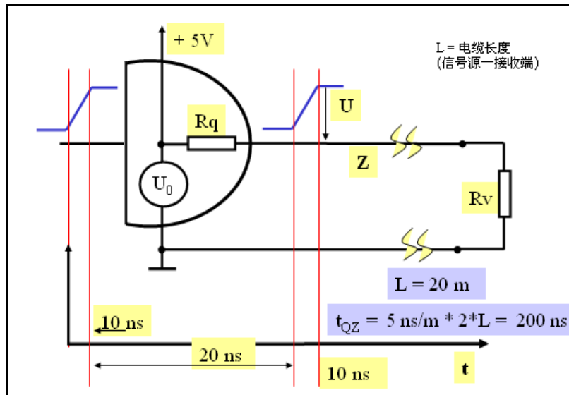
图 1-7 信号反射
