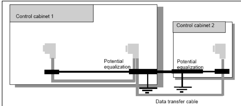
图 4-7 PROFIBUS 屏蔽层接地 3
