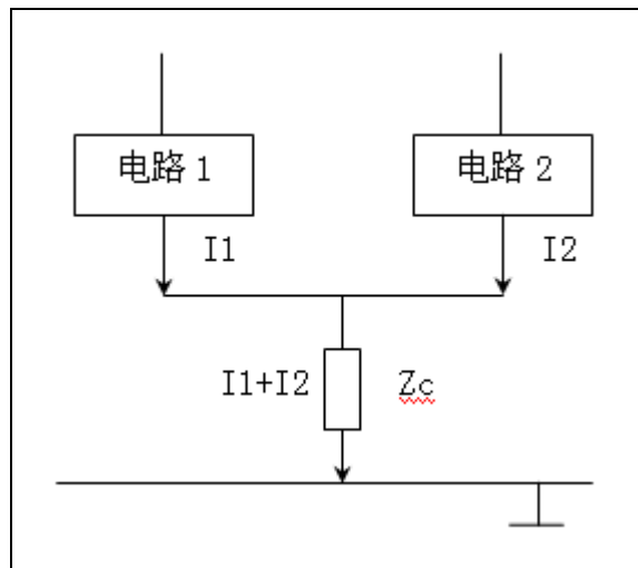
图 1-6 共阻抗耦合
