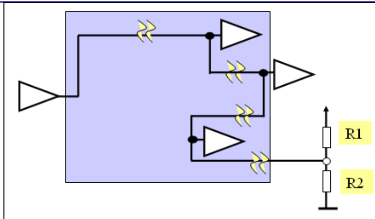
图 1-10 终端电阻的配置 2
