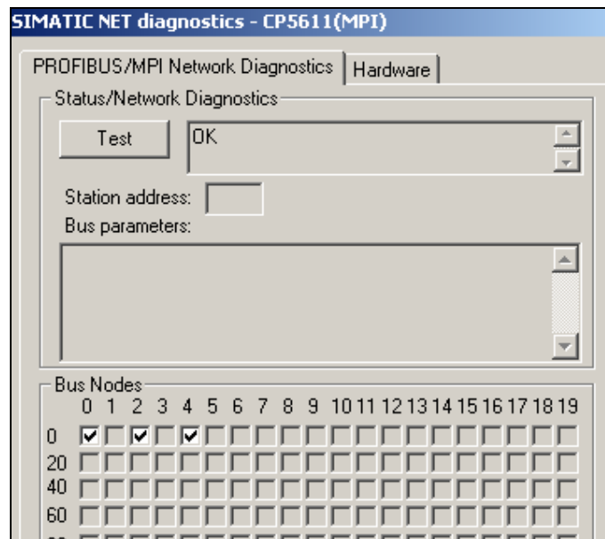
图 7 使用网卡诊断站号
