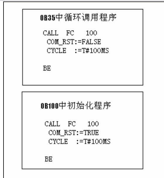
图 12 FM355 模块循环调用和初始化程序
