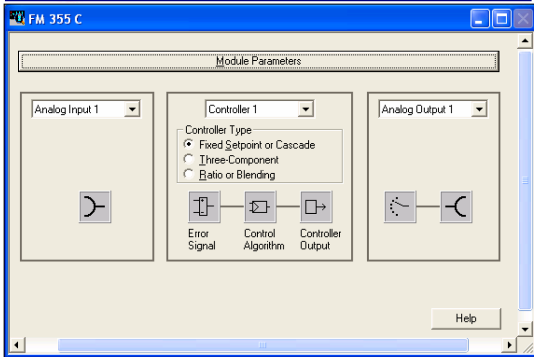
图 7 FM355 模块 参数化界面
