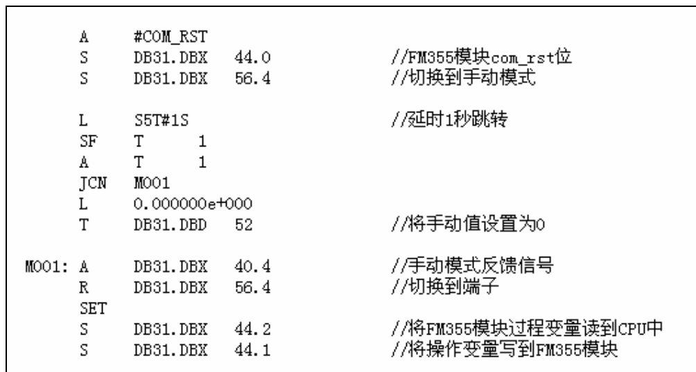
图 13 FM355 函数 FC100 PID 回路初始化程序
