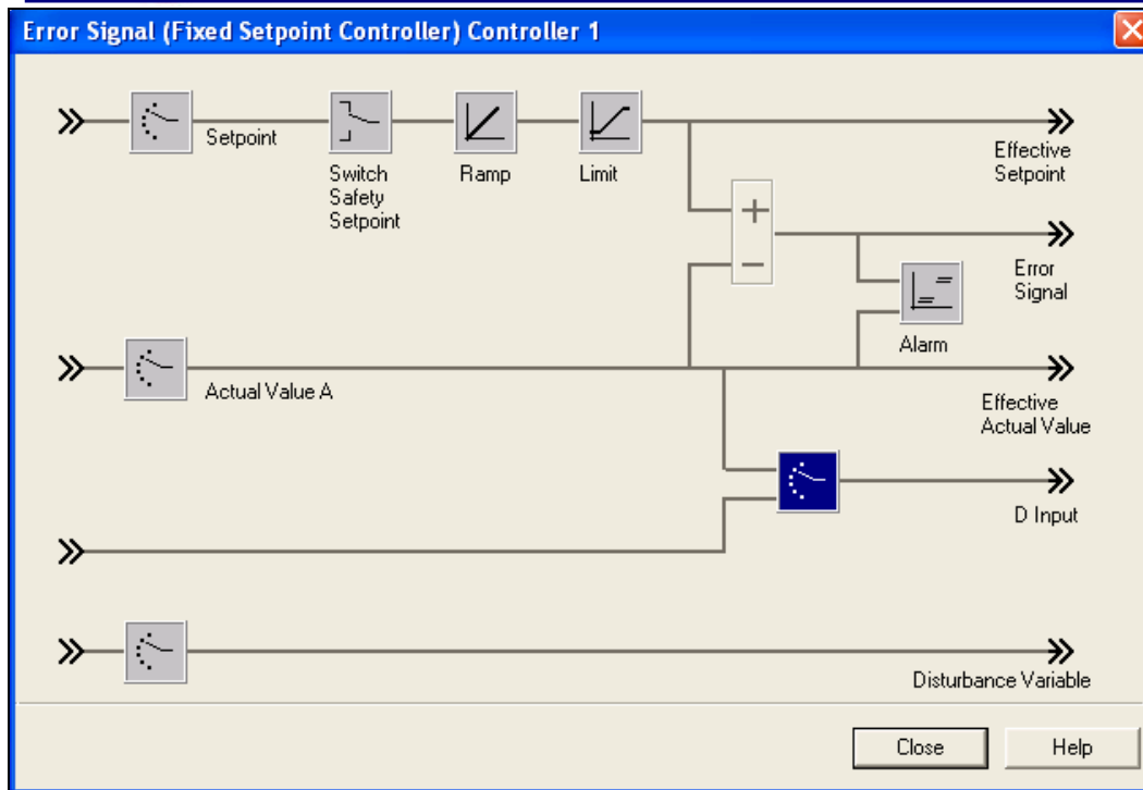
图 9 FM355 模块偏差 参数化界面
