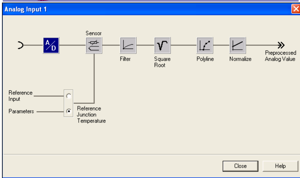
图 8 FM355 模块过程值 参数化界面
