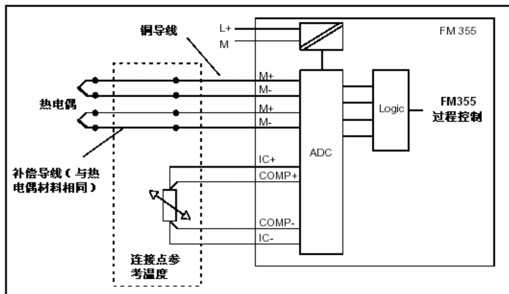
图 5 连接热电偶传感器—外部补偿
