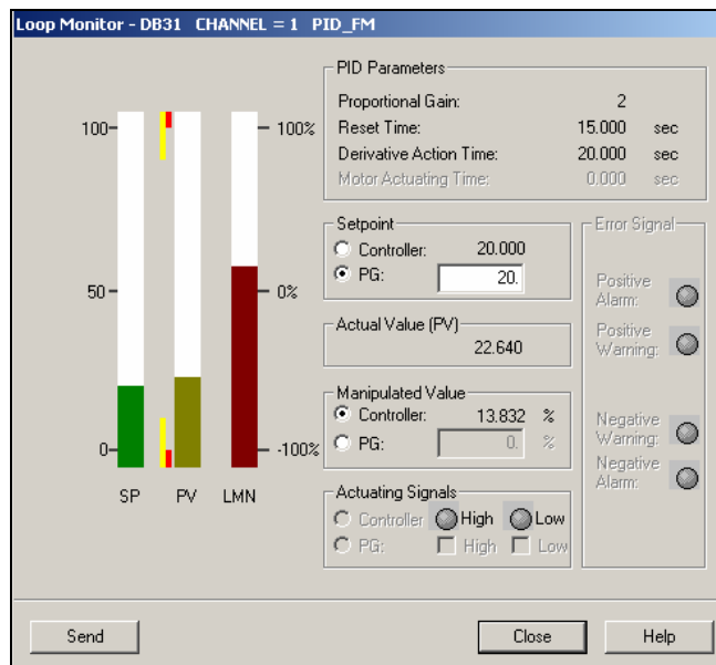
图 14 FM355 回路监控监控界面
