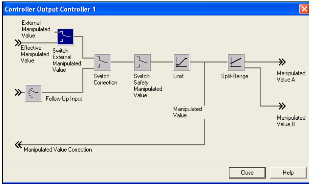
图 11 FM355 模块控制回路输出参数化界面
