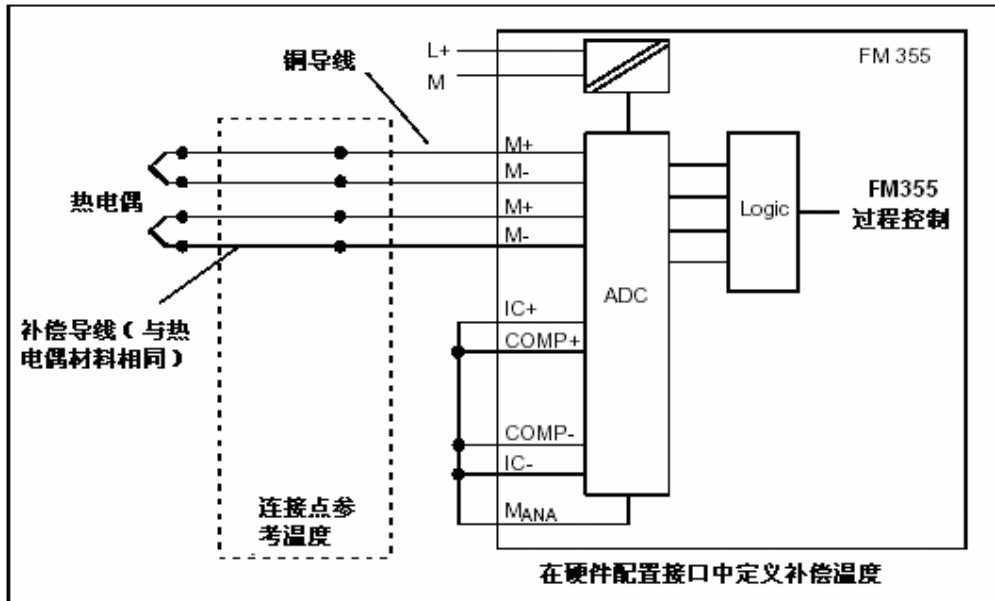
图 6 连接热电偶传感器—内部部补偿
