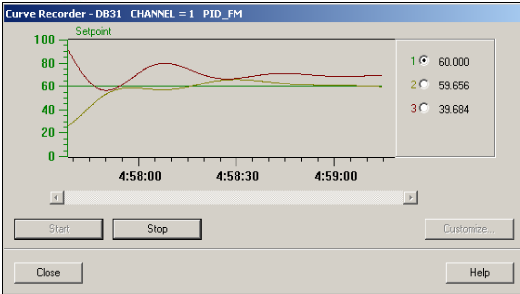
图 15 FM355 参数曲线界面
