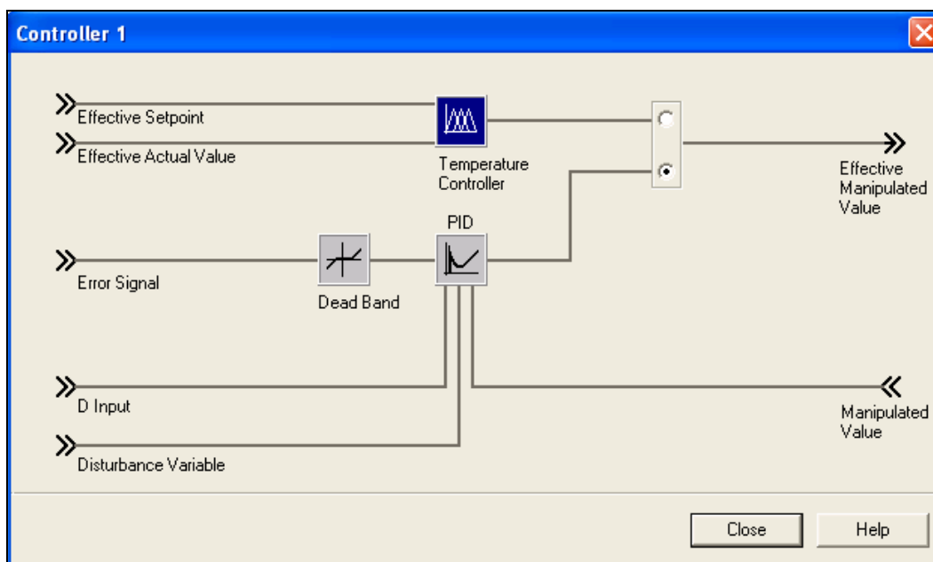
图 10 FM355 模块控制算法参数化界面
