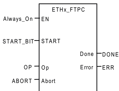
图 4-5 调用 ETHx_FTPC 子程序
