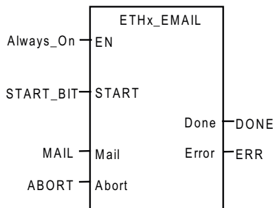
图 4-4 调用 ETHx_EMAIL 子程序
