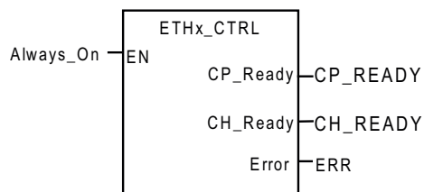
图 4-1 调用 ETHx_CTRL 子程序
