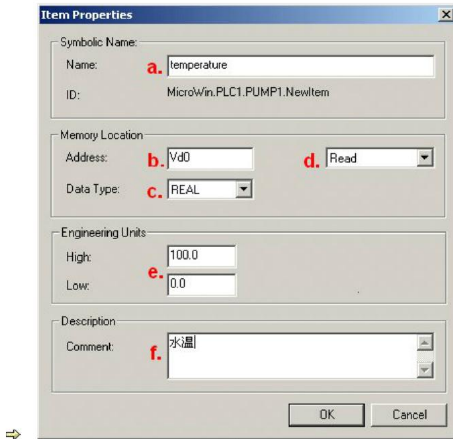
图 5. 添加 Item
