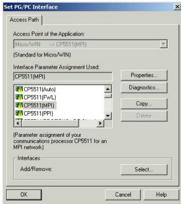
图 2. 选择 CP 卡
