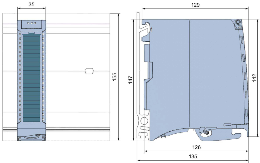
图 A-1 DI 16x24...125VUC HF 模块的尺寸图
