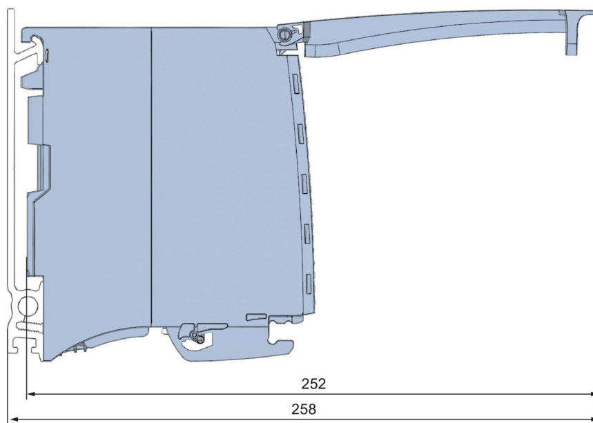
图 A-2 DI 16x24...125VUC HF 模块的尺寸图，前盖板打开时的侧视图
