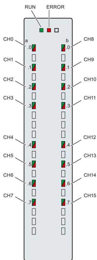
图 5-1 DI 16x24...125VUC HF 模块的 LED 指示灯
