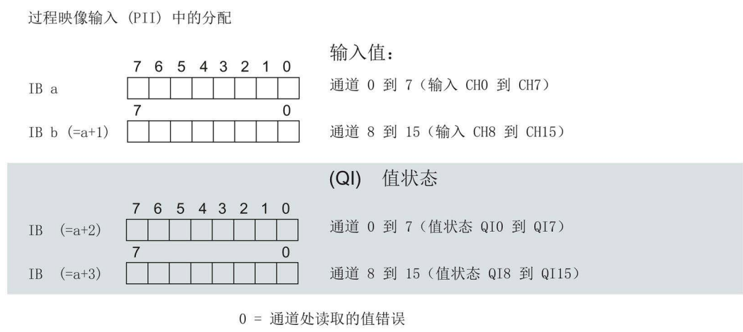
图 4-1 组态为 16 通道 DI 16x24...125VUC HF QI 的地址空间 (带值状态)
