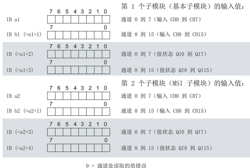
图 4-3 组态为 1 x 16 通道 DI 16x24...125VUC HF MSI 的地址空间
