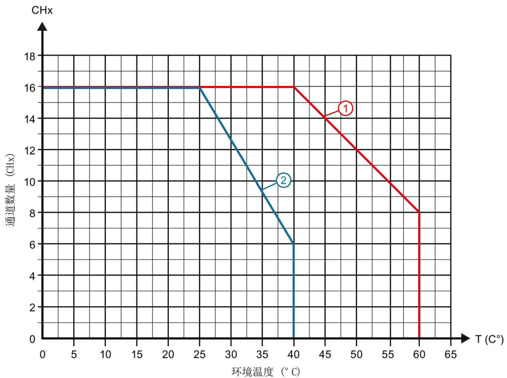
图 6-1 每个模块中可同时使用的通道数量：
