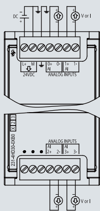
6ES7 231-4HD32-0XB0
