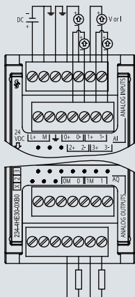
6ES7 234-4HE32-0XB0
