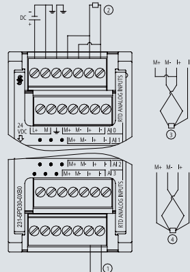
6ES7 231-5PD32-0XB0
