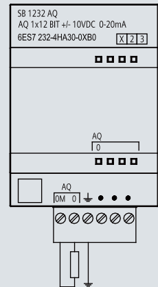
6ES7 232-4HA30-0XB0
