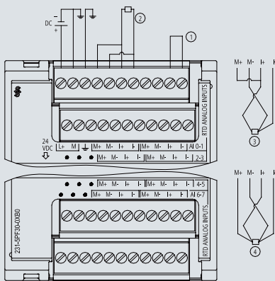
6ES7 231-5PF32-0XB0
