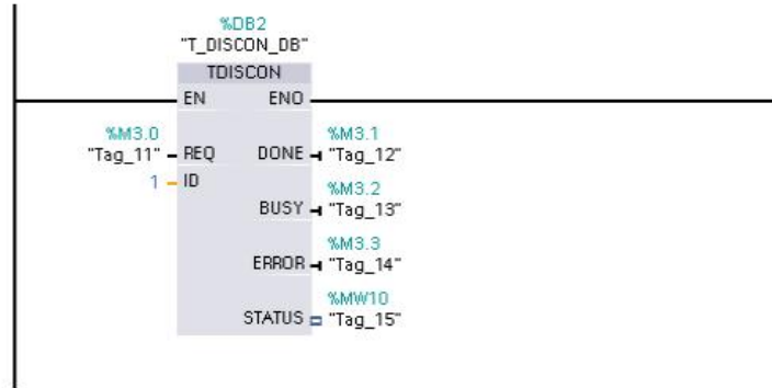
图 9 : TDISCON 函数块
