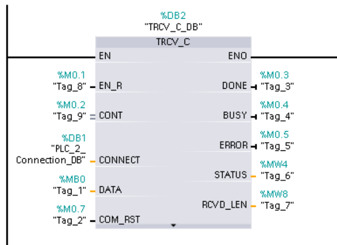
图 7：TRCV_C 函数块
