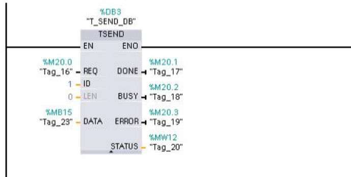
图 10 : TSEND 函数块
