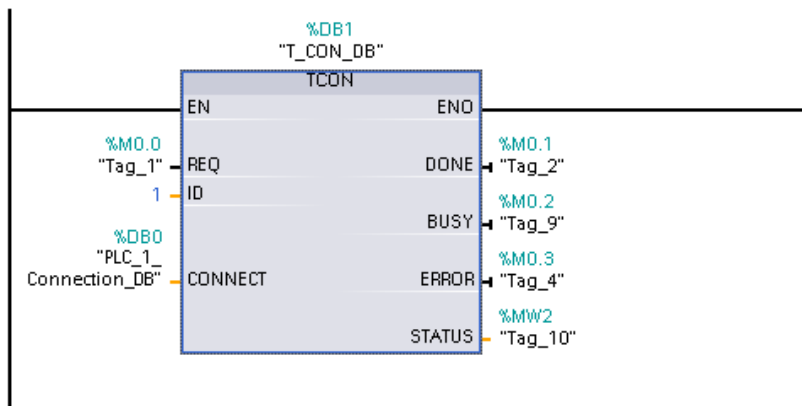
图 8：TCON 函数块
