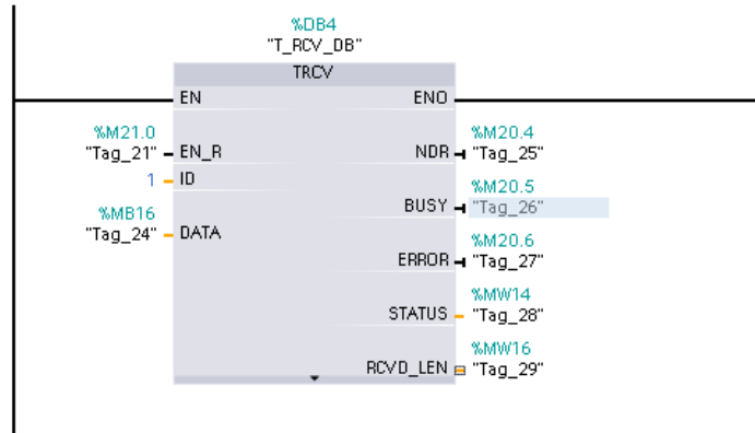
图 11 : TRCV 函数块
