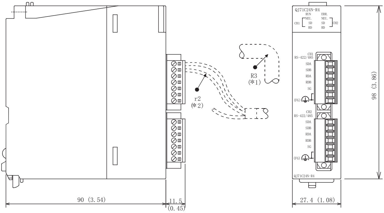
(3) QJ71C24N-R4
