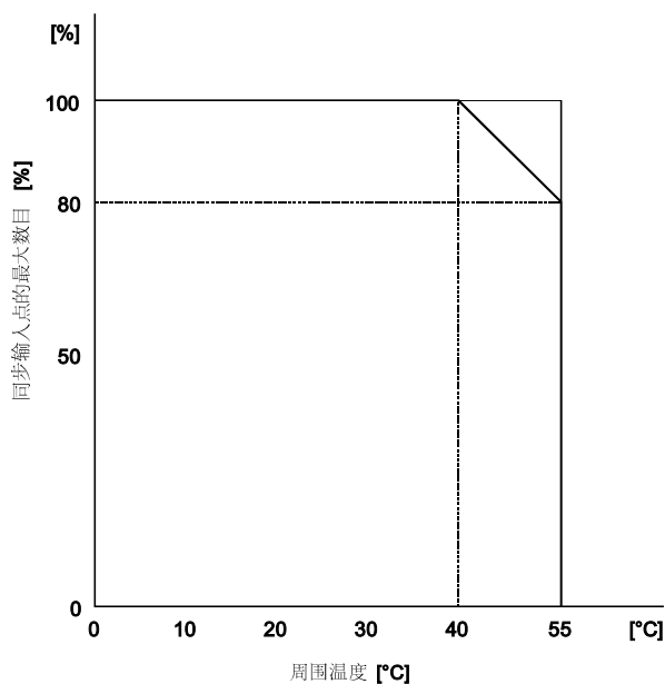
AJ65SBTC1-32D 或 AJ65SBTC1-32D1 型的额定度降低曲线
