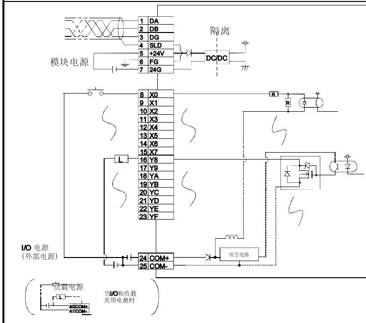
外部连接 (漏型输入)
