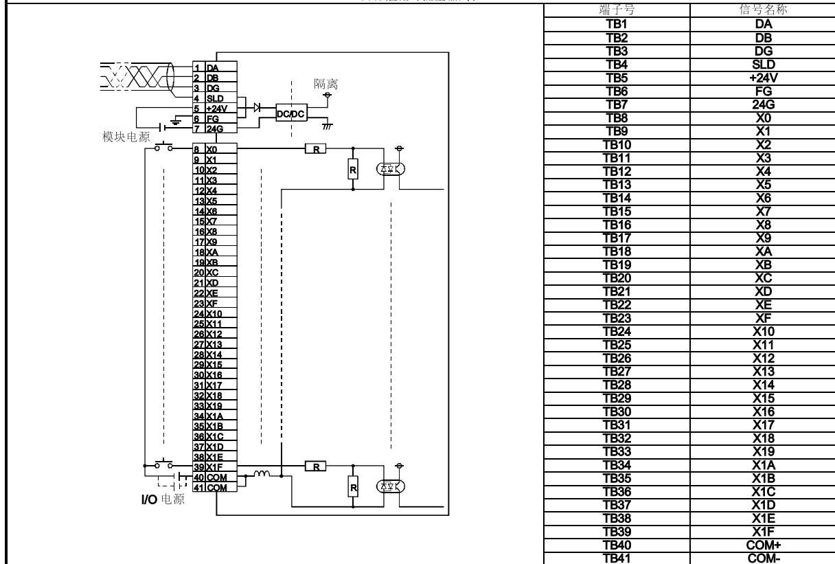
外部连接 (漏型输入)
