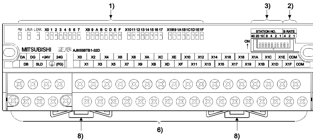
AJ65SBTB1-32 □ (32 点端子排模块, 单线)
