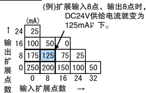
FX2N-16~32M
