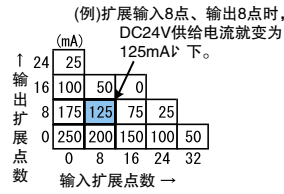
FX2N-32E
