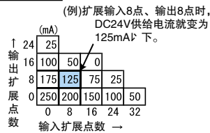
FX2N-32E
