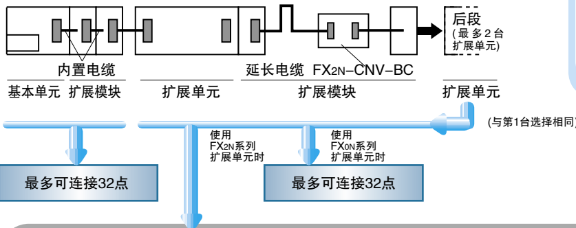
FX2N-32E(AC电源型)
