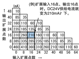
FX2N-48~128M
