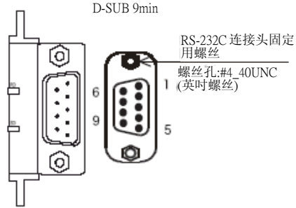
FX3U-232-BD
