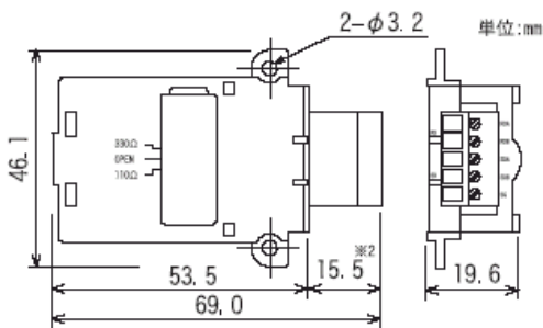
FX3U-CNV-BD
