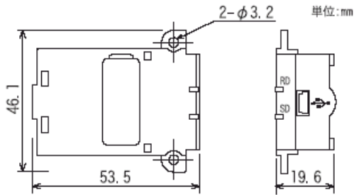
FX3U-232-BD
