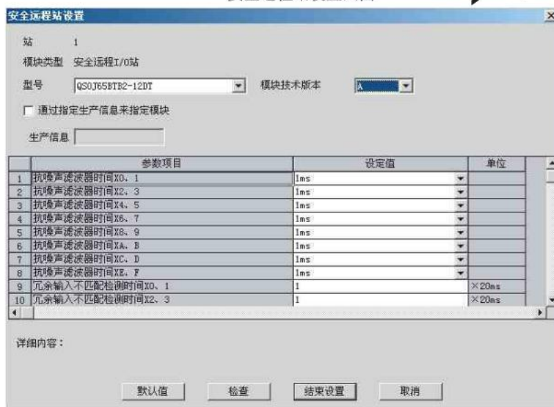
安全远程站设置画面
