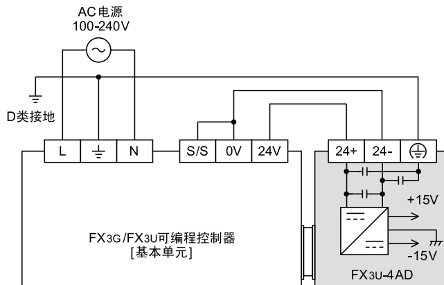
基本单元的 [S/S]端子和 [0V]端子连接。
