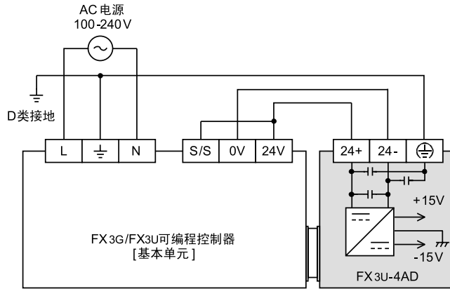
基本单元的 [S/S]端子和 [24V]端子连接。
