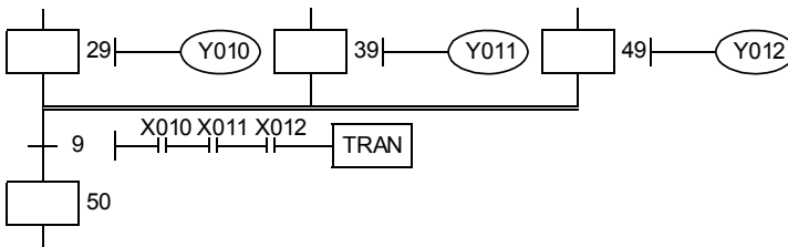
《步进梯形图》
