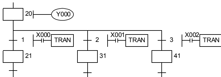
《步进梯形图》
