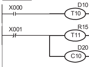
梯形图程序
