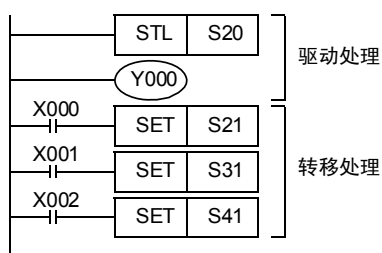
《步进梯形图》
