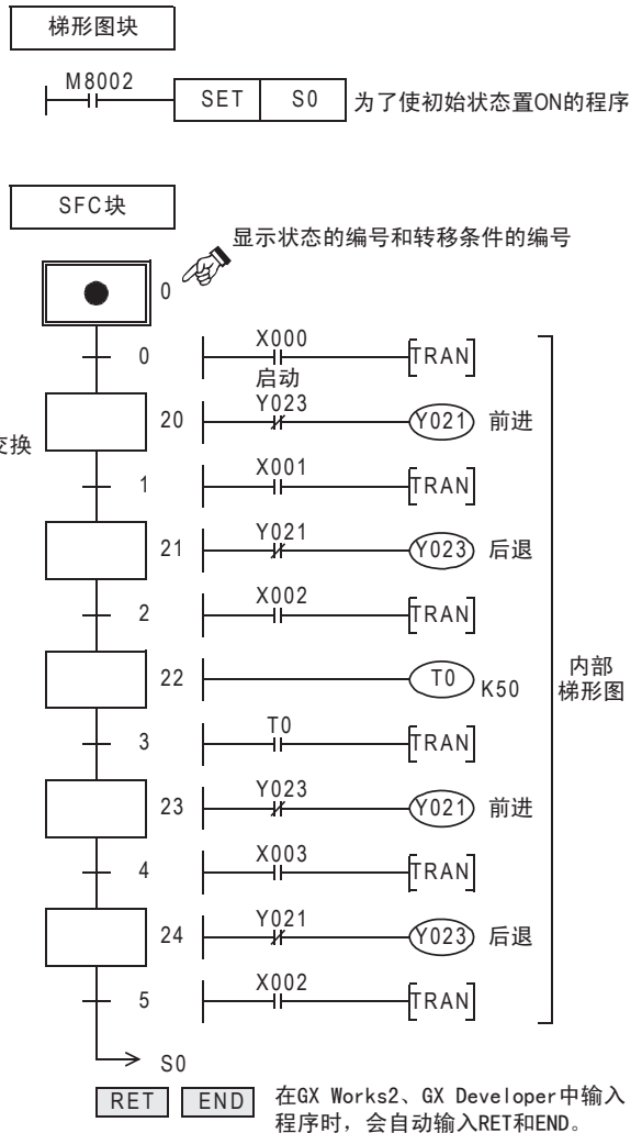
《SFC程序》
