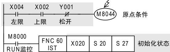
梯形图块
