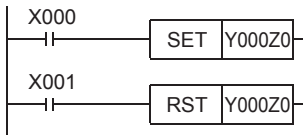
梯形图程序
