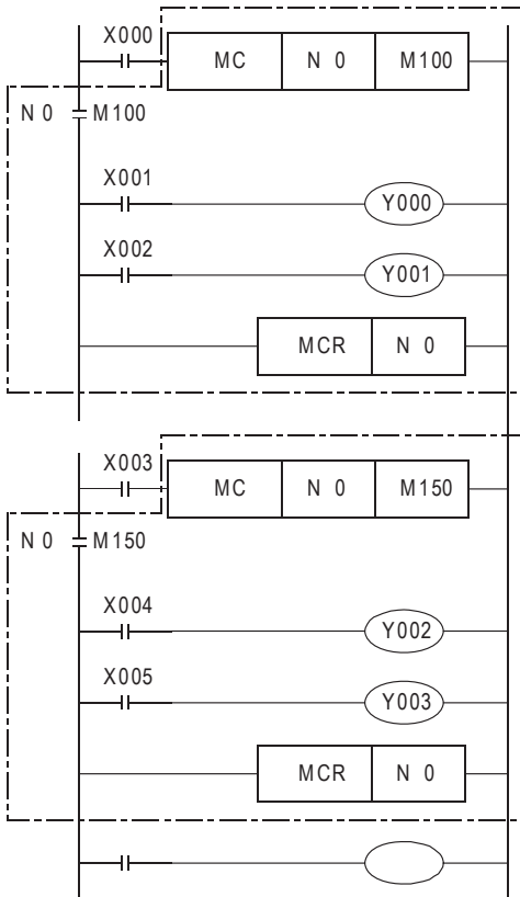
梯形图程序
