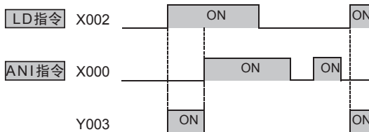
时序图
