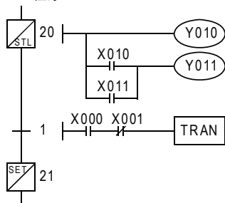
《SFC程序》
