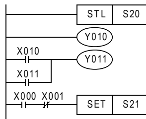
《步进梯形图》
