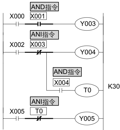
梯形图程序
