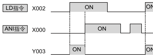
时序图
