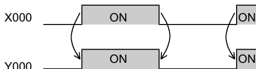
时序图
