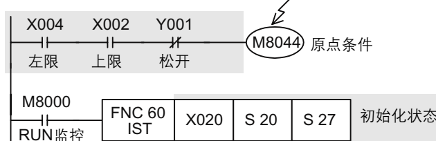
梯形图块
