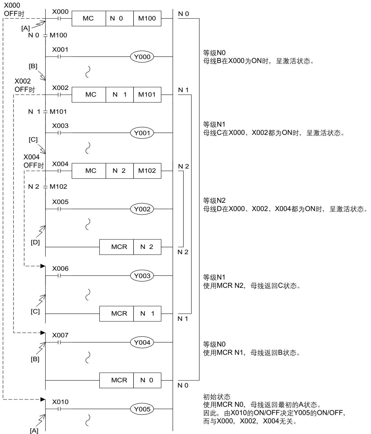
梯形图程序
