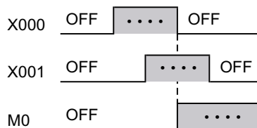
时序图
