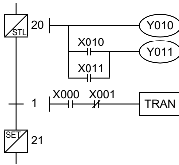
《SFC程序》
