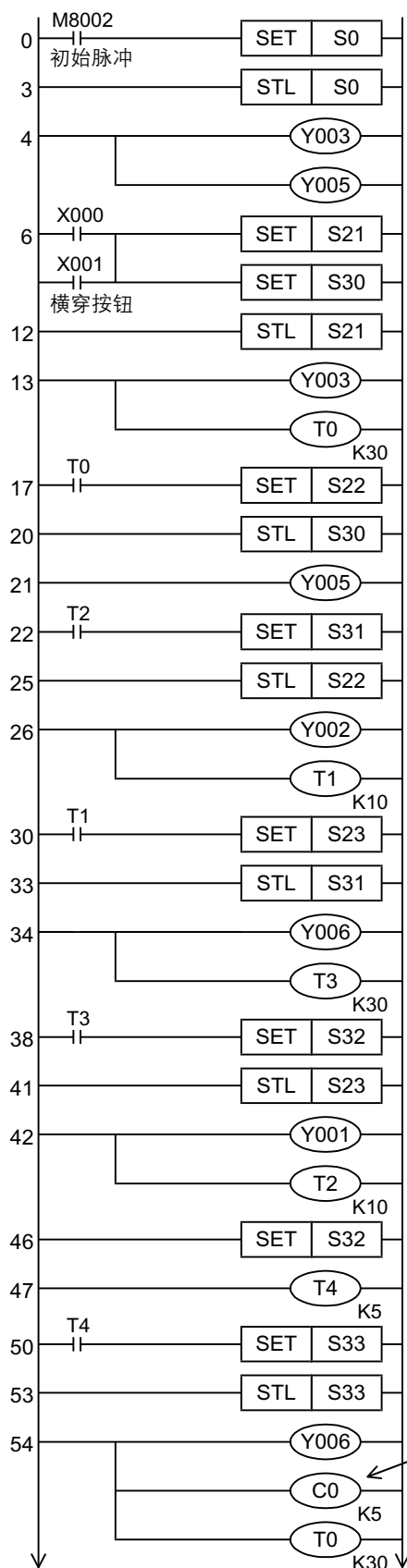
《步进梯形图》
