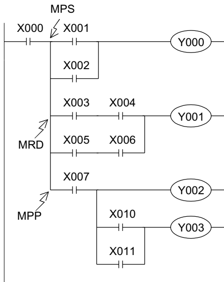
梯形图程序
