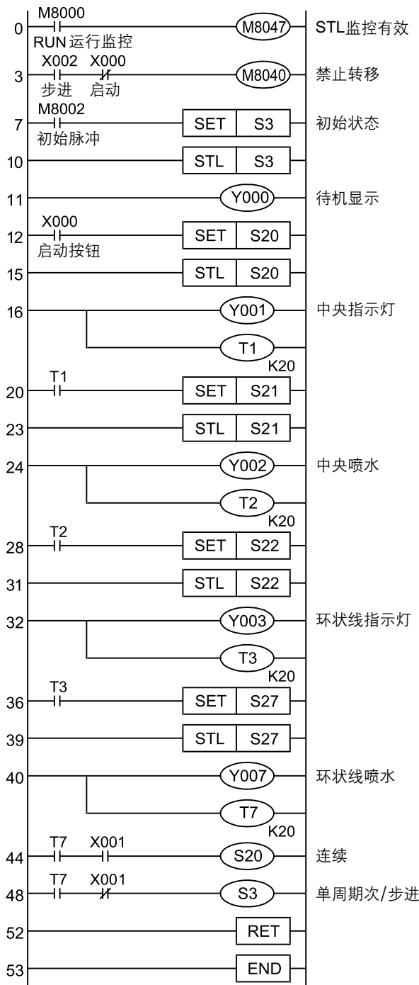
《步进梯形图》
