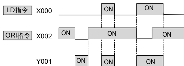
时序图
