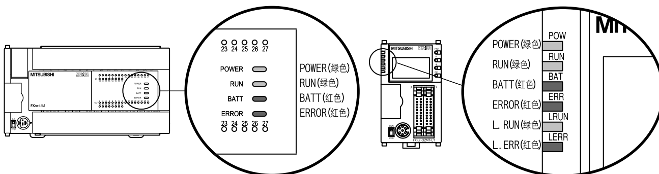
FX3U可编程控制器
