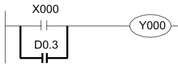
梯形图程序
