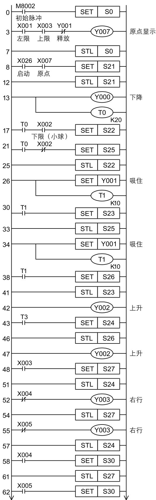
《步进梯形图》
