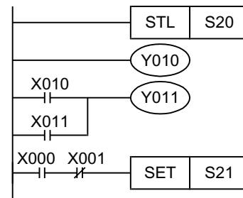
《步进梯形图》
