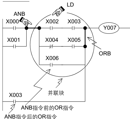
梯形图程序
