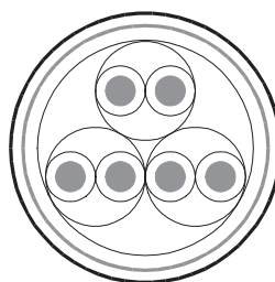
3对电缆的结构图实例
