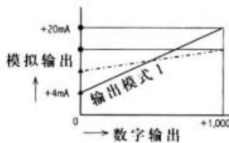
标准电流输出特性 (+4mA 到 +20mA)
