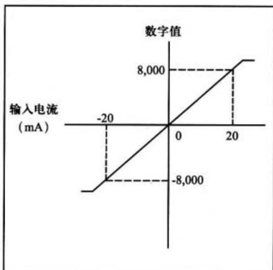
6. 电流输入，-20 到 20mA，40mA × 1/16,000
