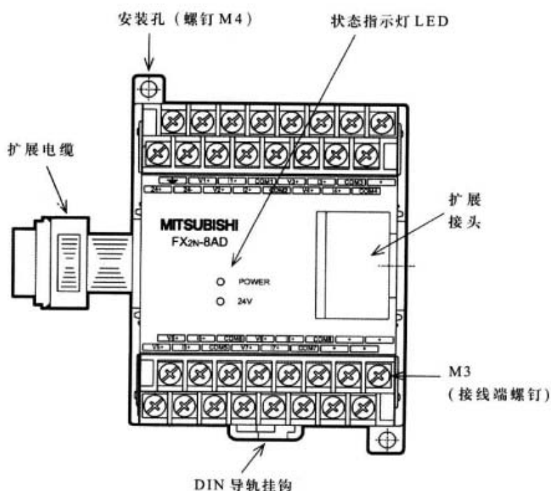
图 3.1: 部件名字
