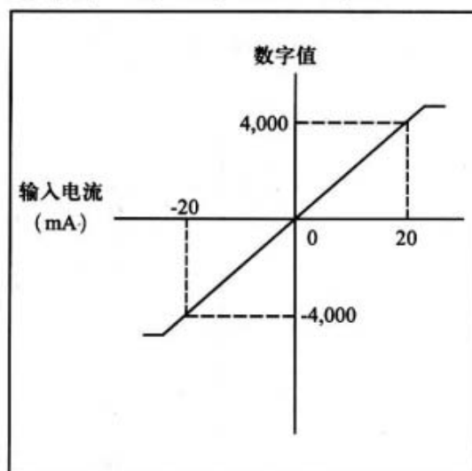
7. 电流输入，-20 到 20mA，40mA × 1/8,000
