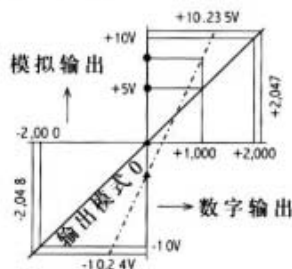
标准的电压输出特性
