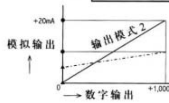
标准电流输出特性 (0mA-20mA)
