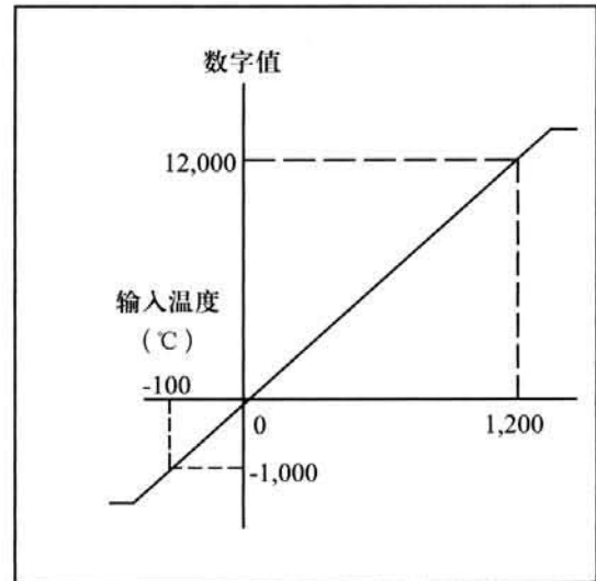
9. 热电偶输入，K 类，摄氏温度
