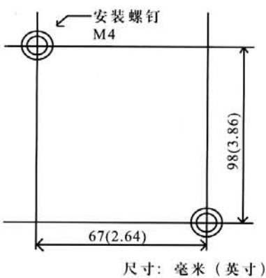
图 4.2: 直接安装
