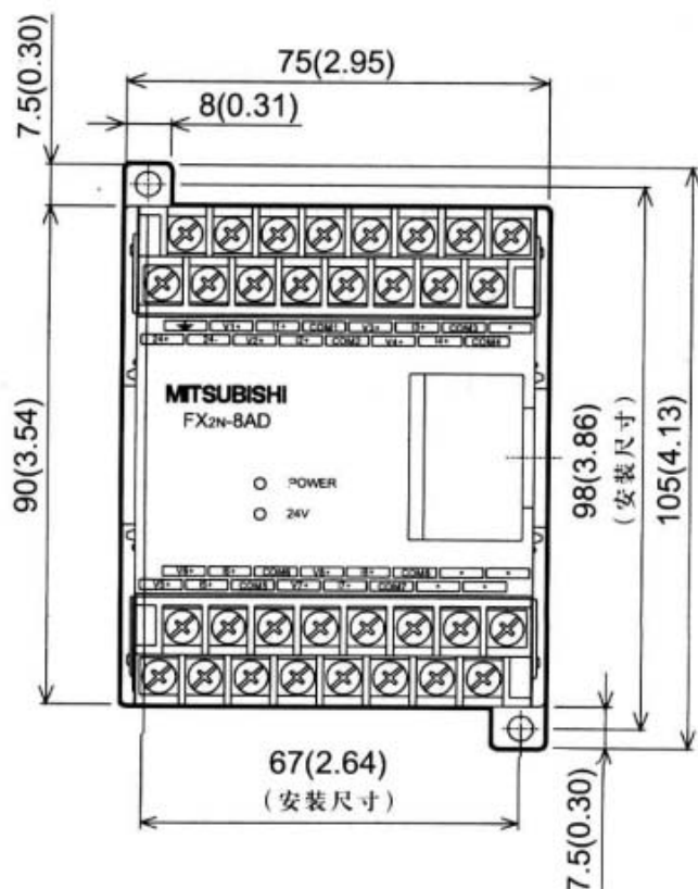
图 2.1: 外部尺寸
