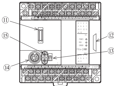
盖板打开时
