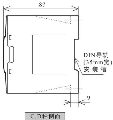
C,D种侧面
