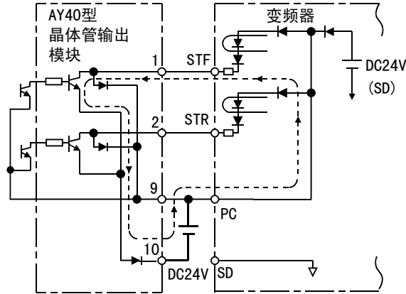
--- 电流的流动方向
