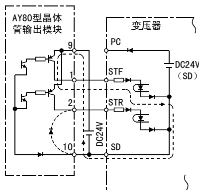
--- 电流的流动方向
