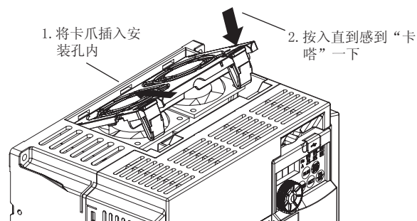
FR-E740-5.5K-CHT的示例
