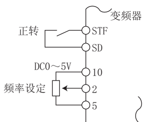
使用端子2（DC0~5V）时的布线例
