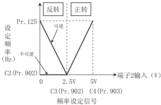
可逆运行示例
