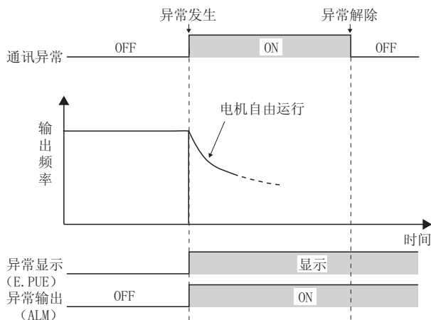
●Pr. 502 设定值 “2”
