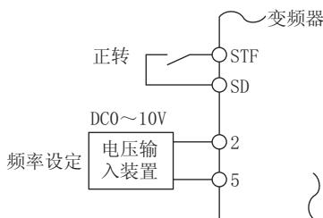
使用端子2（DC0~10V）时的布线例
