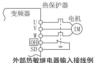
外部热敏继电器输入接线例
