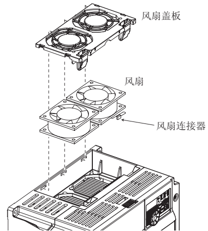
FR-D740-7.5K-CHT的示例
