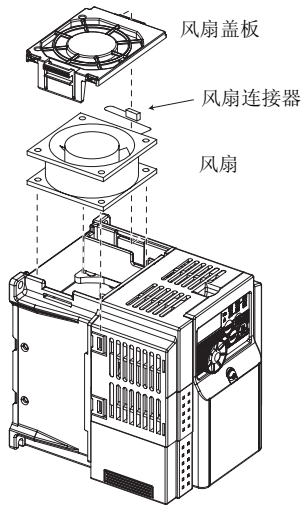
FR-D740-1.5K-CHT的示例
