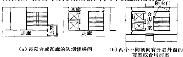
图14 带阳台或凹廊的防烟楼梯间及两个不同朝向有开启外窗的前室或合用前室
