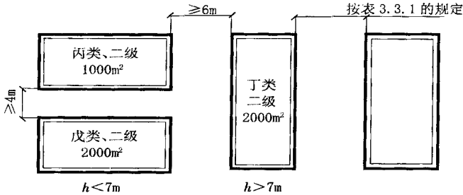
图 4 成组厂房布置示意图
