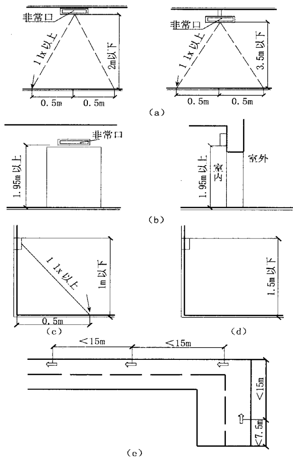
图 18 应急照明和疏散诱导灯设置位置(日本规范规定)
