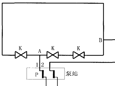
图 13 消防水泵房出水管与环状管道连接示意图
