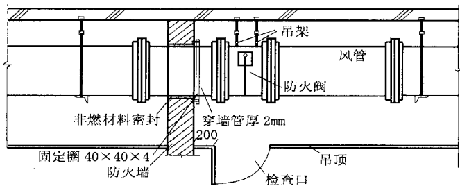
图 17 防火阀检修口设置示意图
