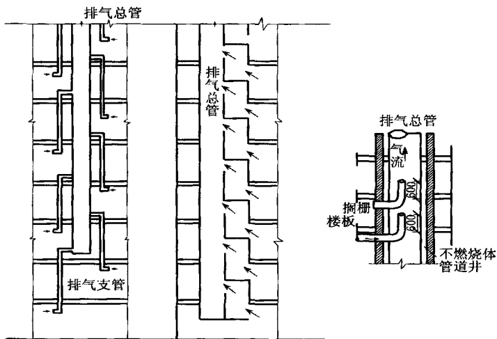
图 15 排气管防止回流示意图
