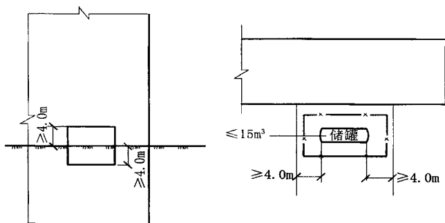
图 2 油罐面 4.0m 范围外墙设防火墙示意图
