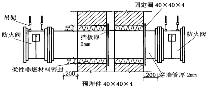
图 16 变形缝处的防火阀
