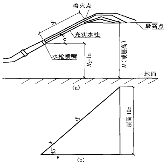
图 12 充实水柱长度计算
