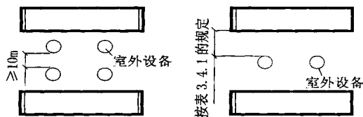
图 1 有室外设备时的防火间距
