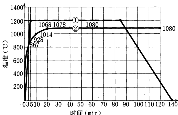
图 A.0.1 RABT 标准升温曲线
