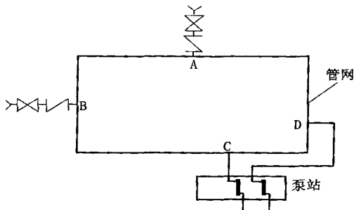
图 9 水泵接合器的布置要求
