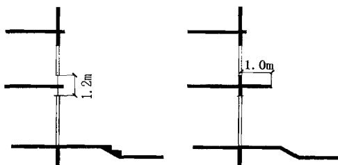
图7 防火挑檐示意图
