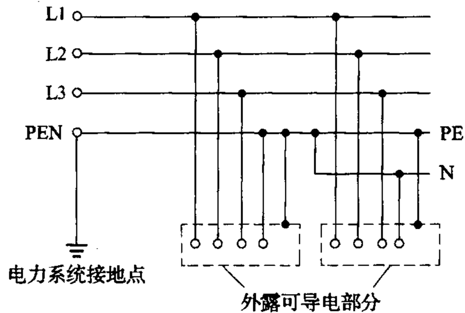
图 6 TN-C-S 系统
