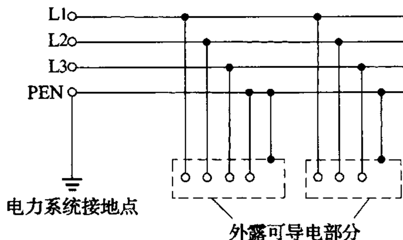
图 5 TN-C 系统
