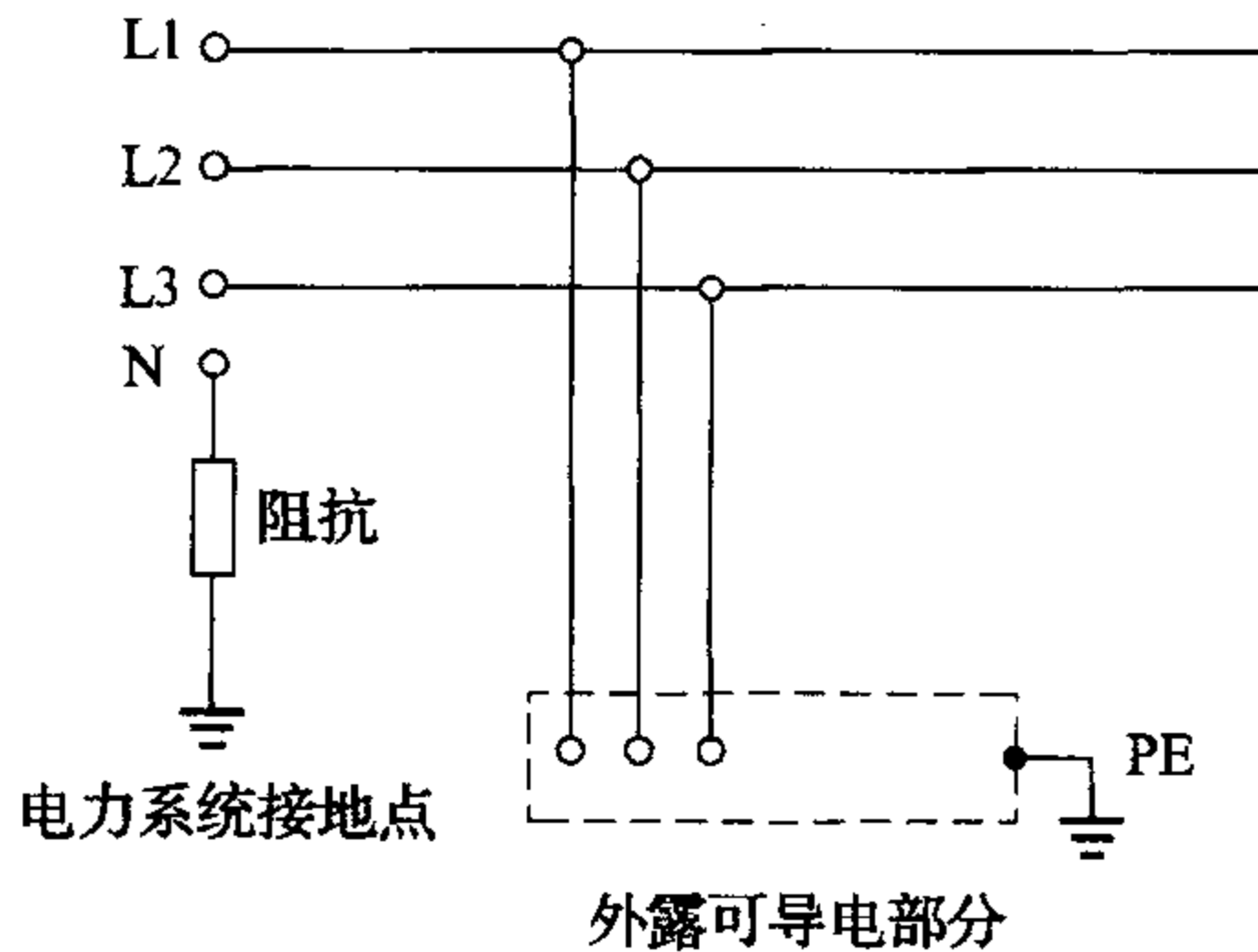
图 9 IT 系统
