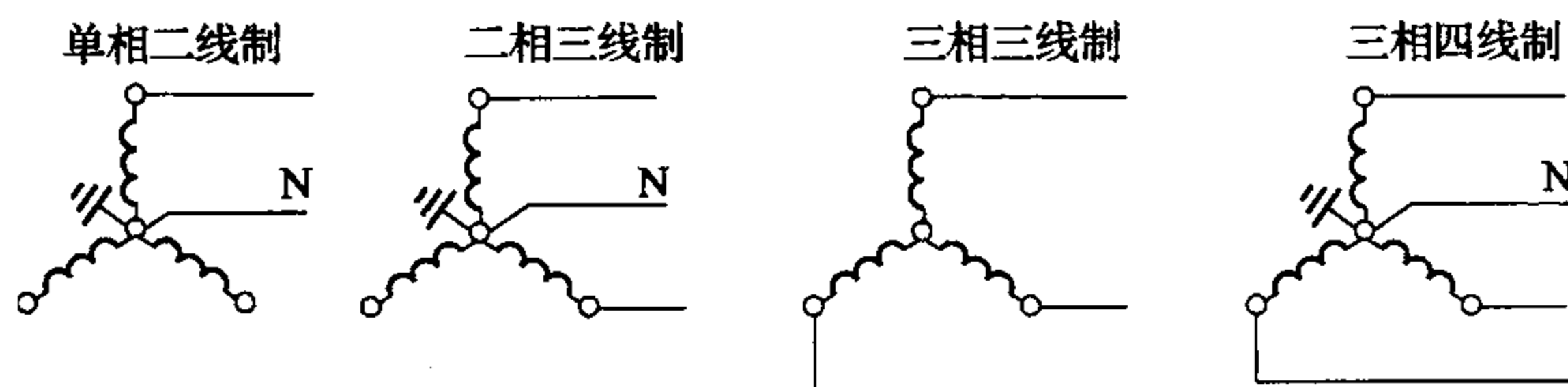
图 4 交流系统带电导体类型
