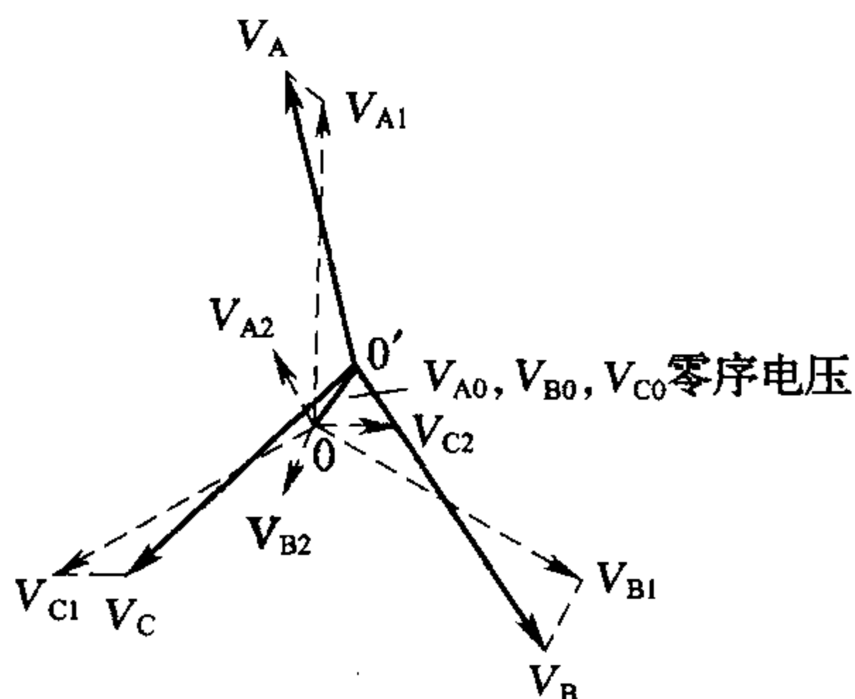
图 3 不对称电压向量图
