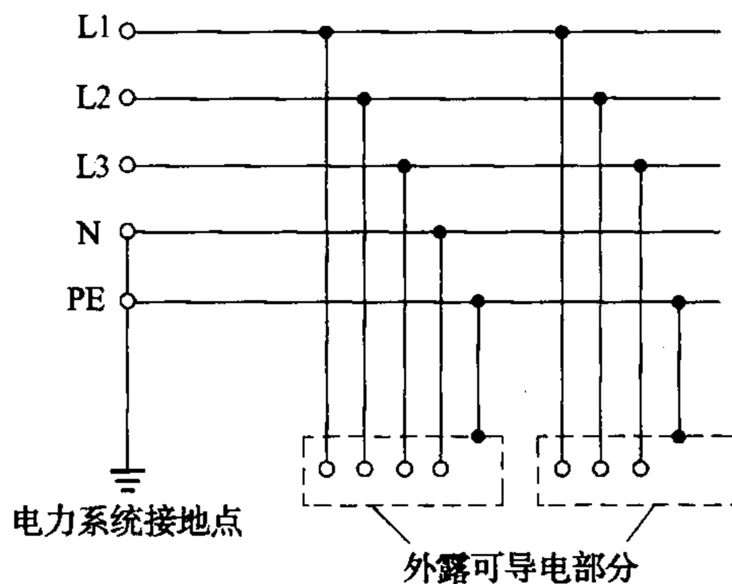
图 7 TN-S 系统
