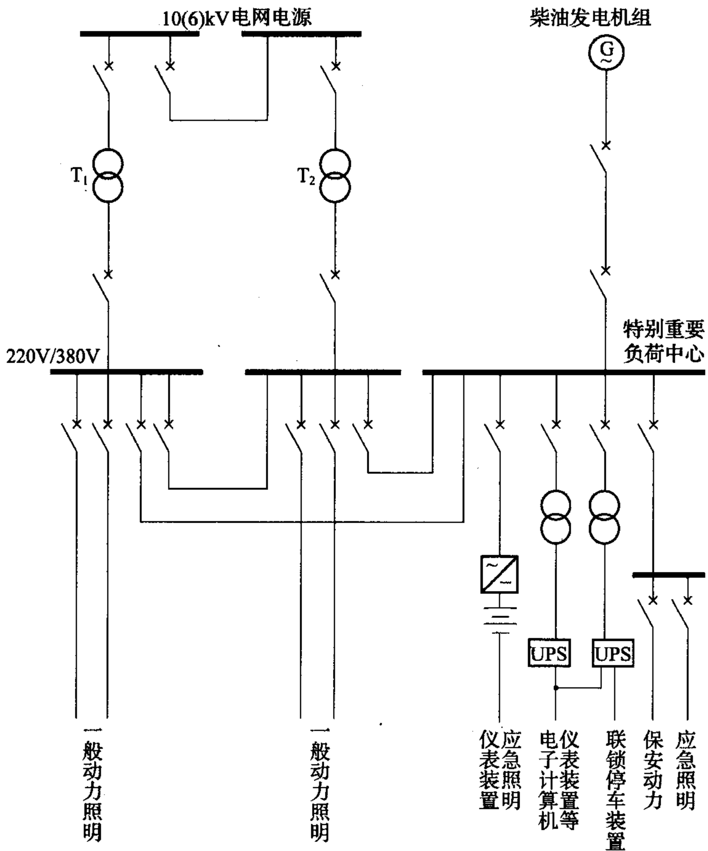
图 1 应急电源接线示例
