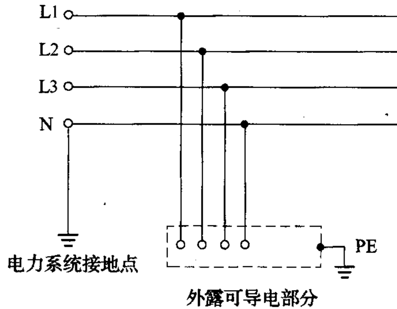
图 8 TT 系统
