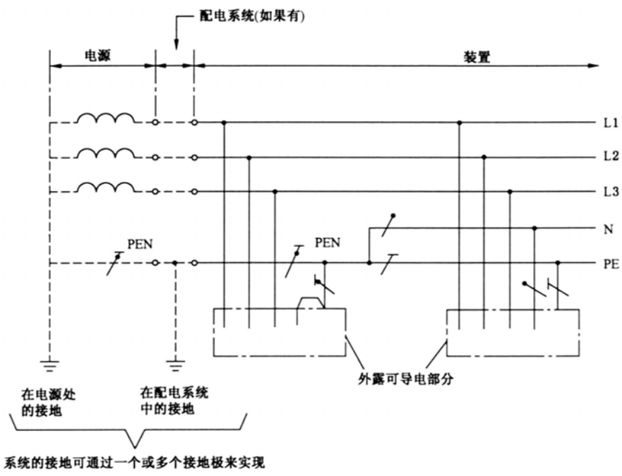
图 7.1.1-4 在装置非受电点的某处将 PEN 分离成 PE 和 N 的 3 相 4 线制的 TN-C-S 系统
