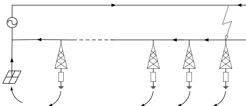
图 B.0.2-2 站外接地故障示意
