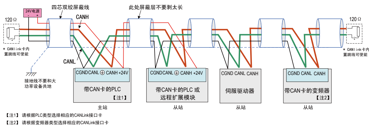
多台设备组网连接示意图
