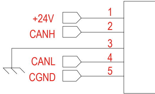
CANLink 接口引脚定义
