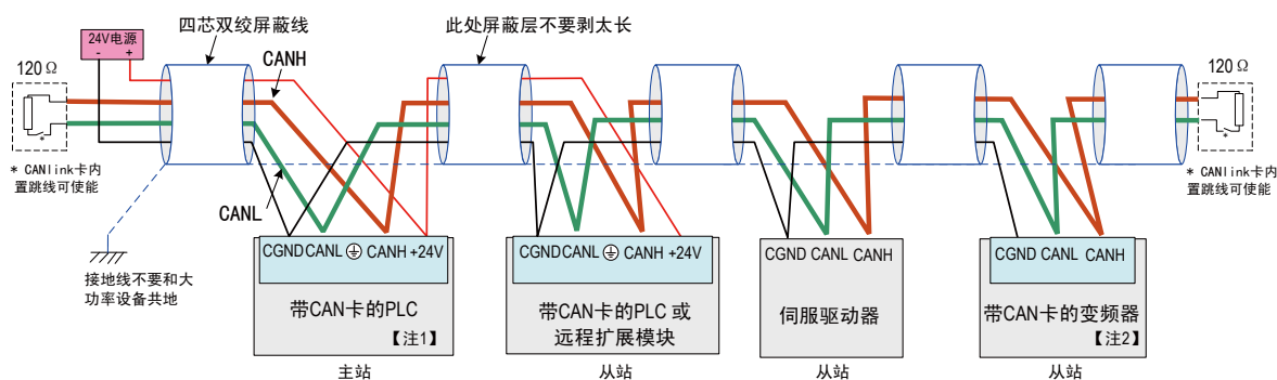
正确的 CANlink 网络接线
