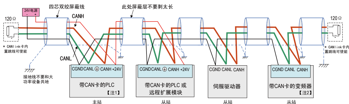
接线错误 -- 屏蔽层接地
