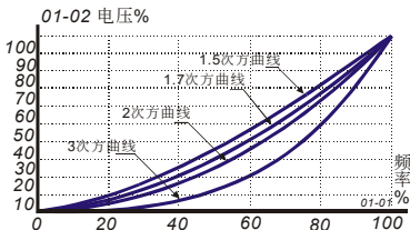
V/F 次方曲线图
