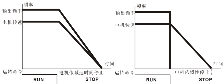
减速停止与自由运转停止
