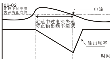
定速中过电流失速防止功能
