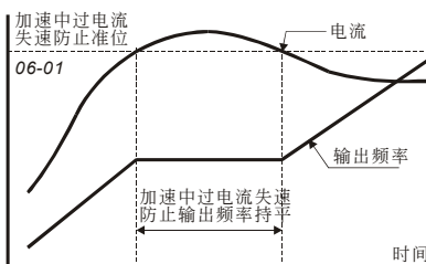
加速中过电流失速防止功能
