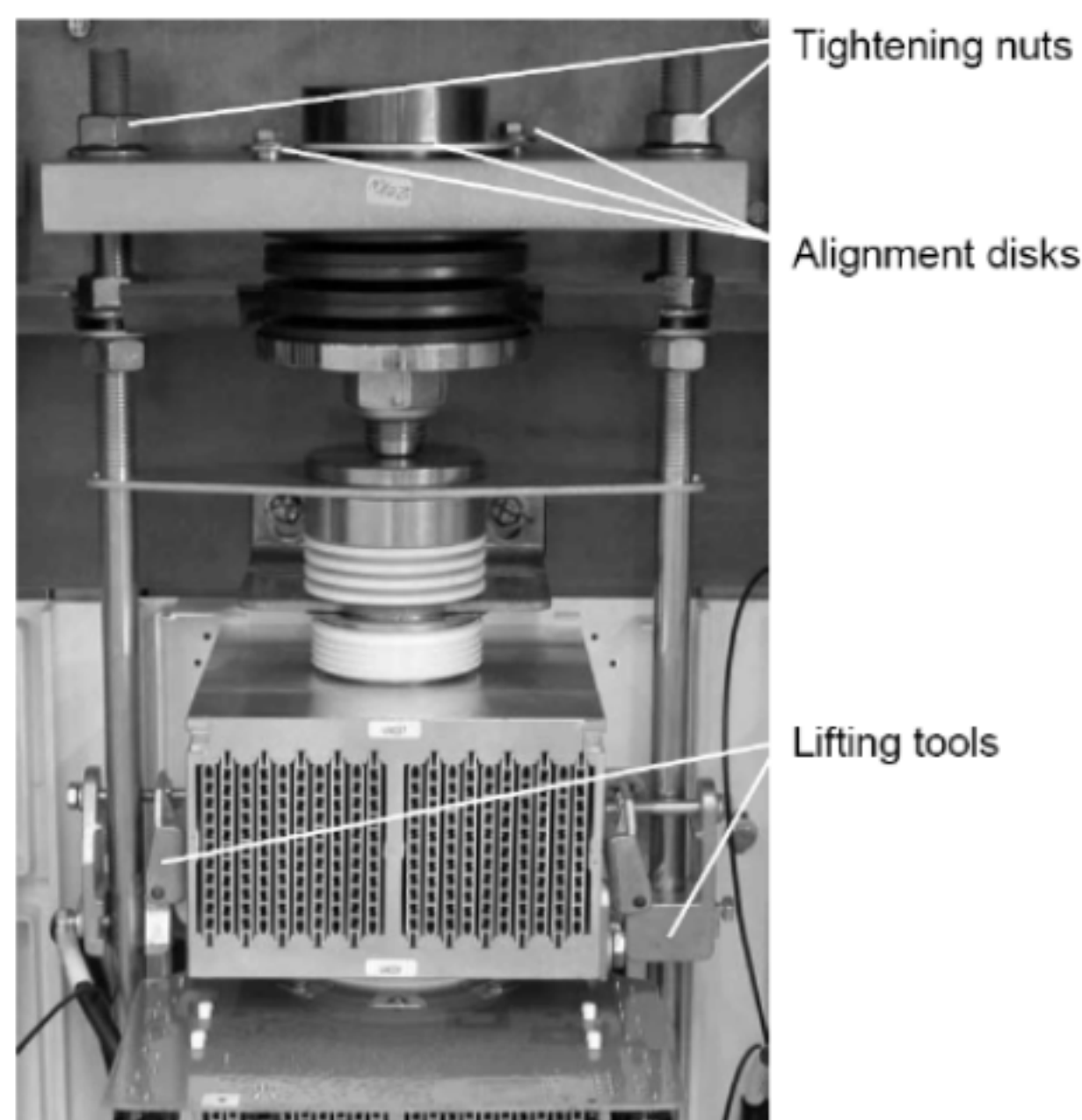
图5.1 相模块固定装置和提升工具
