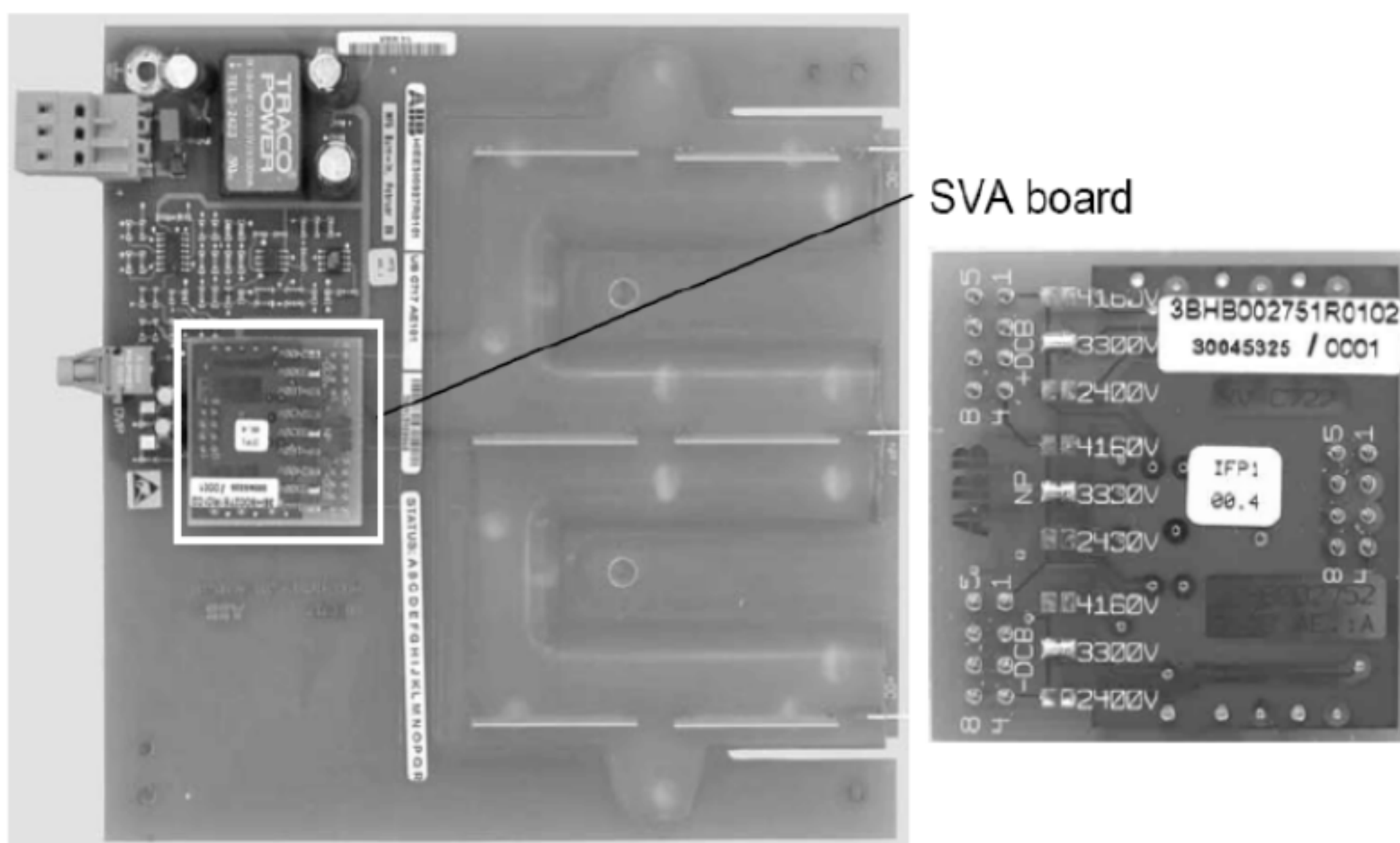
图6.9 电压侦测板和整流监控器
