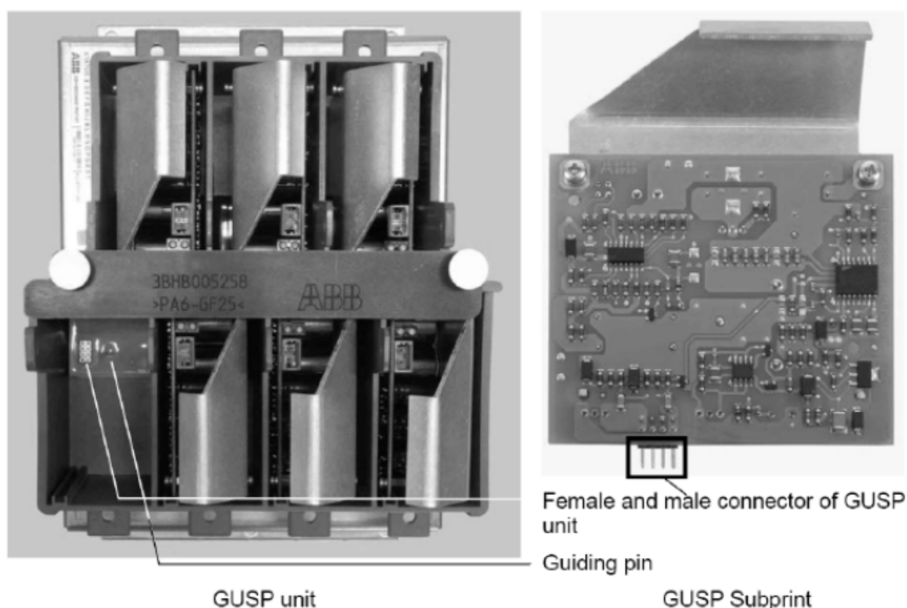
图 6.15 GUSP 单元和 GUSP 子板
