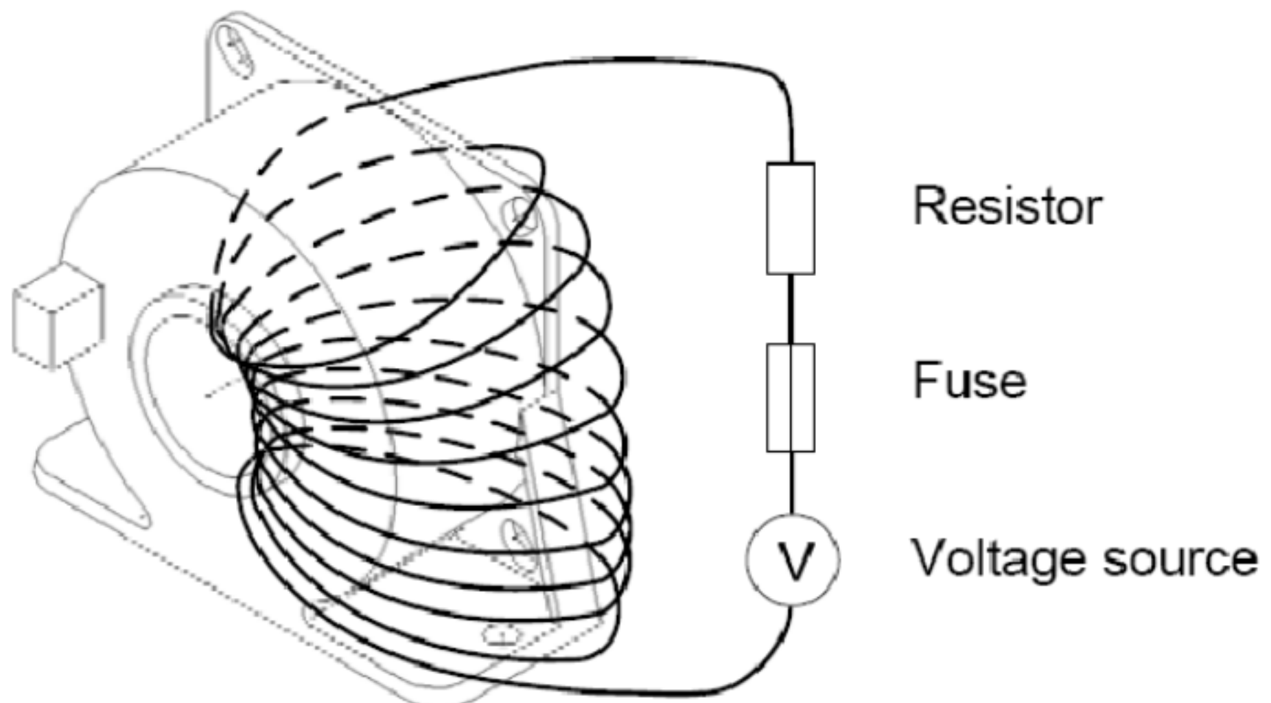
图4.1 测量电流互感器
