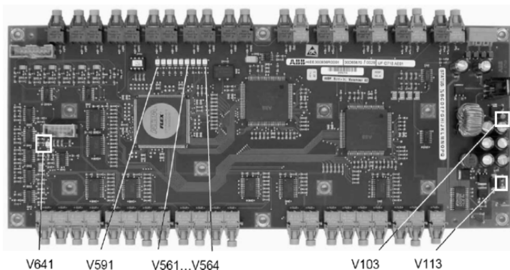
图7.2 INT板
