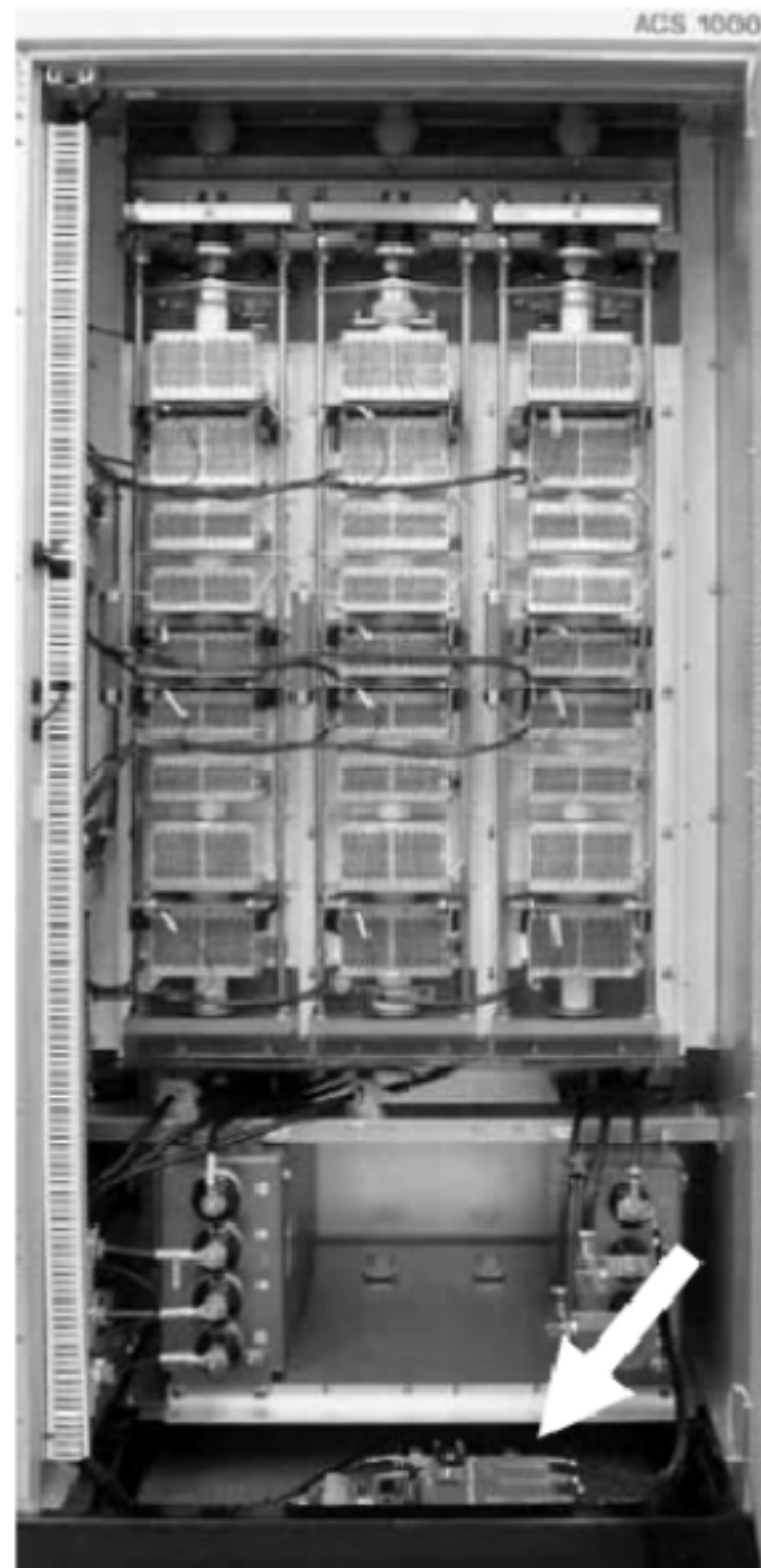
图6.14 ADCVI板在ACS1000i中位置
