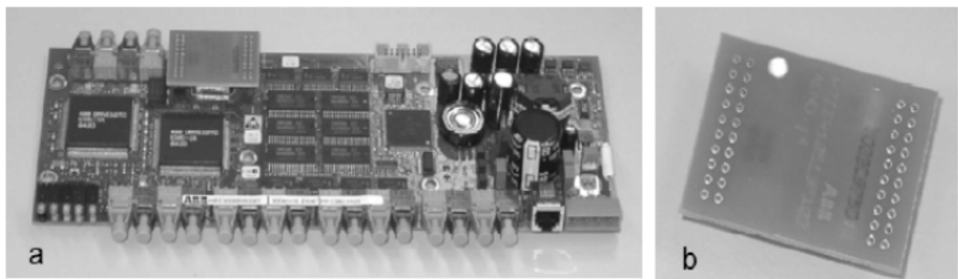
图6.3 AMC板和闪存PCB板
