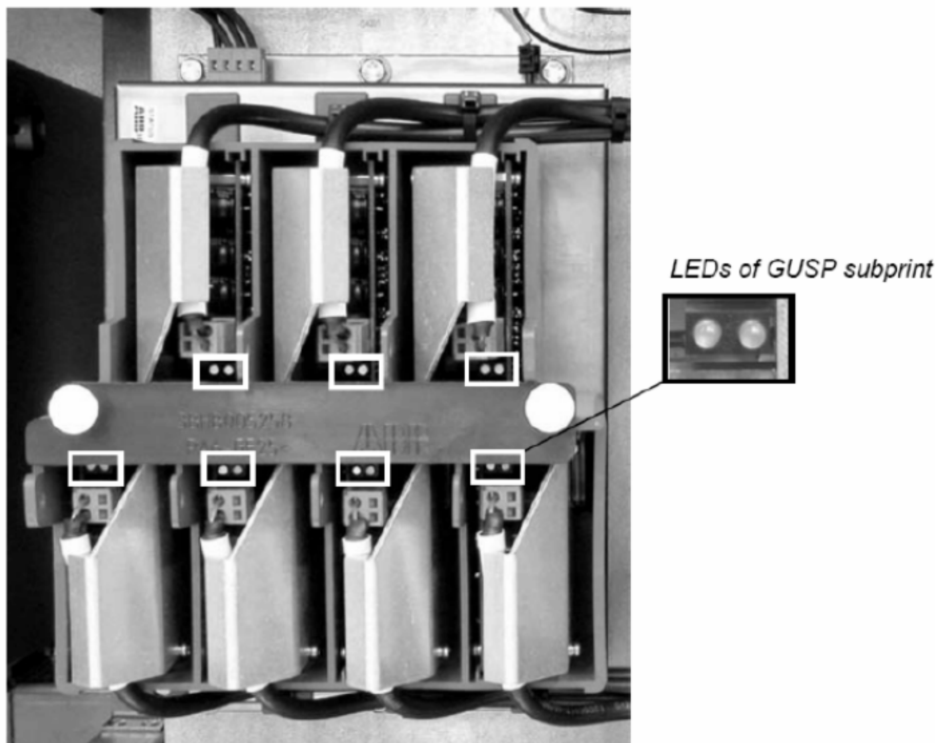
图7.3 GUSP单元
