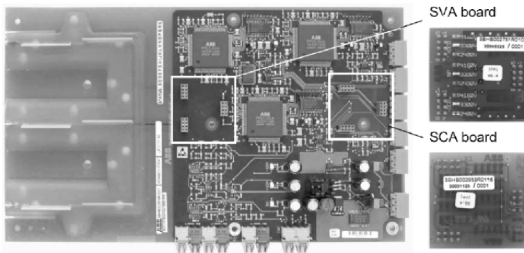
图6.12 ADCVI板
