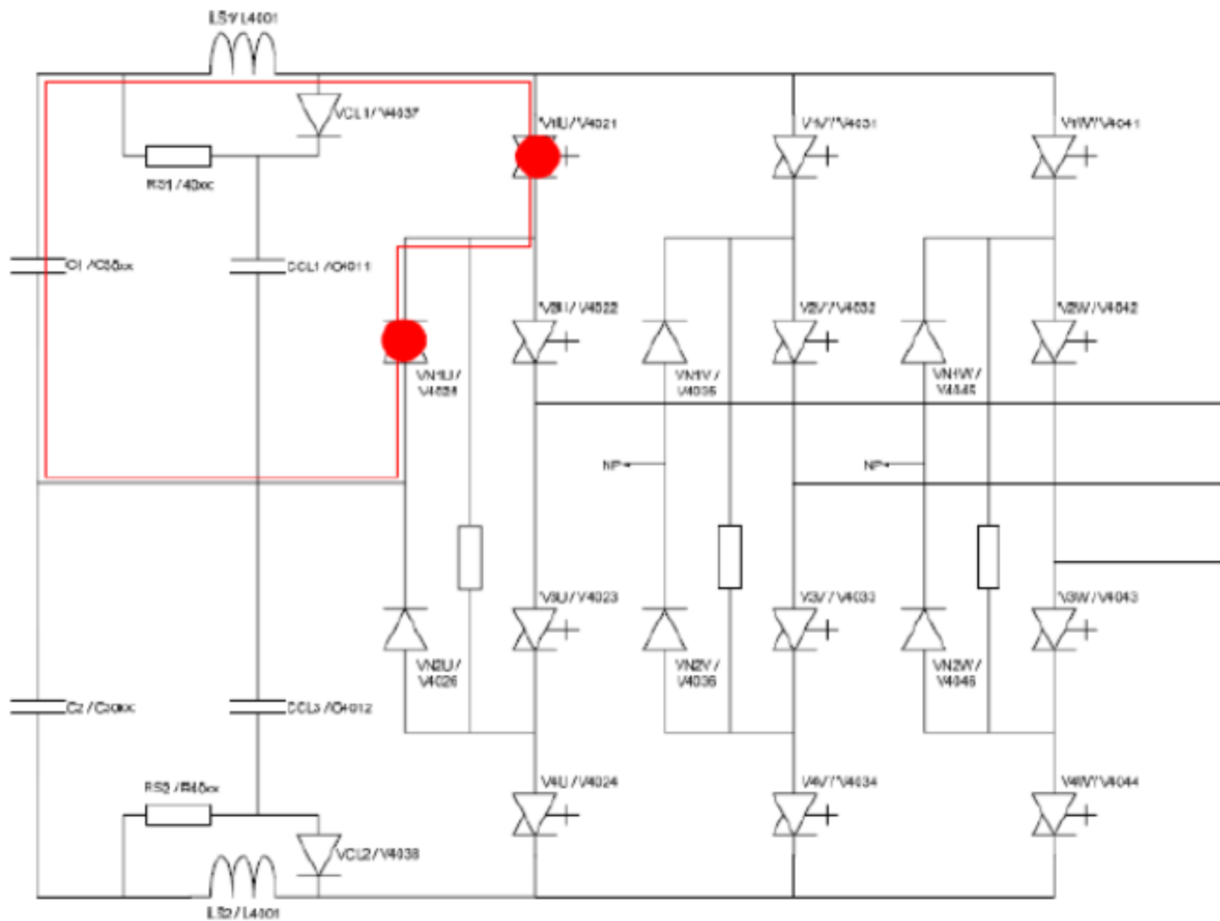
图 2. 1 典型的正极故障
