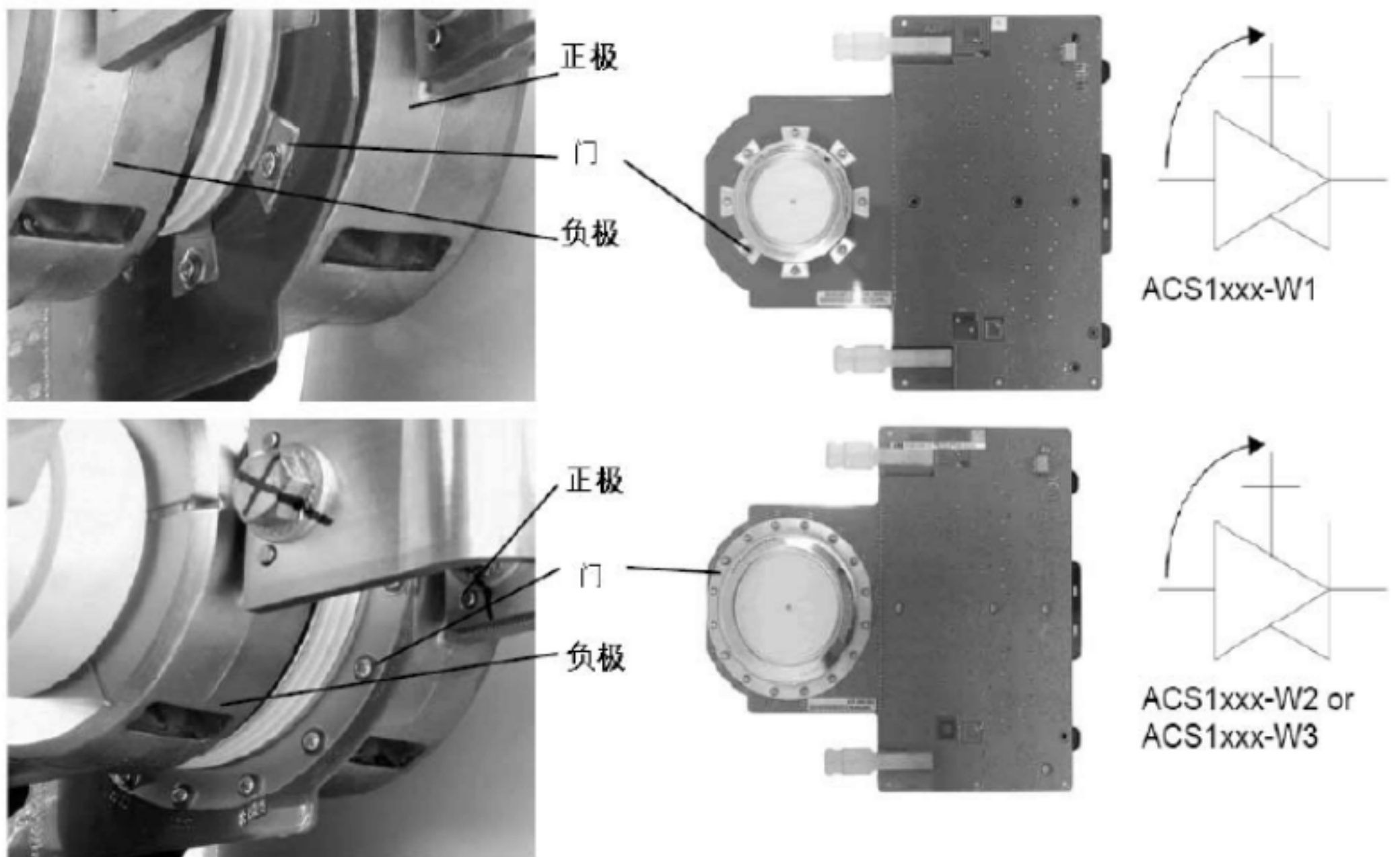
图 3.2 测试水冷型变频器内 IGCT
