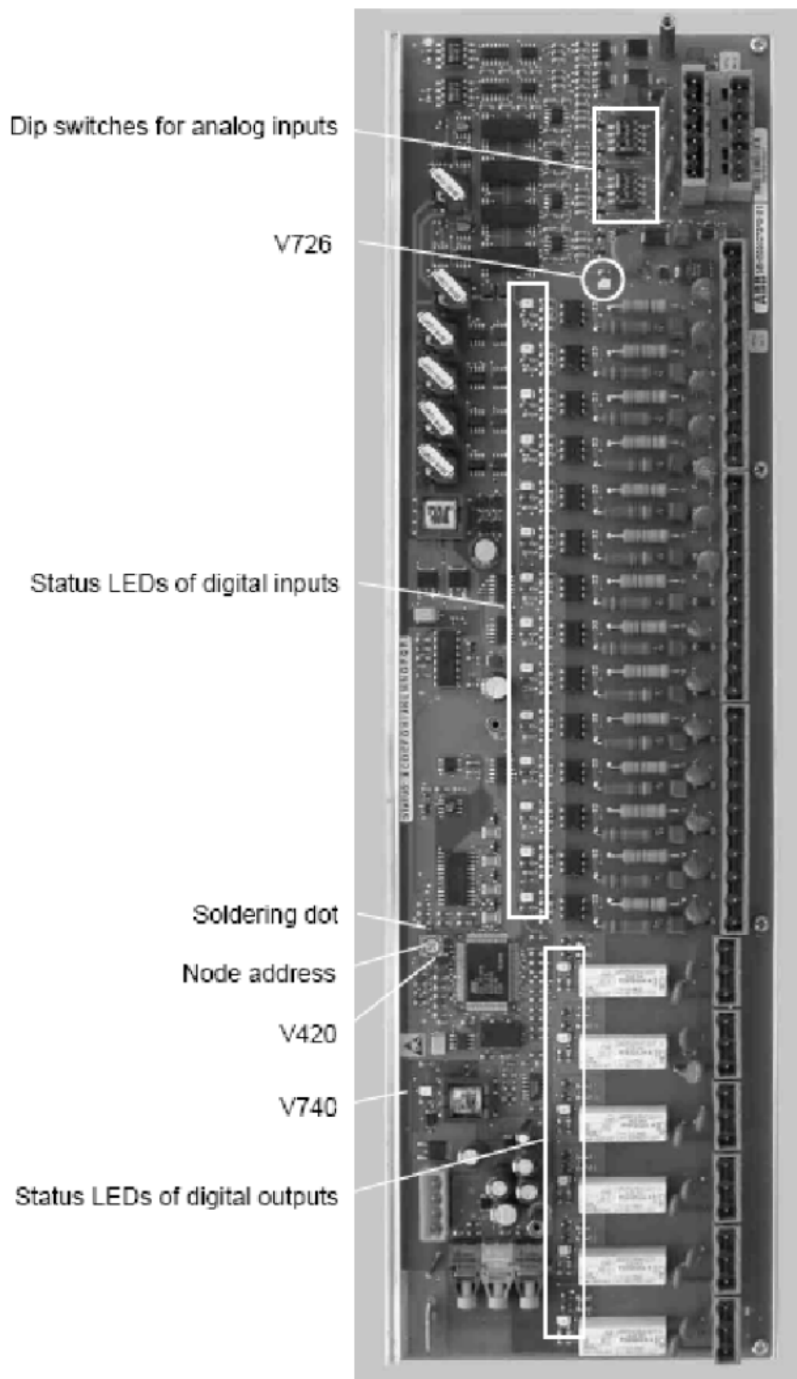
图7.4 IOEC板
