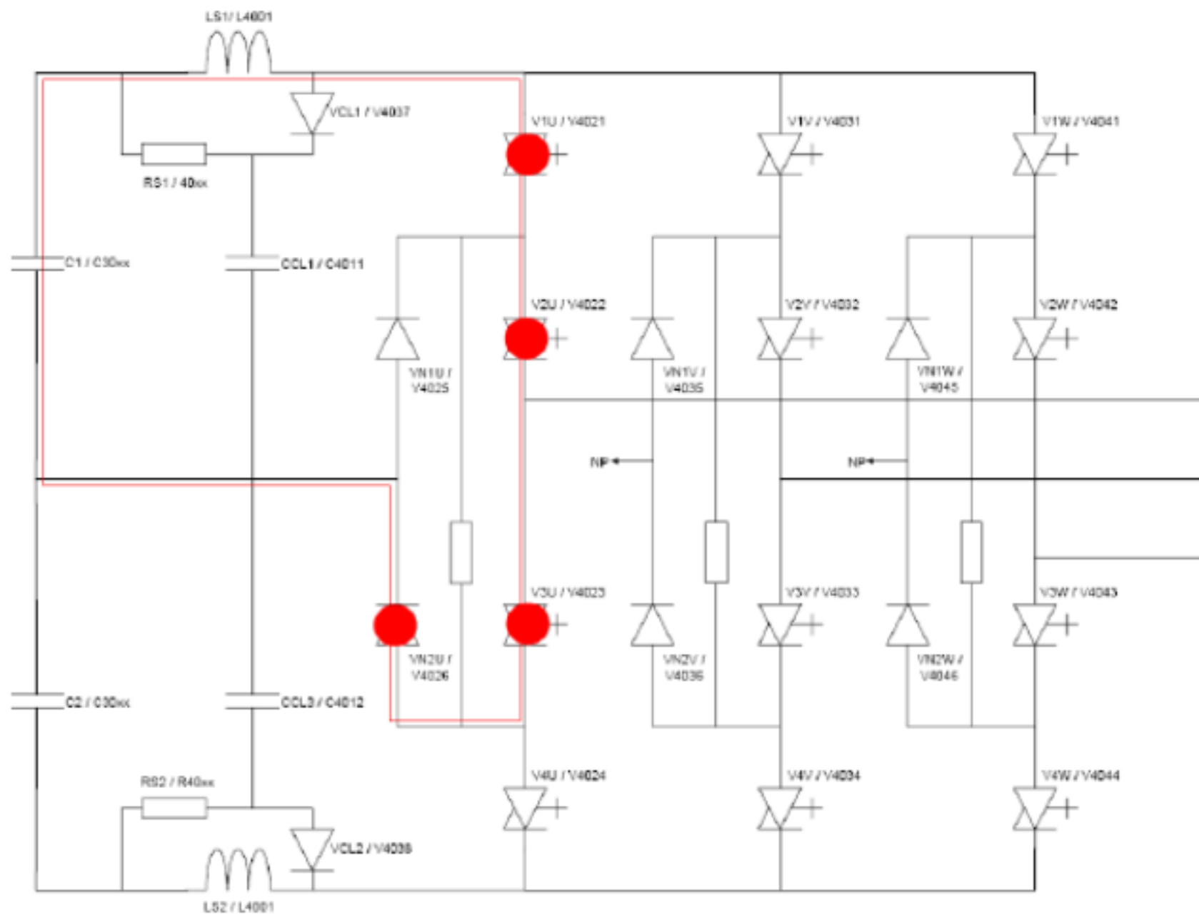
图 2. 3 典型的正极故障
