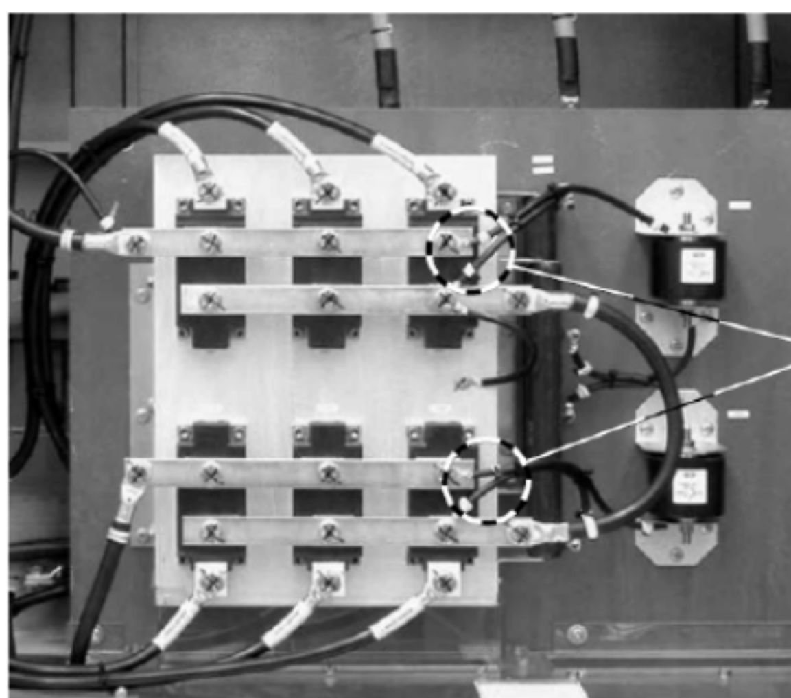
图5.6 ACS1000i中的整流二极管
