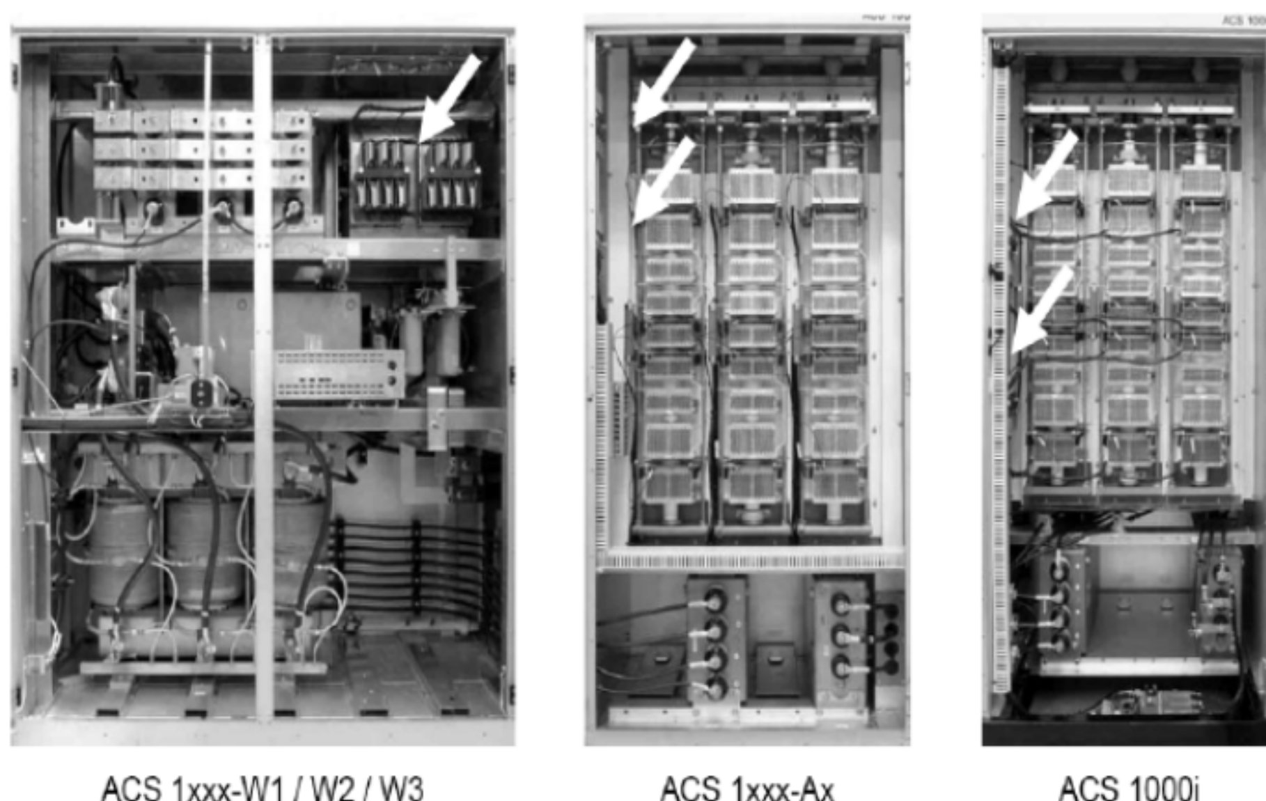
图 6.16 GUSP 位置图
