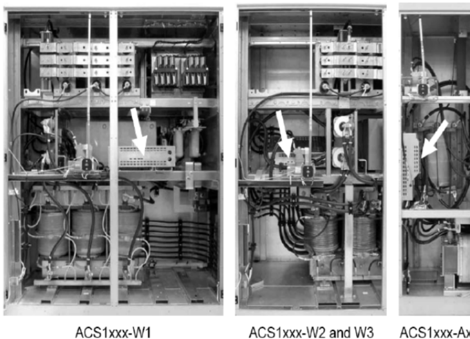
图6.10 标准水冷型和风冷型ACS1000变频器中OVVP板的位置分布 电压侦测板在ACS1000i变频器中安装在逆变单元中（如6.11整体图）。整流监控器安装在逆变单元的中部靠近柜体壁的地方（如6.11放大图）。
