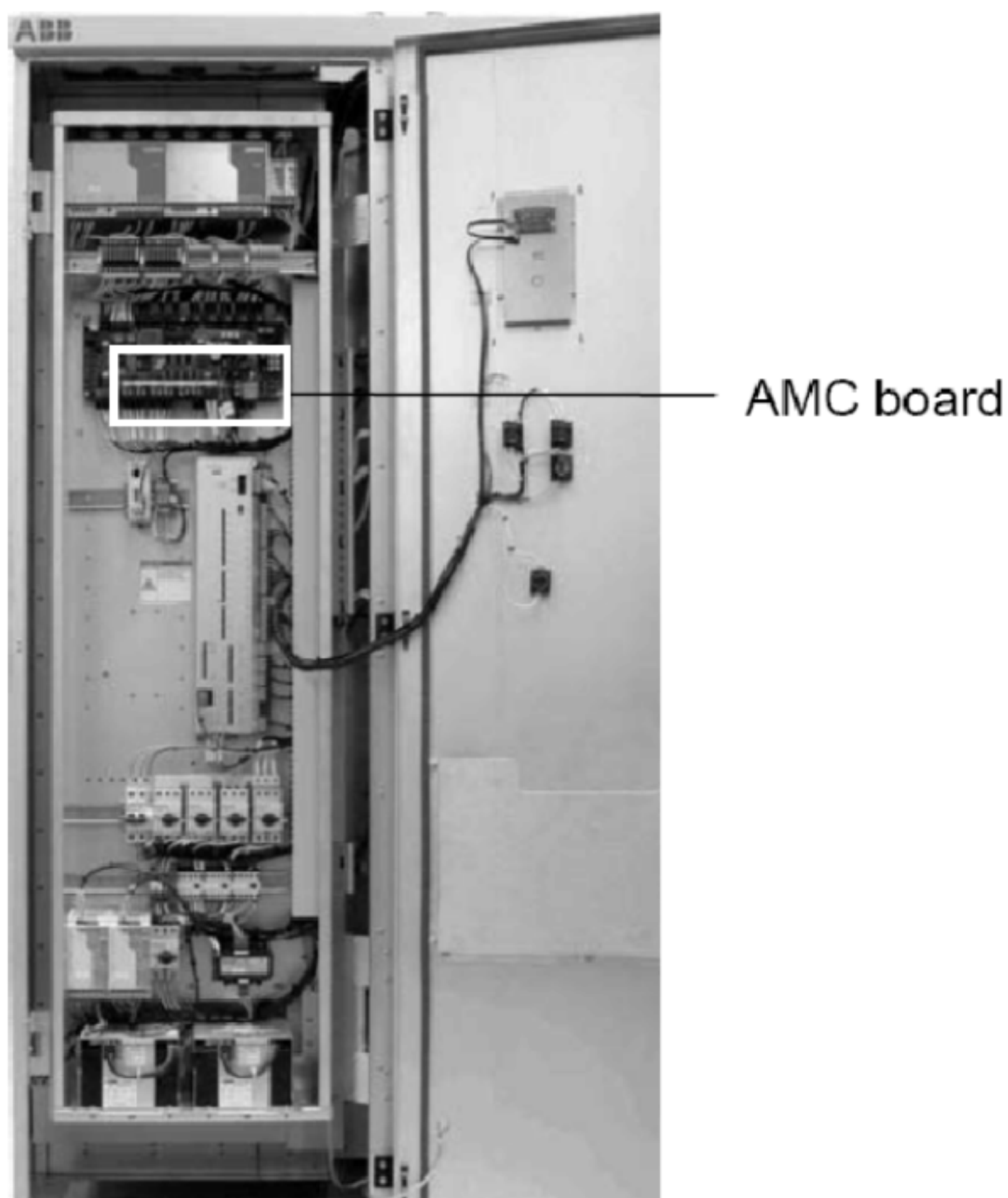
图6.2 AMC板的安装位置
