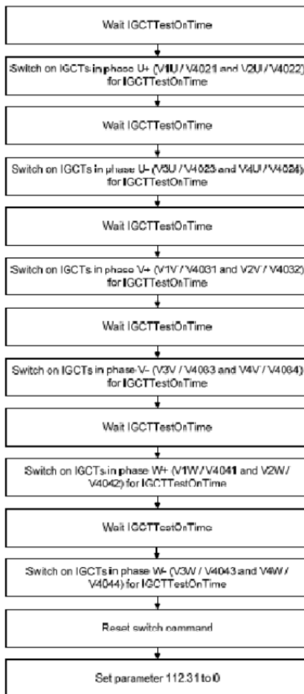
图 3.4 IGCT 测试次序
