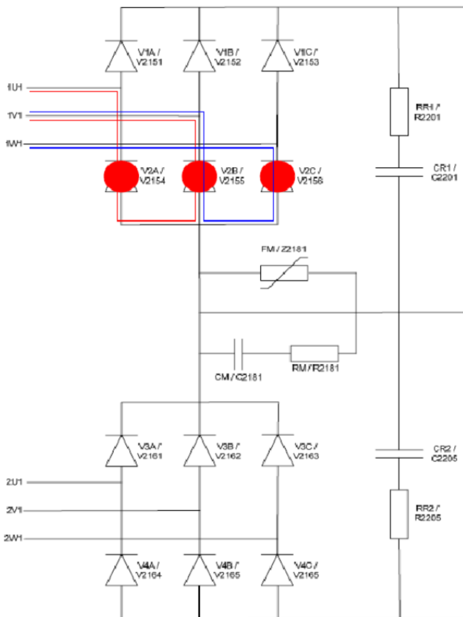
图 2.5 整流故障中一例
