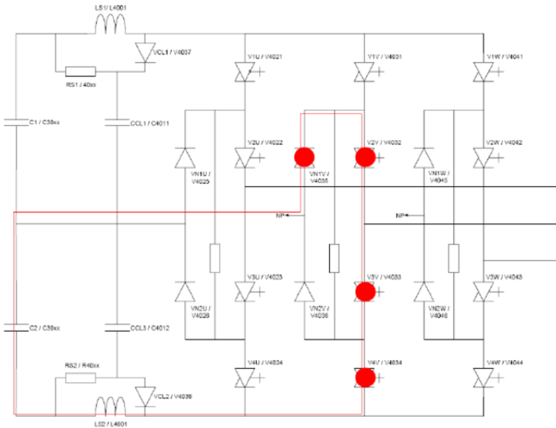
图 2. 2 典型的负极故障
