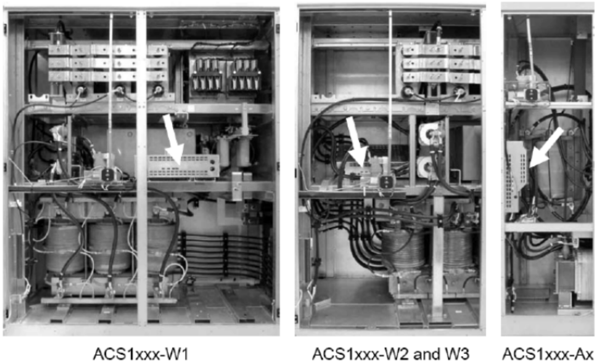
图6.13 ADCVI板在ACS1000中位置
