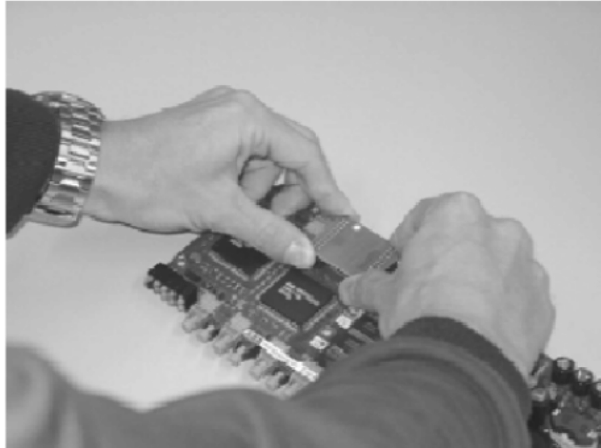
图6.6 插入新闪存PCB板
