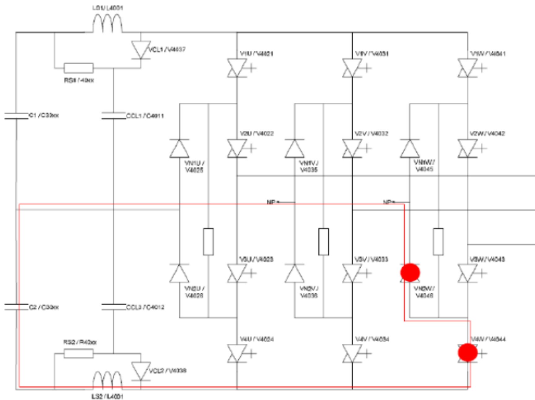
图 2. 2 典型的负极故障
