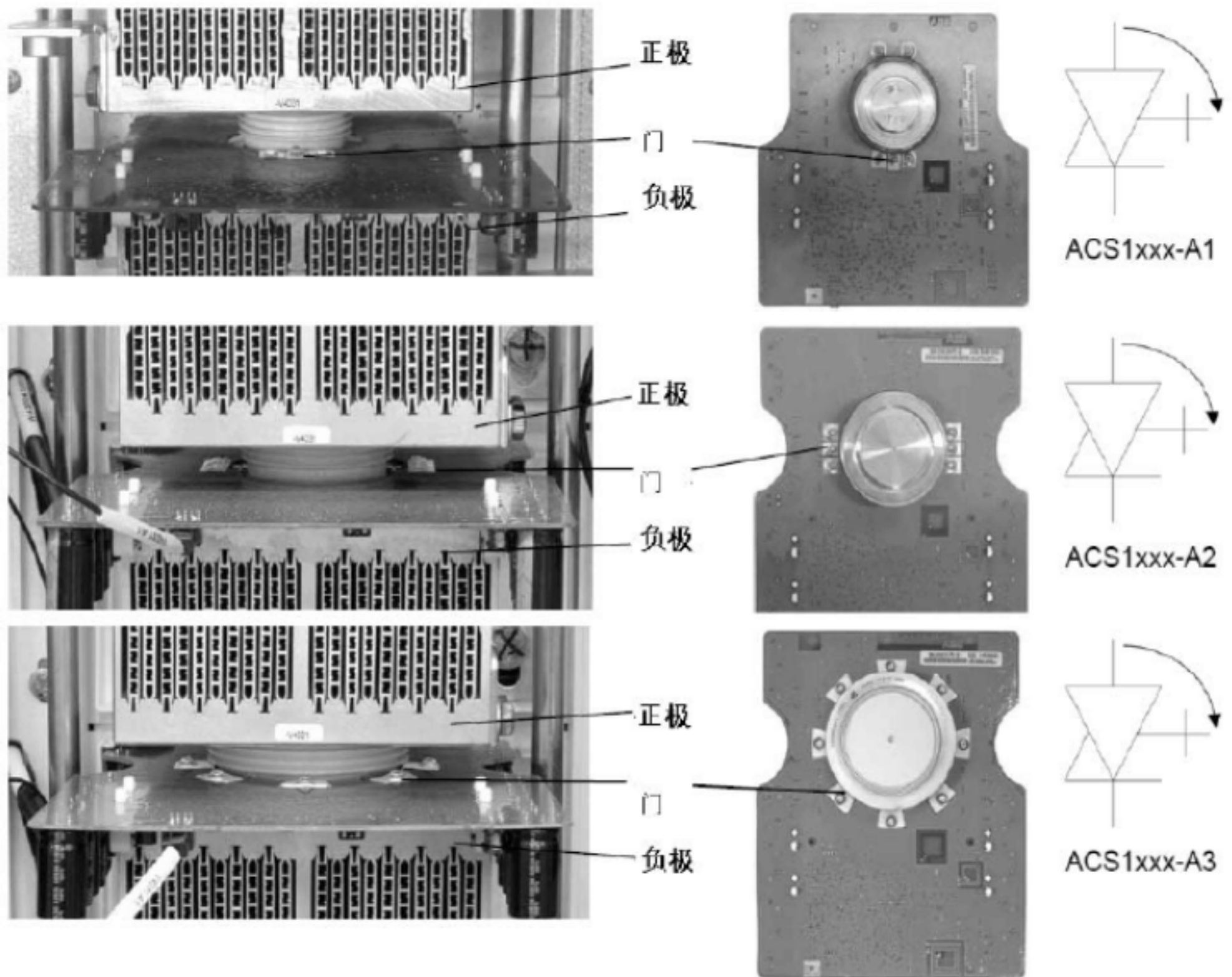
图 3.2 测试风冷型变频器内 IGCT
