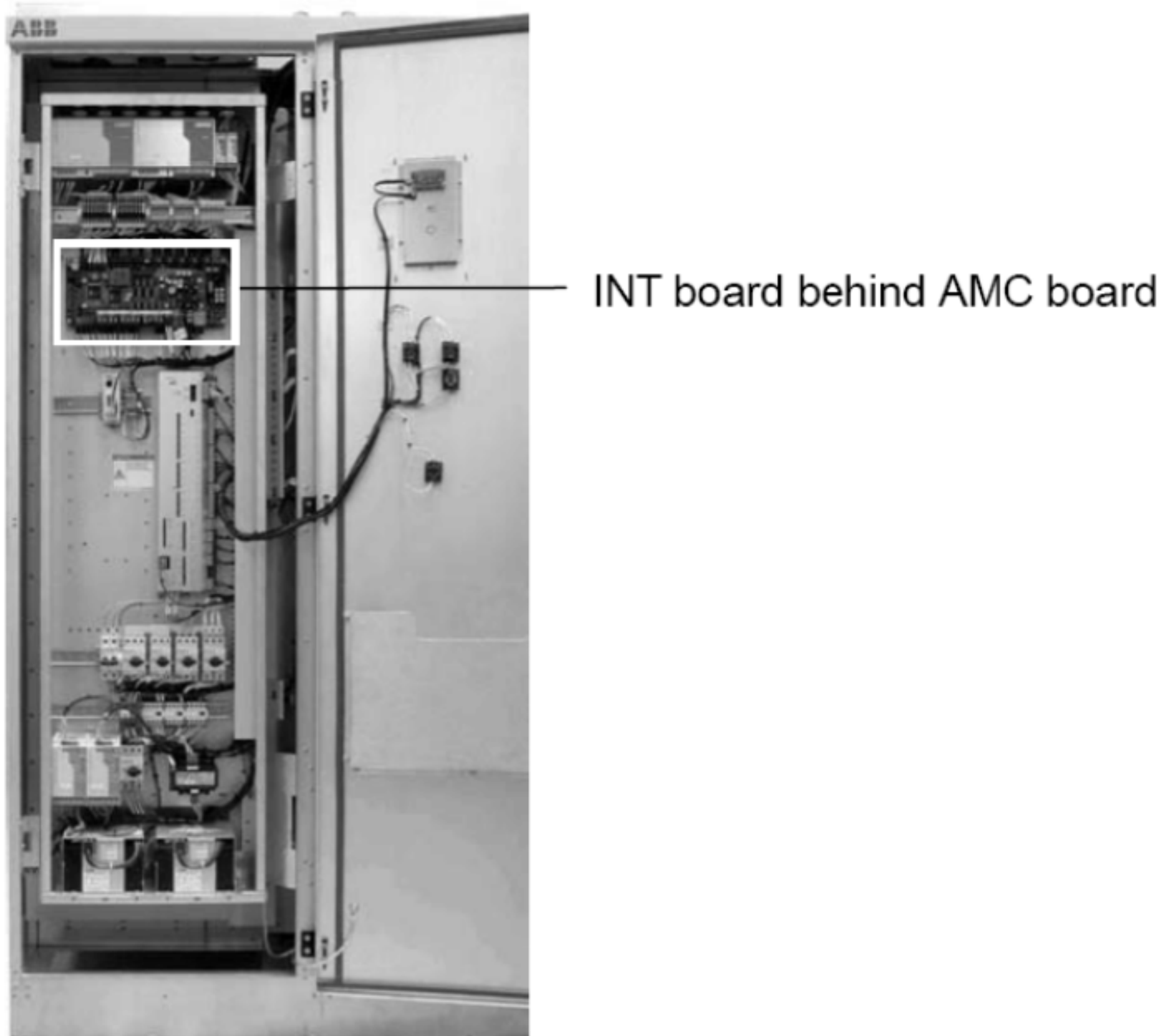
图6.8 INT板的分布
