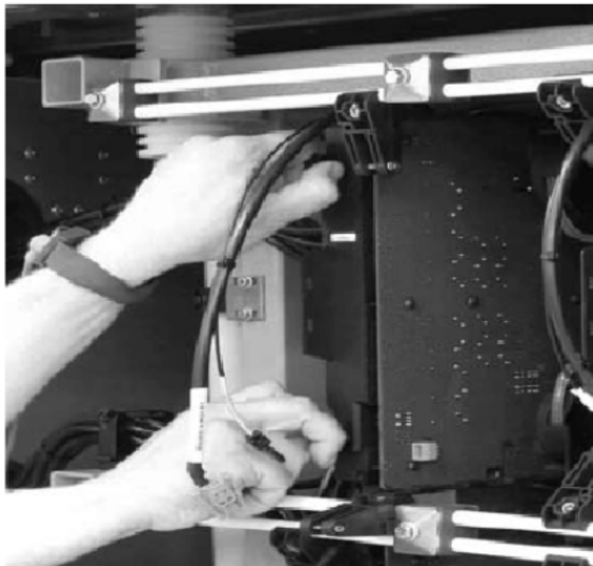
图5.5 取出IGCT
