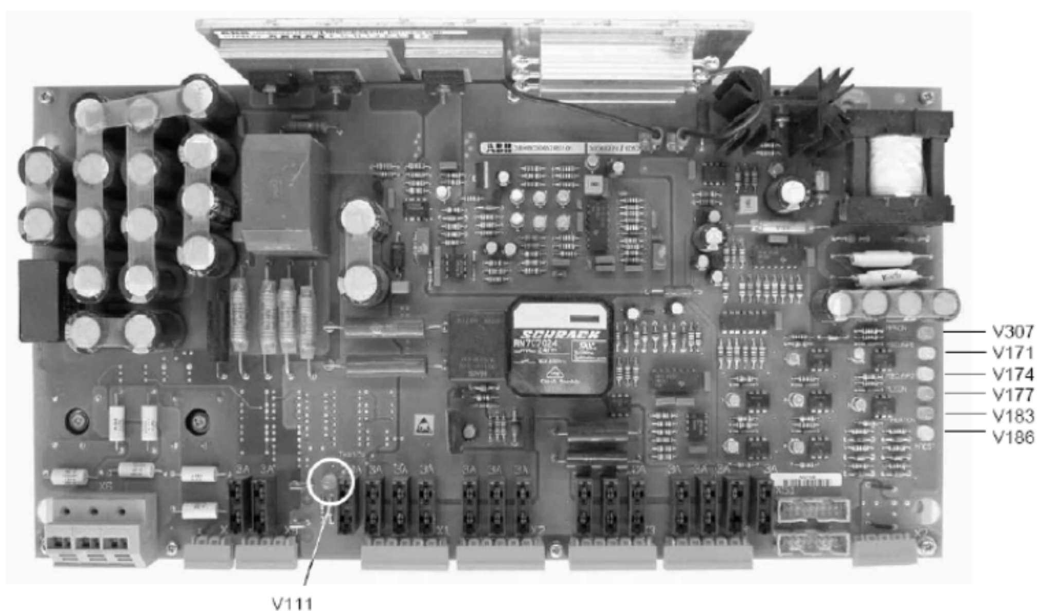
图7.1 EPS板
