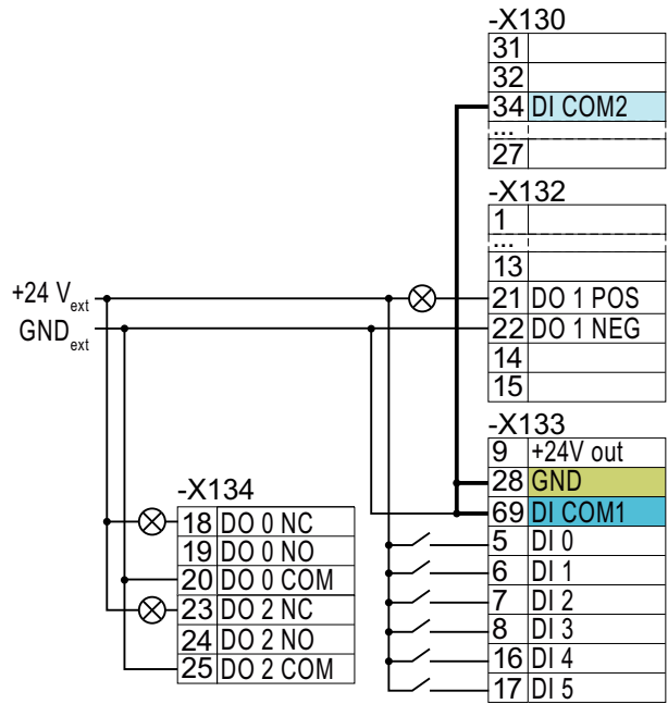
连接源型触点和外部电源
