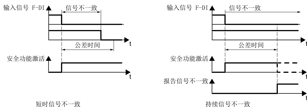
图 6-27 差异时间一致性监控
