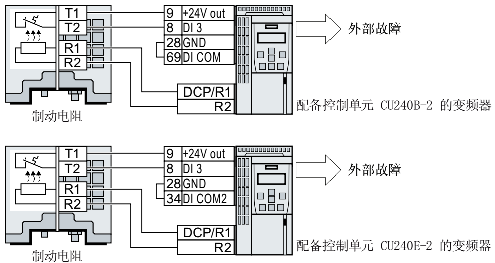
图 4-28 示例：通过控制单元的数字量输入 DI 3 进行制动电阻的温度监控
