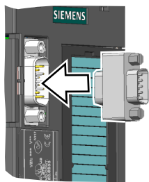
图 3-1 将 KnorrTec 适配器插入操作面板接口
