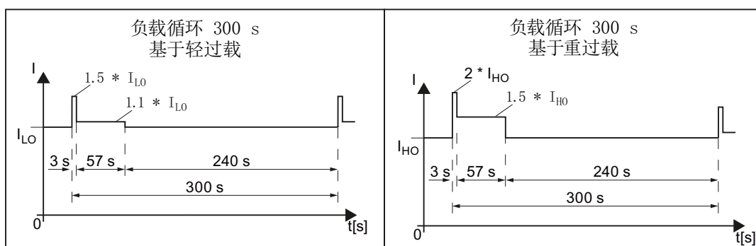
图 10-1 “轻过载”和“重过载”的负载循环
