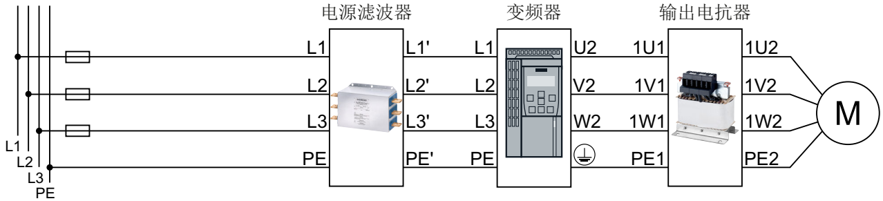
图 4-13 功率模块 PM230 的接线一览
