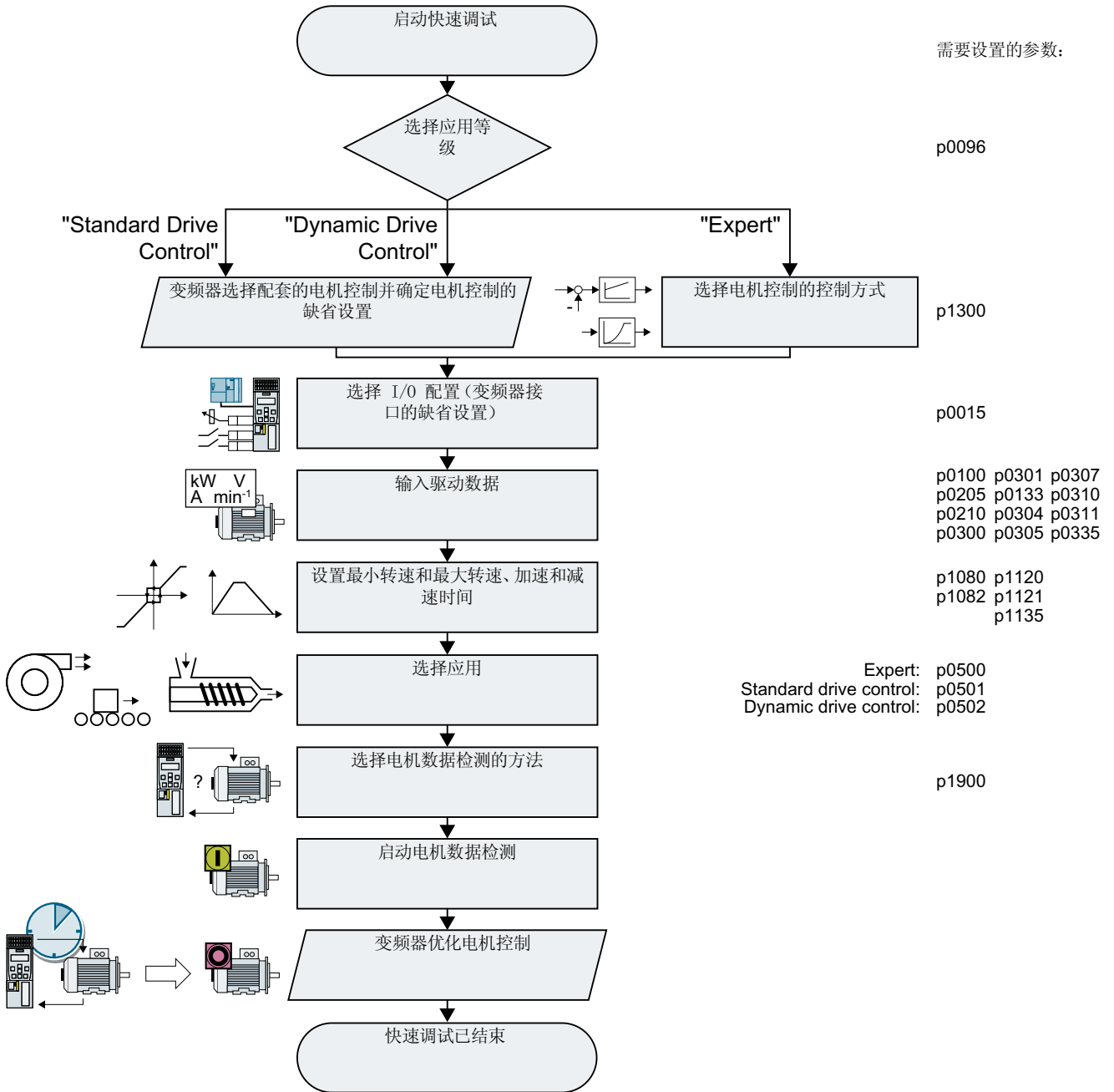
图 5-12 使用 PC 进行快速调试
