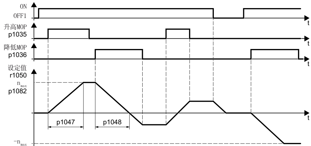
图 6-35 电动电位器的功能图
