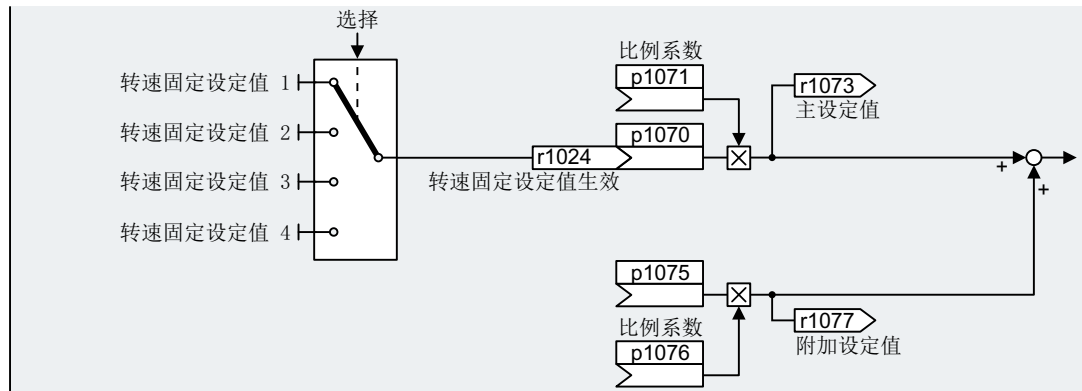
图 6-36 转速固定设定值设为设定值源
