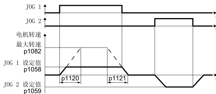
图 6-21 JOG 时电机的工作时序
