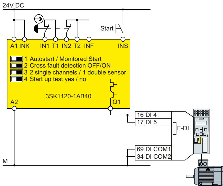
图 A-10 安全开关设备（如 SIRIUS 3SK11）的接线
