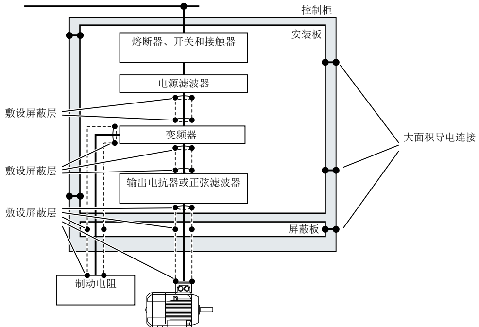
图 4-3 控制柜内部和外部的变频器布线
