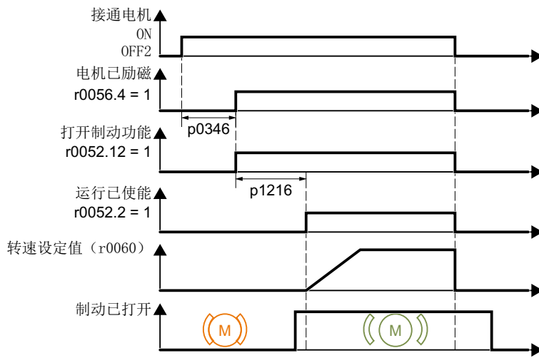
图 6-25 发出 OFF2 指令后电机抱闸的控制方式
