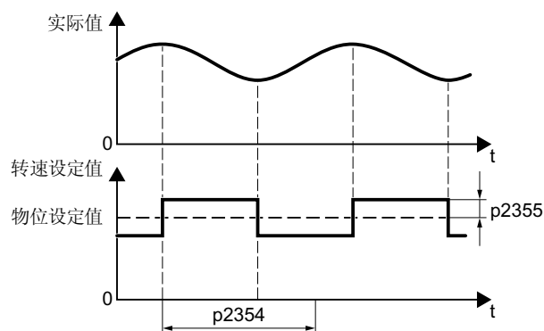
图 6-44 自动优化时的转速设定值和过程实际值示例
