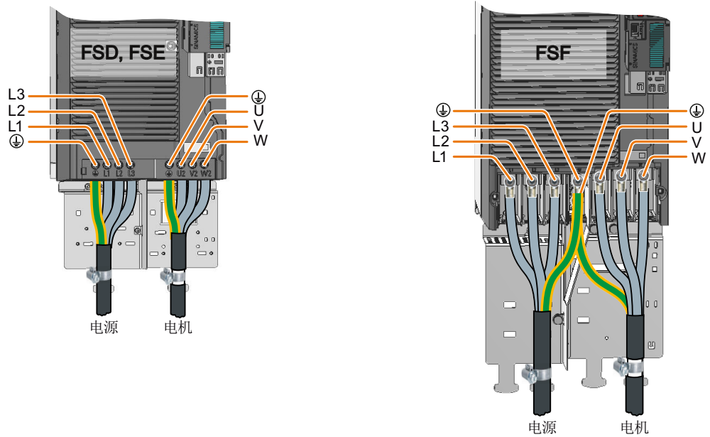
图 4-16 电源和电机接口
