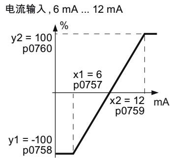
图 6-6 应用示例特性曲线
