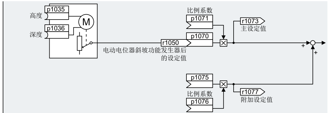
图 6-34 电动电位器设为设定值源
