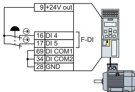
图 A-9 传感器（如：急停蘑菇按钮、限位开关）的接线
