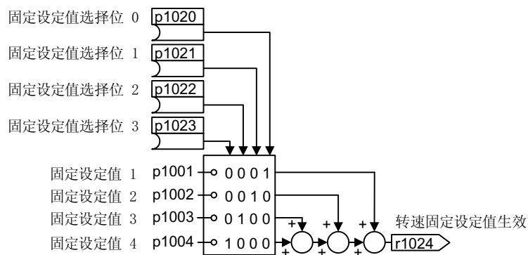
图 6-37 转速固定设定值的直接选择
