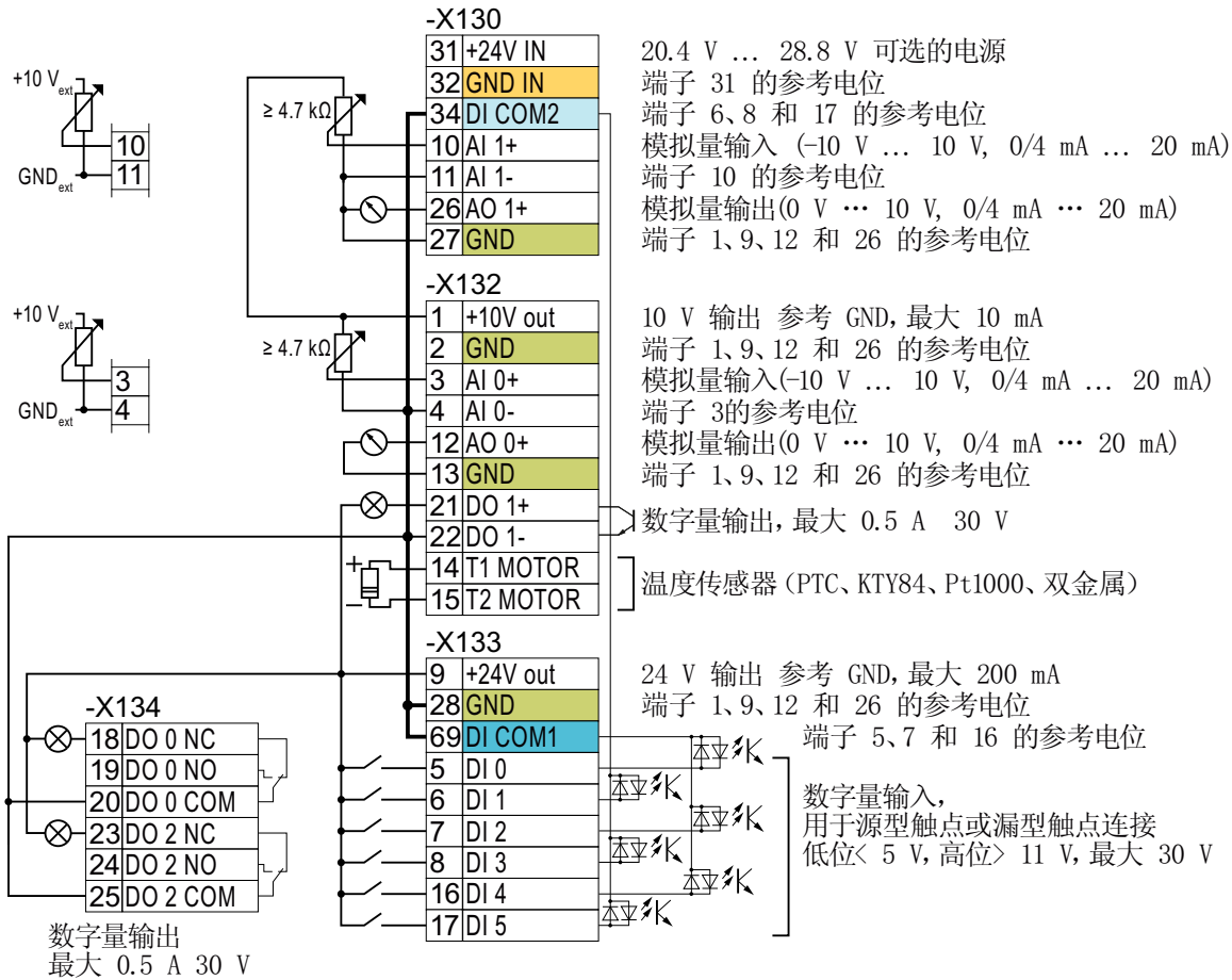
图 4-22 使用变频器内部 24 V 电源的数字量输入的布线示例
