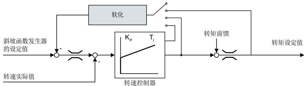
图 6-53 转速控制器中软化功能的作用
