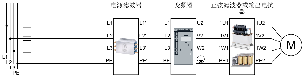
图 4-17 功率模块 PM250 的接线图
