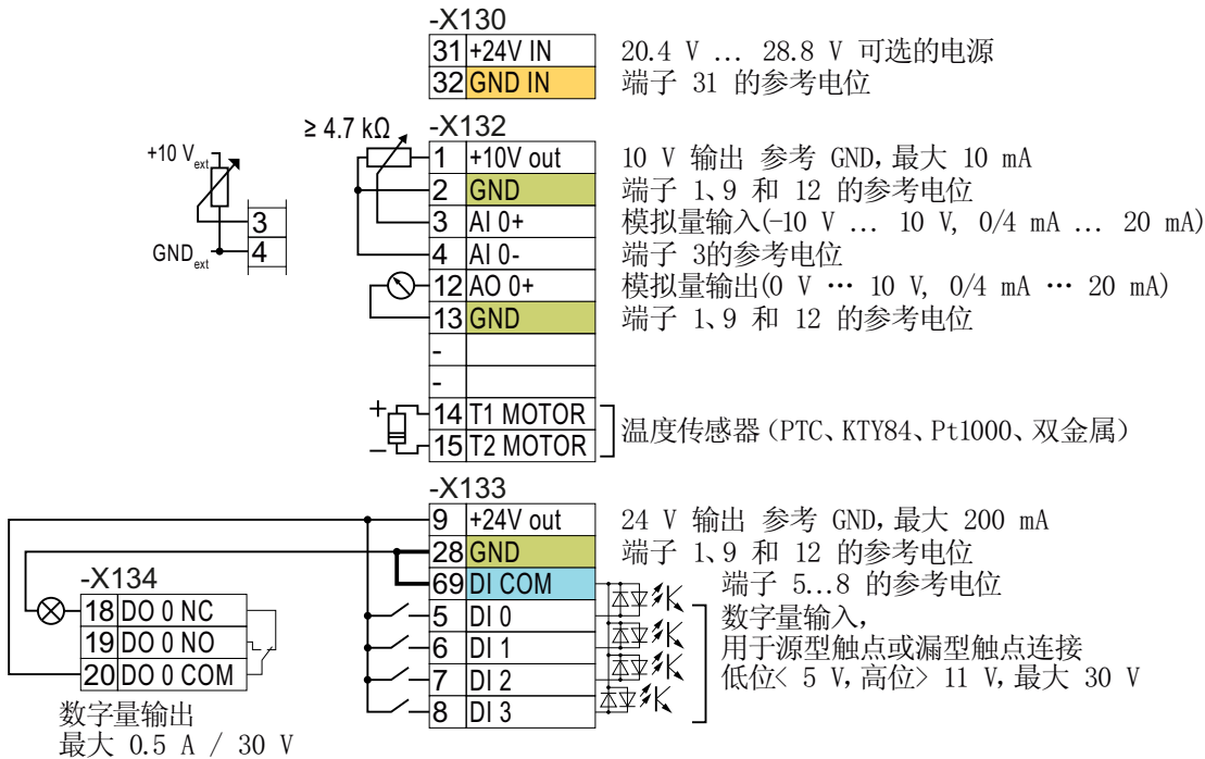
图 4-19 使用变频器内部 24 V 电源的数字量输入的布线示例
