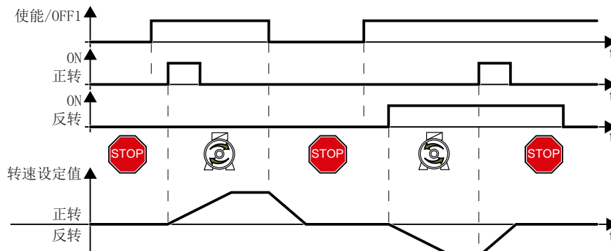
图 6-12 三线制控制，方法 1
