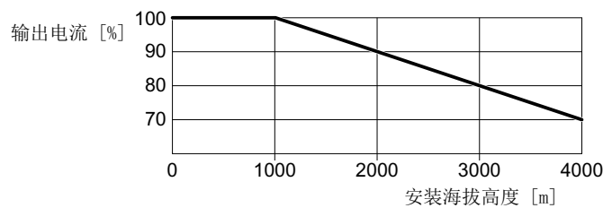
图 10-4 功率模块 PM240-2 和 PM240P-2 的特性曲线
