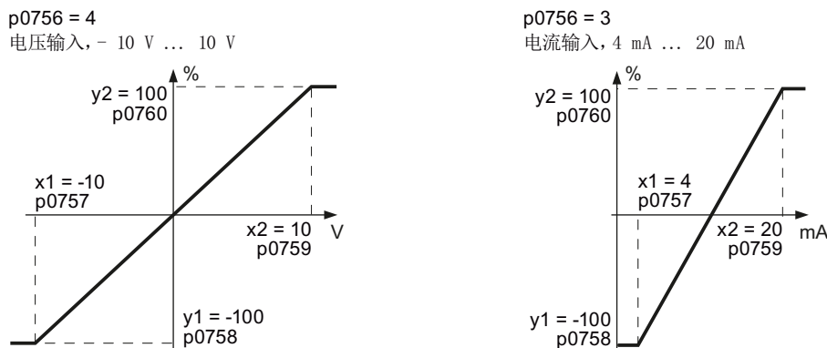
图 6-5 定标特性曲线示例
