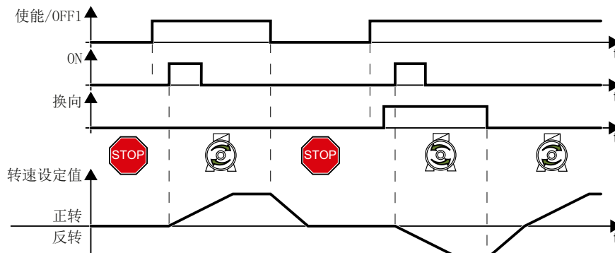
图 6-13 三线制控制，方法 2
