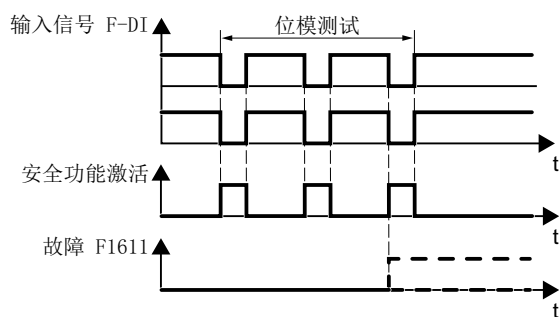
图 6-28 变频器对位模测试作出响应
