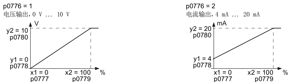
图 6-7 定标特性曲线示例
