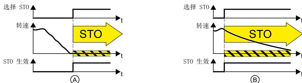
图 6-26 静态电机 (A) 和旋转电机 (B) 上的 STO 功能的工作原理
