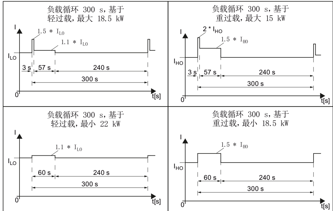
图 10-3 “重过载”和“轻过载”负载循环
