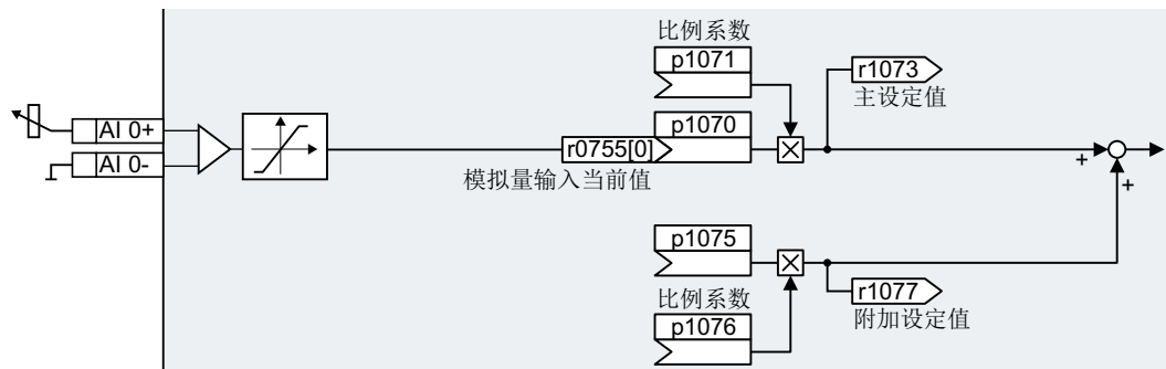
图 6-32 示例：模拟量输入 0 设为设定值源
