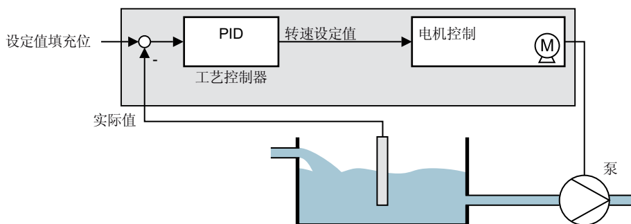
图 6-41 示例：工艺控制器用作流量控制器
