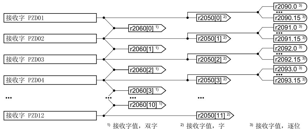
图 6-17 接收数据的互联
