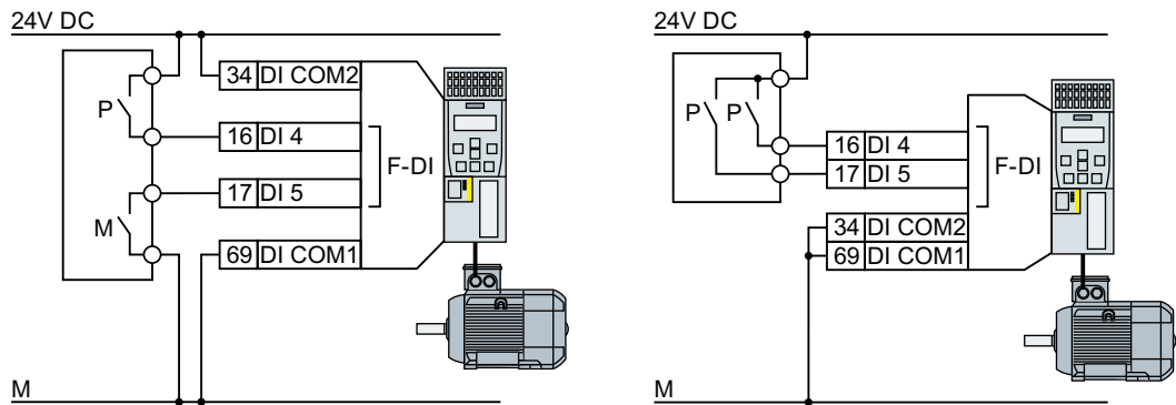
图 A-8 源型和漏型故障安全数字量输出的接线
