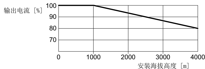
图 10-5 功率模块 PM230 和 PM250 的特性曲线
