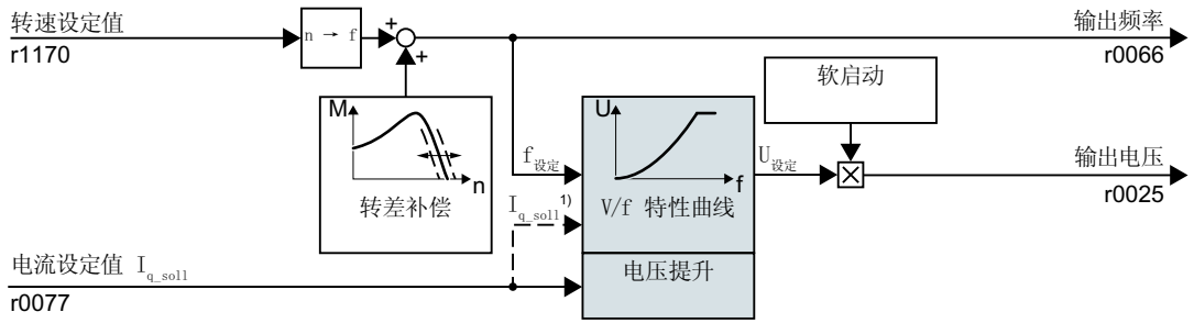
图 6-46 V/f 控制的简易功能图
