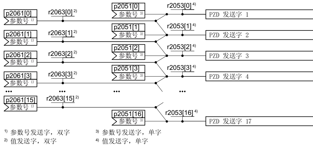
图 6-16 发送数据的互联
