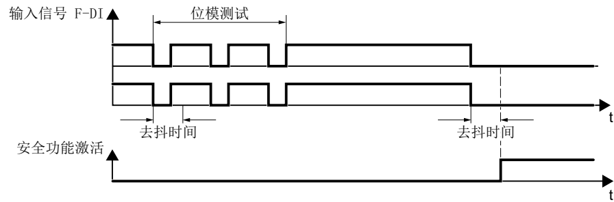
图 6-29 对短暂出现的信号进行滤波
