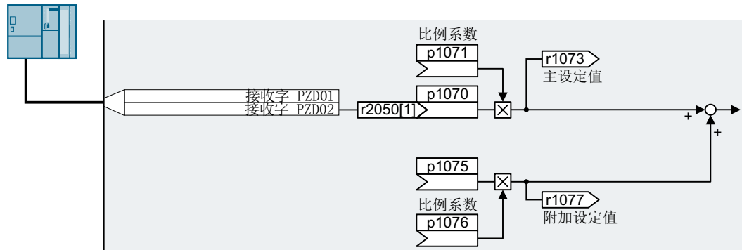
图 6-33 现场总线设为设定值源
