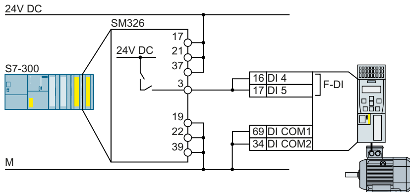
图 A-11 故障安全的数字量输出模块（如：SIMATIC F 模块）的接线
