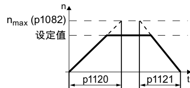
图 5-11 电机的升降时间
