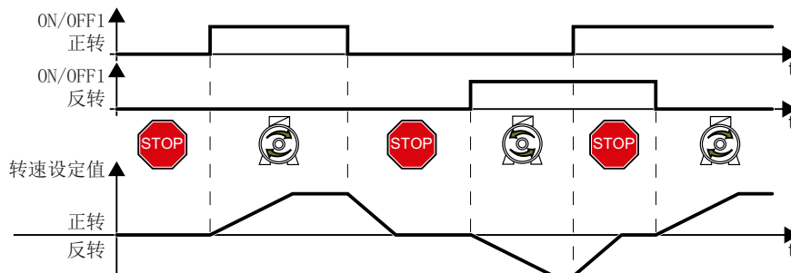
图 6-11 双线制控制，方法 3
