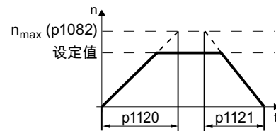
图 5-9 电机的升降时间
