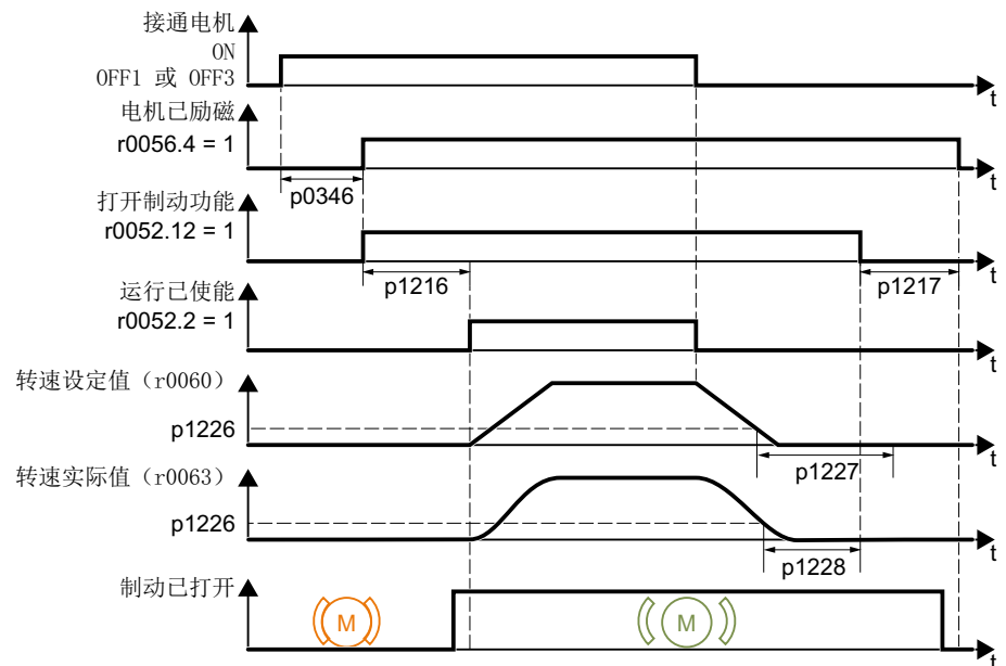
图 6-24 电机抱闸功能
