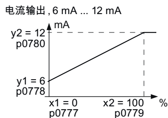
图 6-8 应用示例特性曲线
