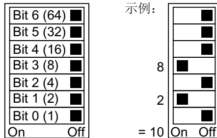
图 4-27 用于总线地址 10 的地址开关示例
