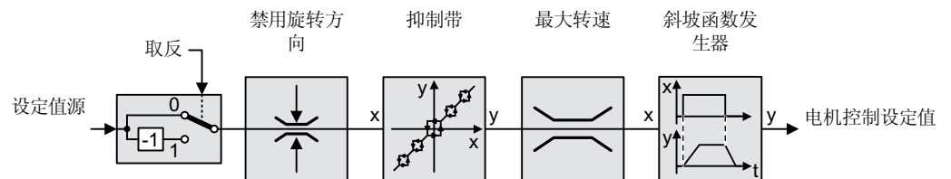
图 6-39 变频器内的设定值处理
