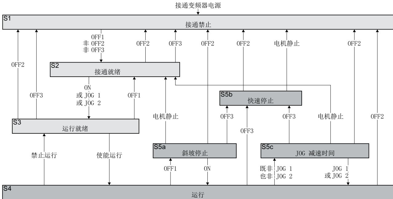
图 6-3 电机接通和关闭时变频器的顺序控制
