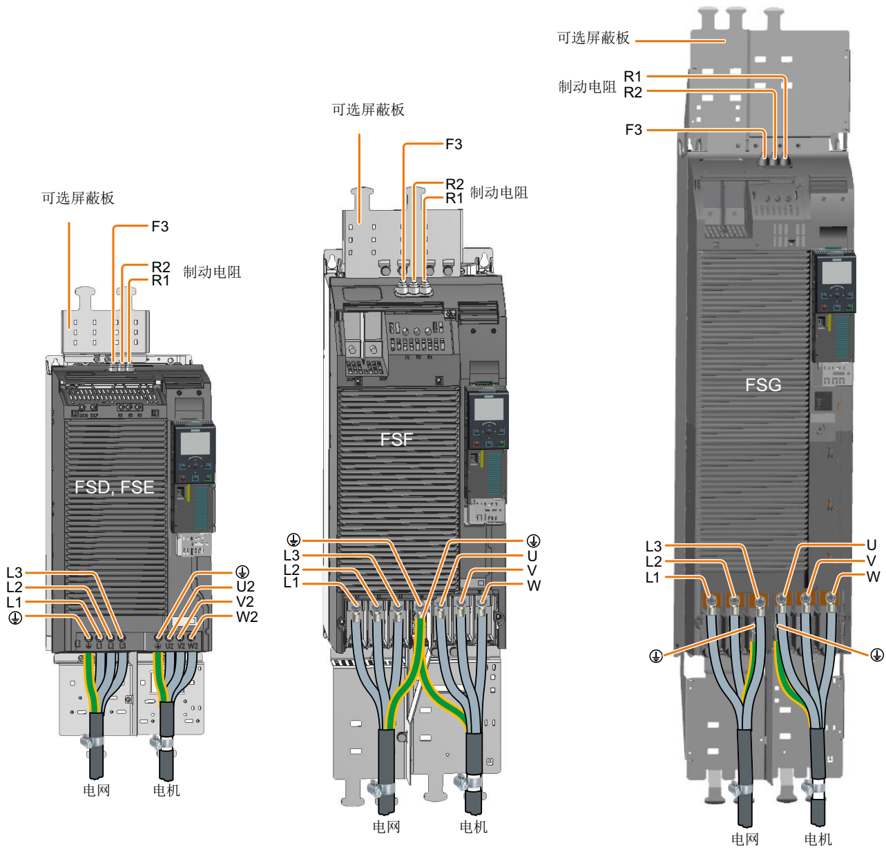
图 4-12 电源、电机和制动电阻的连接器
