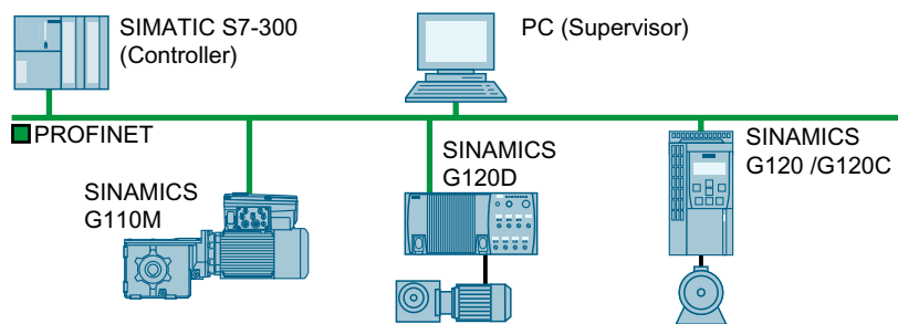
图 4-25 变频器在 PROFINET IO 模式中
