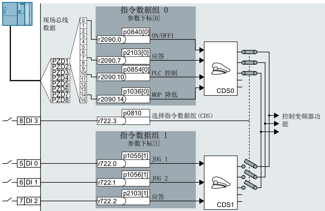
图 6-23 示例：控制方式从端子排切换到 PROFIBUS 或 PROFINET
