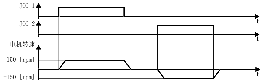
图 5-4 出厂设置中电机的 JOG 模式
