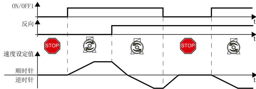
图 6-9 双线制控制：方法 1
