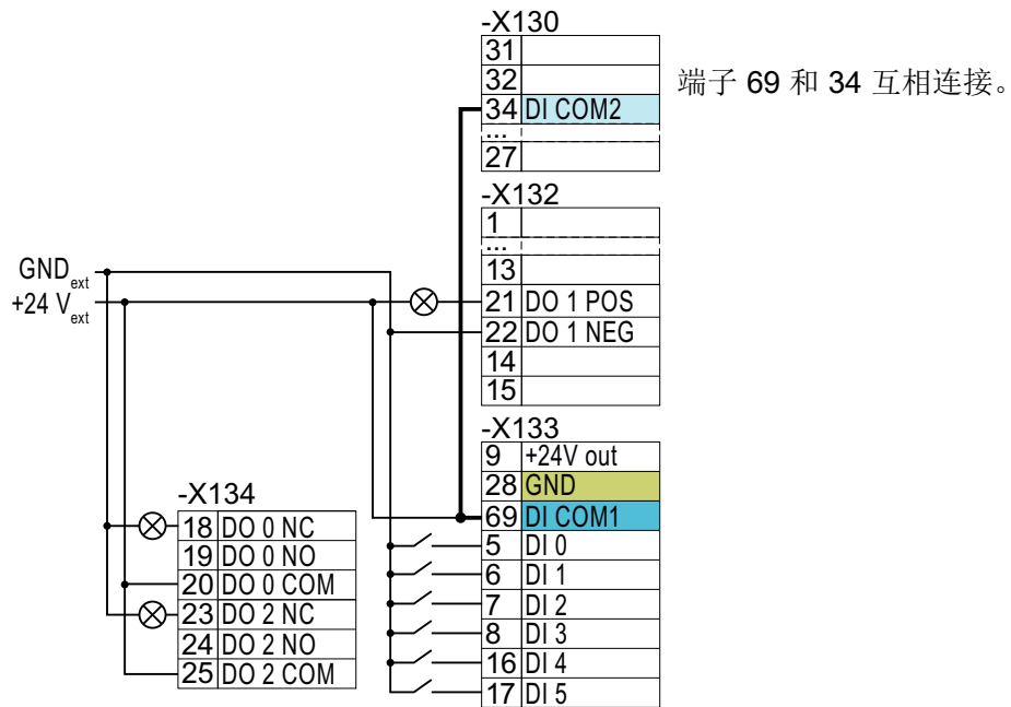
连接漏型触点和外部电源
