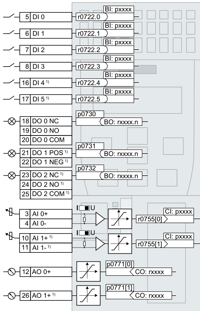
图 6-4 输入输出的内部接线
