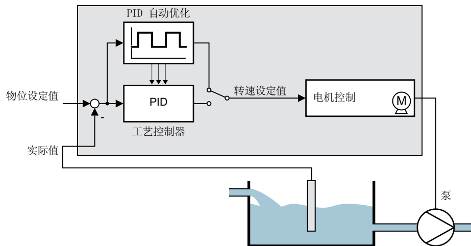
图 6-43 自动优化示例（物位调节）
