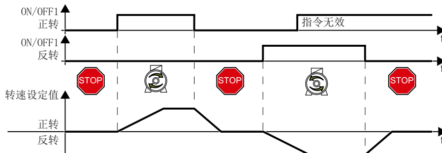
图 6-10 双线制控制，方法 2
