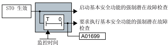
图 6-30 强制潜在故障检查的启动和监控 (Teststopp)
