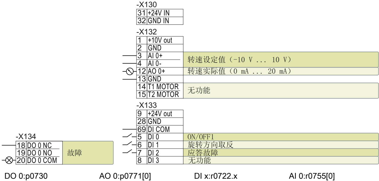
图 4-21 控制单元 CU240B-2 的出厂设置
