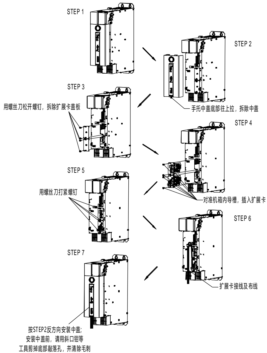
图 A.2 扩展卡安装步骤示意图
