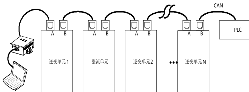
图 6.3 CANopen 总线组网接线 2
