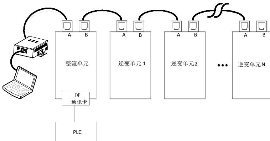
图 6.5 PROFIBUS-DP 转 CANopen 组网拓扑图
