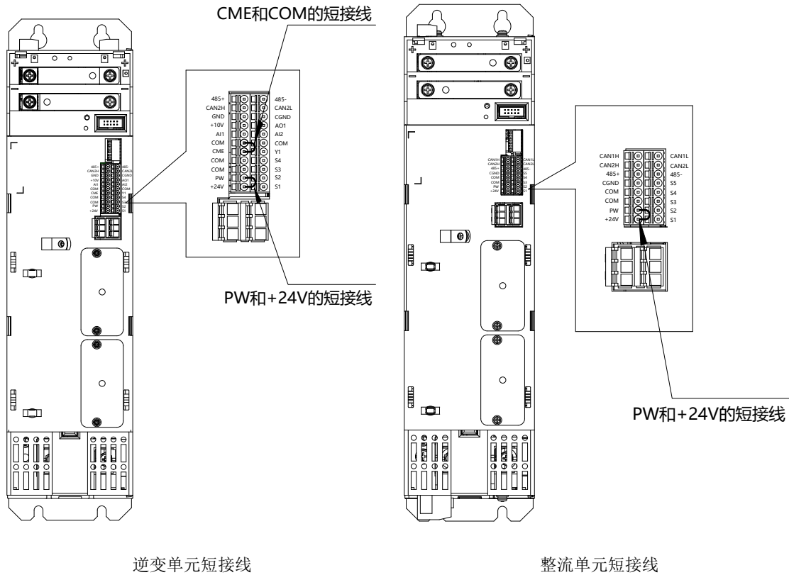
图 4.14 短接线位置示意图
