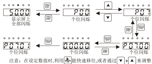
图 5.4 设定密码示意图
