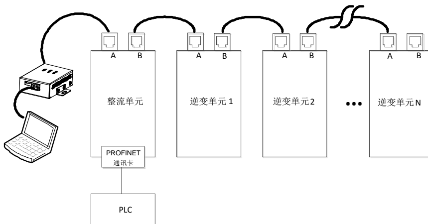
图 6.8 PROFINET 转 CANopen 组网拓扑图
