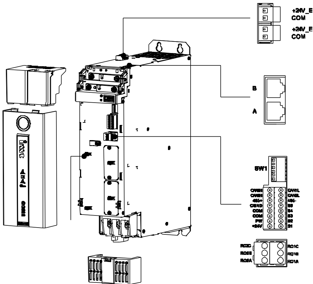
图 4.11 整流单元控制回路端子示意图
