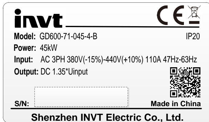
图 3.5 整流单元铭牌
