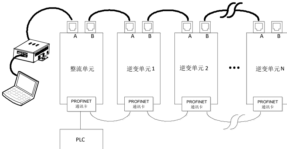
图 6.12 Profinet 通讯组网线型网络拓扑图
