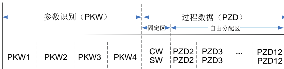
图 6.7 报文结构
