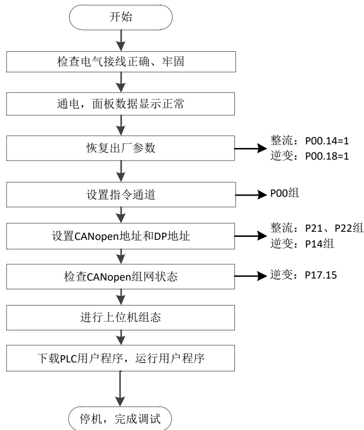
图 6.6 DP 转 CANopen 组网调试步骤
