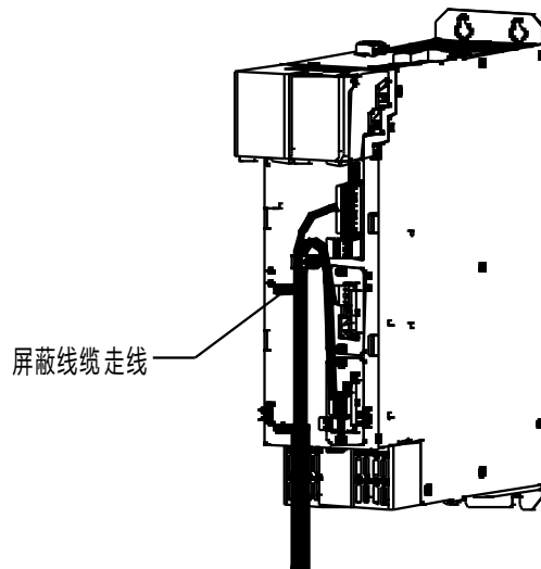
图 A.4 走线方式示意图
