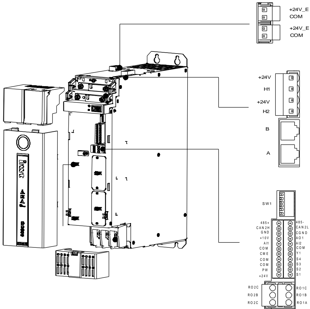
图 4.13 逆变单元控制回路端子示意图
