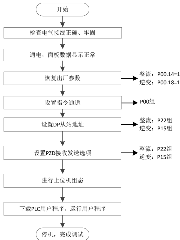
图 6.11 DP 组网调试步骤
