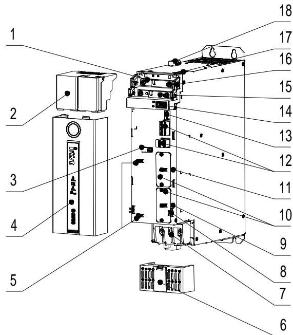
图 3.8 整流单元结构示意图
