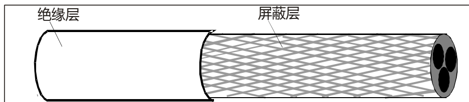
图 E.2 电缆剖面
