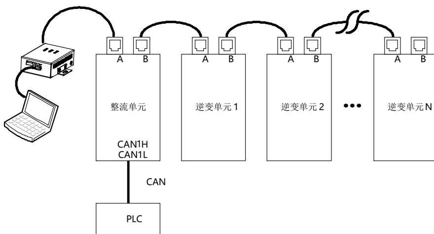
图 6.2 CANopen 总线组网接线 1
