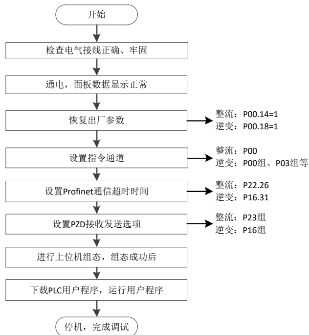
图 6.14 PROFINET 通讯组网调试步骤
