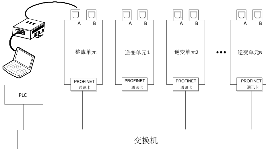
图 6.13 PROFINET 通讯组网星型网络拓扑图
