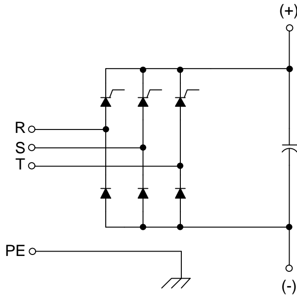
图 3.3 整流单元（160kW/355kW）主回路简图
