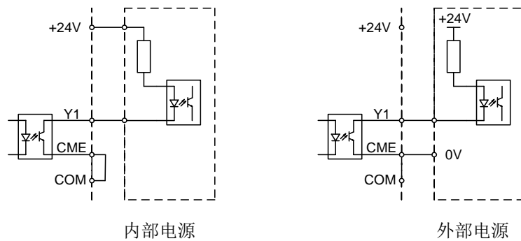
图 4.17 数字量输出接线示意图
