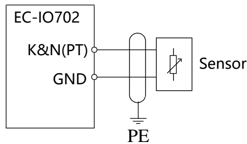
图 5.1 IO 扩展卡温度传感器接线图
