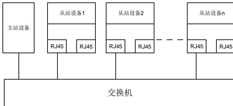
图 A.6 星型网络拓扑电气连接图
