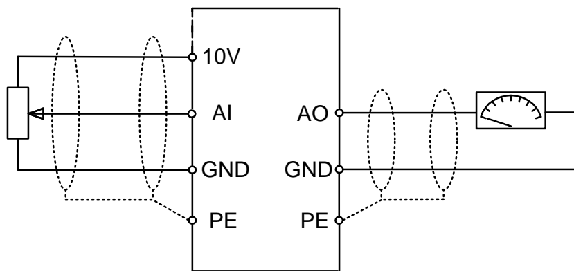
图 4.19 模拟量输入输出接线示意图
