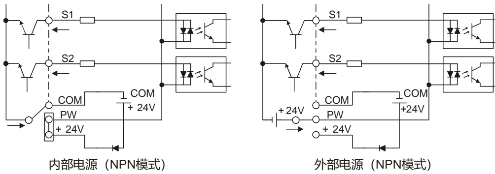
图 4.15 NPN 接线模式示意图
