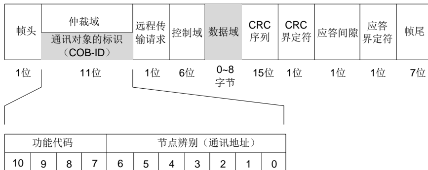
图 6.4 报文结构图
