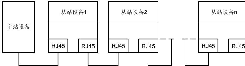
图 A.5 线型网络拓扑电气连接图
