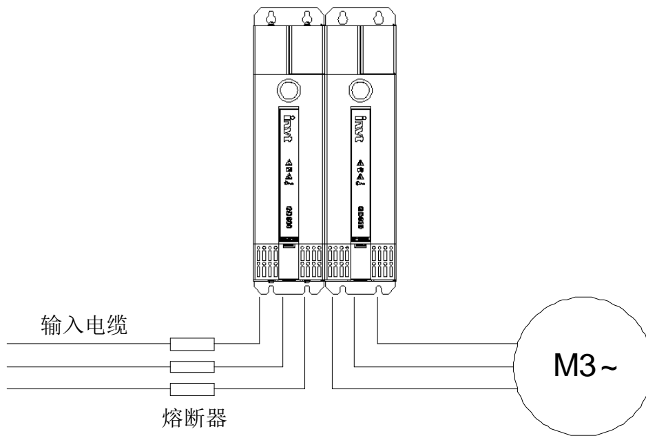
图 4.21 熔断器配置图
