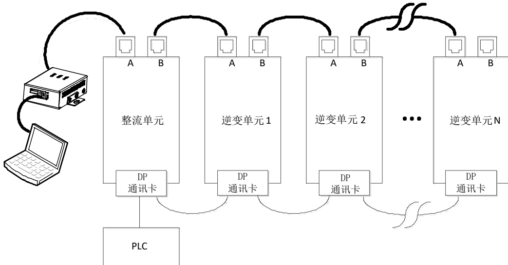
图 6.10 PROFIBUS-DP 通讯组网拓扑图
