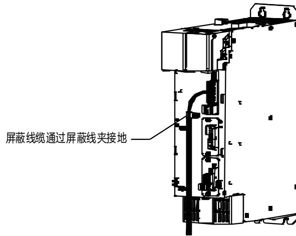
图 A.3 屏蔽线接地示意图
