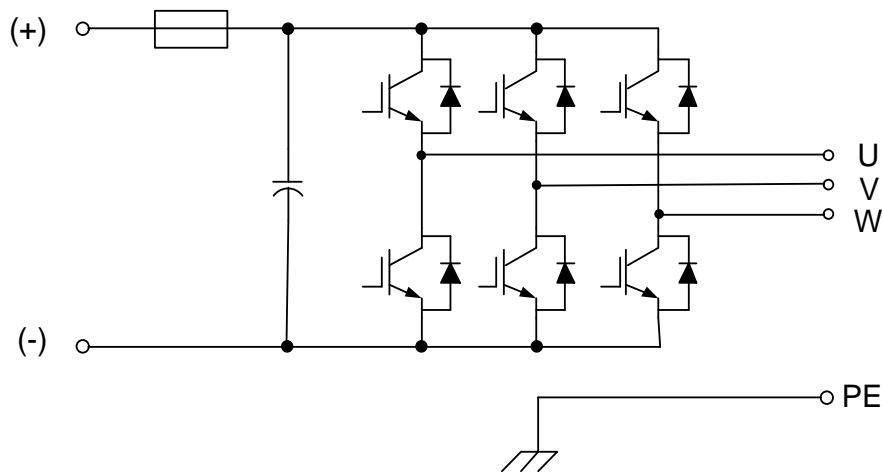
图 3.4 逆变单元主回路简图
