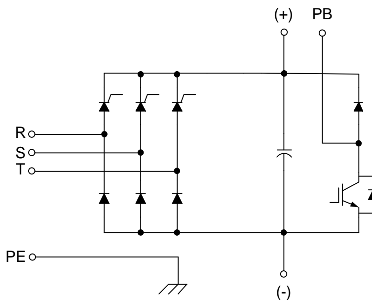
图 3.2 整流单元（45kW）主回路简图
