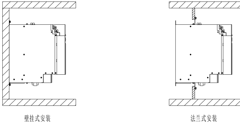
图 4.2 单元安装方式
