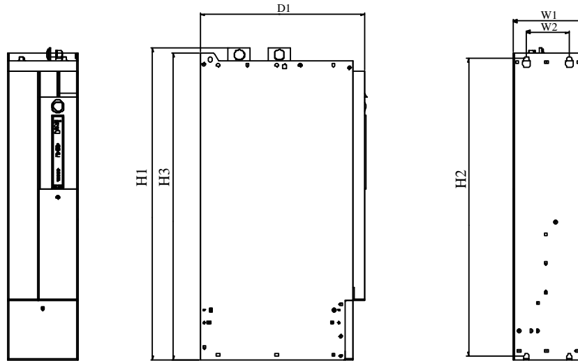
图 D.5 380V 355kW 整流单元壁挂安装示意图
