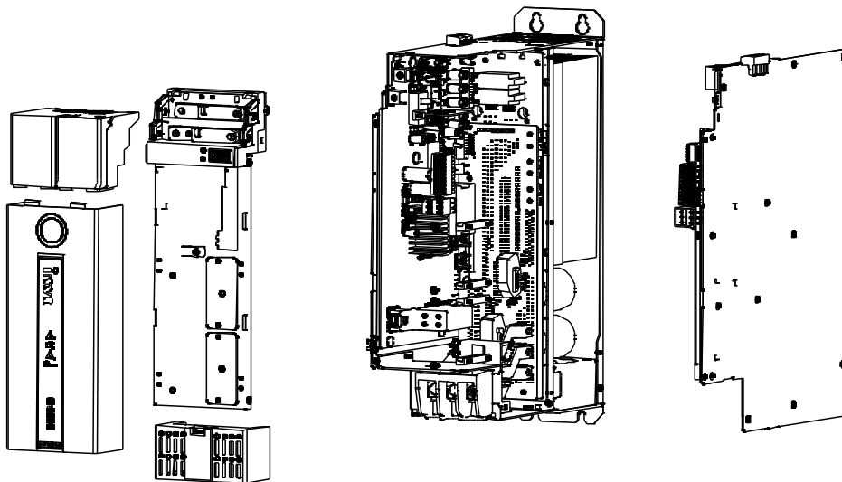
图 D.2 37kW 逆变单元结构图
