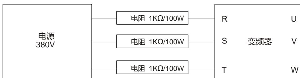
图 10.3 380V 驱动装置充电电路示例
