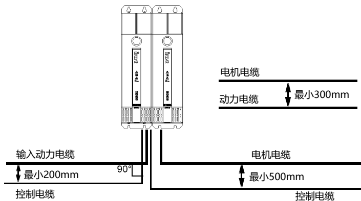
图 E.4 电缆布线距离
