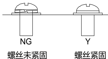
图 4.8 螺丝安装是否正确示意图
