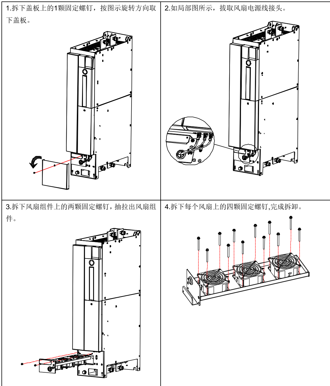
图 10.2 355kW 整流单元风扇维护示意图
