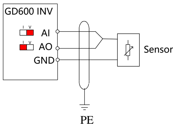
图 5.6 AI/AO 检测电机温度接线图
