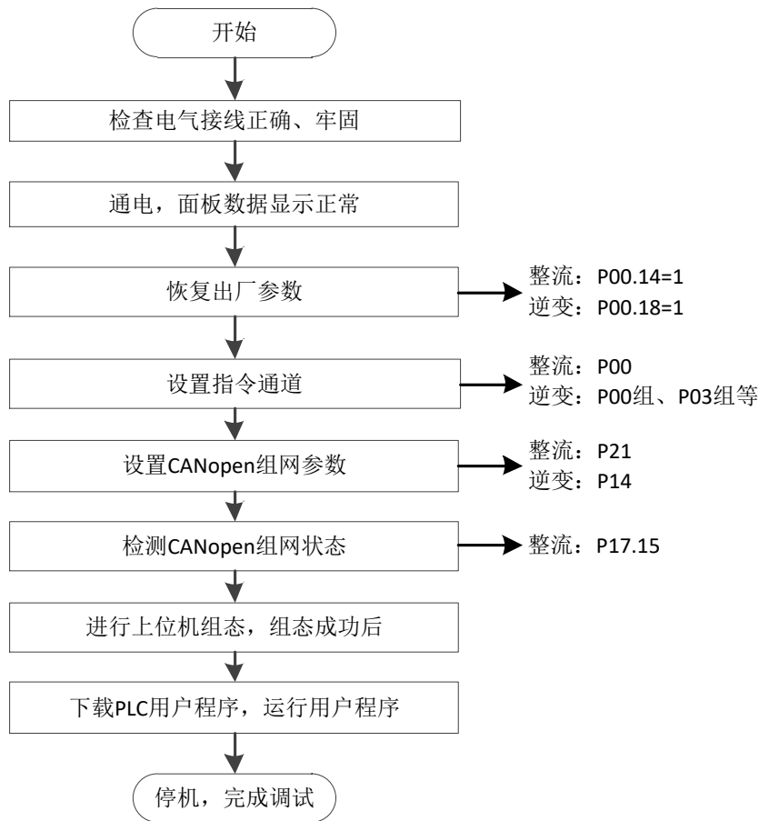
图 6.9 PROFINET 转 CANopen 组网调试步骤
