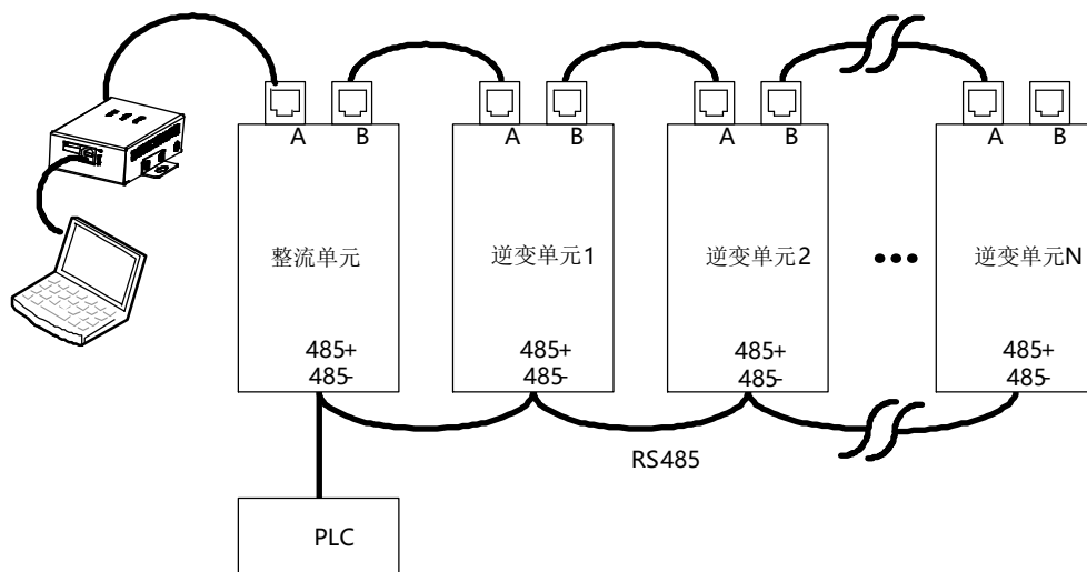
图 6.1 网络拓扑
