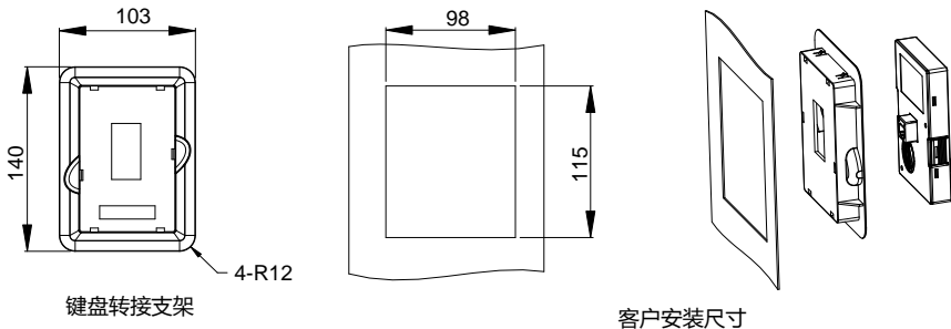
图 C.2 380V 1.5~500kW、660V 22~630kW 键盘安装架（选配）图
