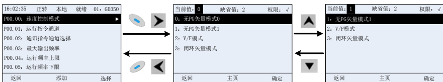
图 5.15 参数选择编辑界面示意图
