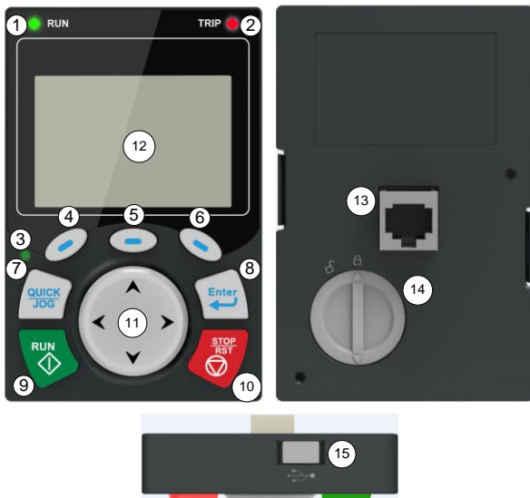
图 5.1 键盘示意图
