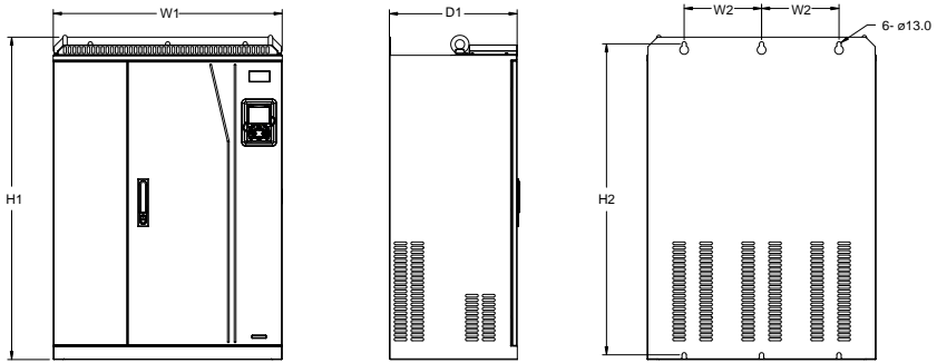
图 C.8 380V 220-315kW 壁挂安装示意图
