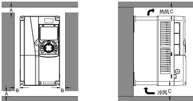
图 4.3 单台安装
