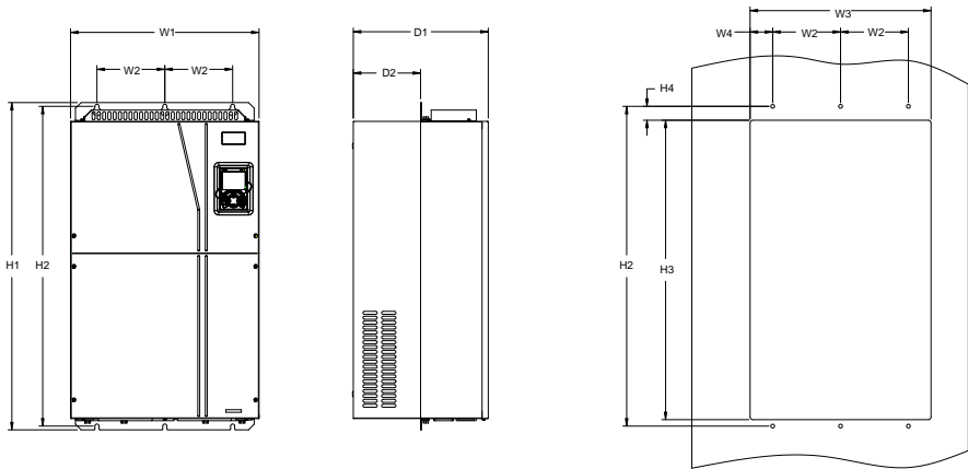
图 C.18 660V 160-220kW 法兰安装示意图表 C.5 660V 法兰安装尺寸表 (单位: mm)
