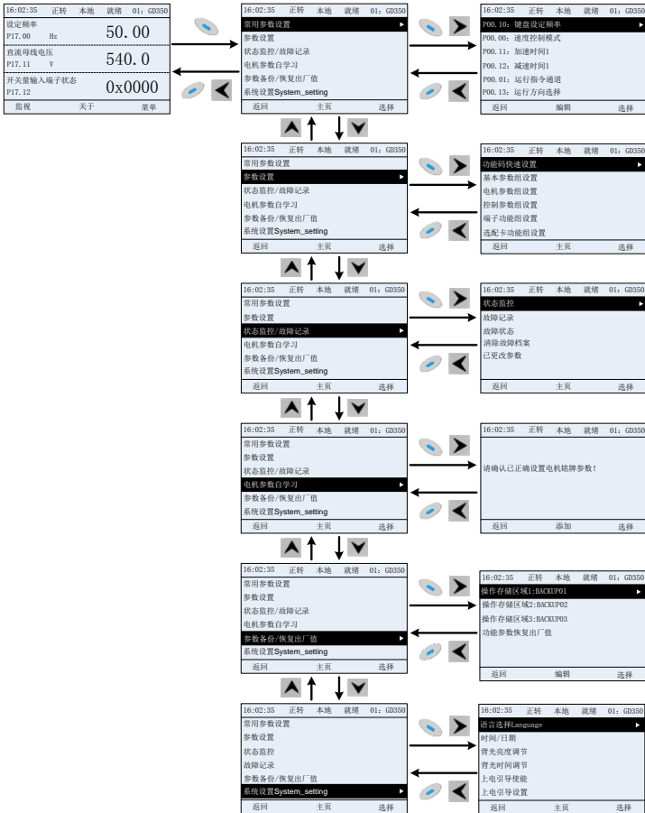
图 5.9 进入/退出各级菜单示意图 2
