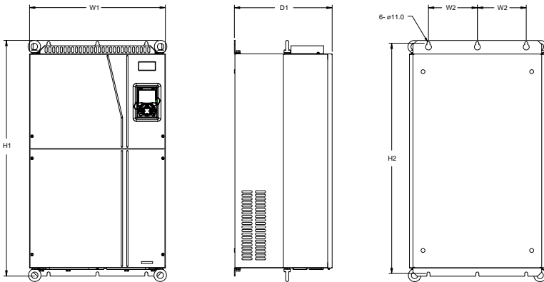
图 C.7 380V 132-200kW 壁挂安装示意图
