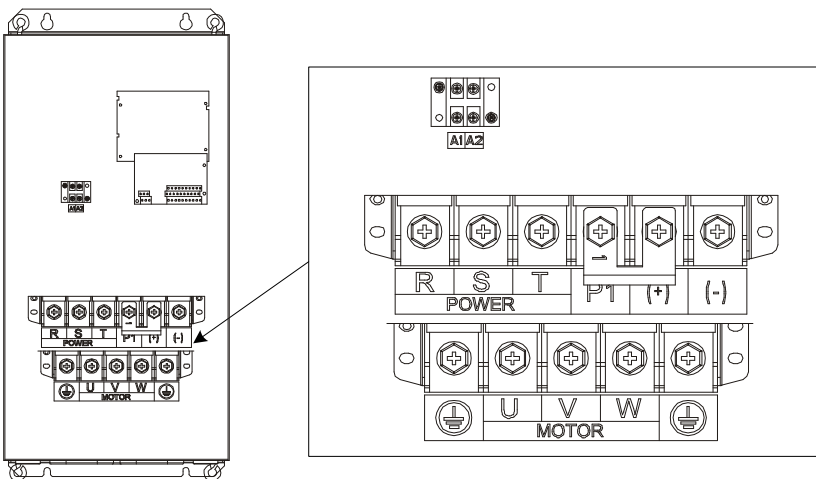
图 4.13 660V 55-132kW 主回路端子示意图
