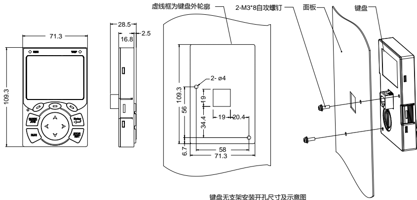
键盘无支架安装开孔尺寸及示意图
