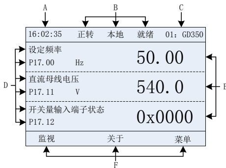
图 5.2 液晶显示器主界面
