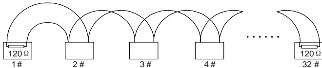
图 10.2 菊花接法现场接线图
