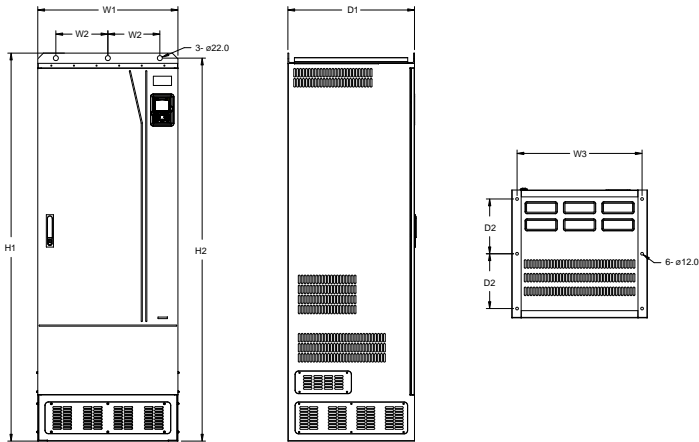
图 C.20 660V 400-630kW 落地安装示意图
