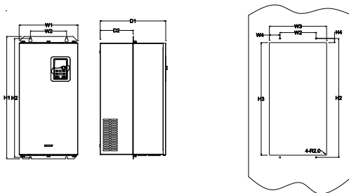
图 B.13 660V 22-132kW 法兰安装示意图
