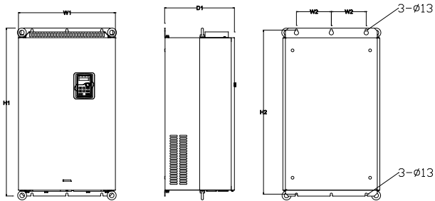
图 B.3 380V 132-200kW 壁挂安装示意图
