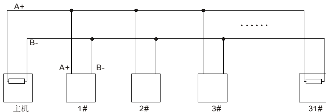
图 11.3 菊花简化接线图
