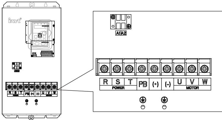
图 4.14 380V 37~55kW 主回路端示意图
