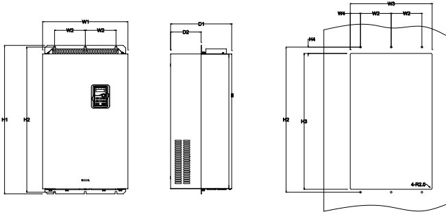
图 B.14 660V 160-220kW 法兰安装示意图
