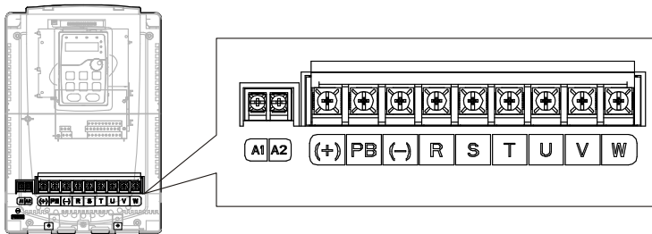
图 4.12 380V 15~18kW 主回路端示意图
