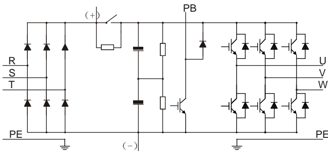
图 3.2 380V（小于 55kW（含））主回路简图
