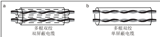
图 C.3 动力电缆布线
