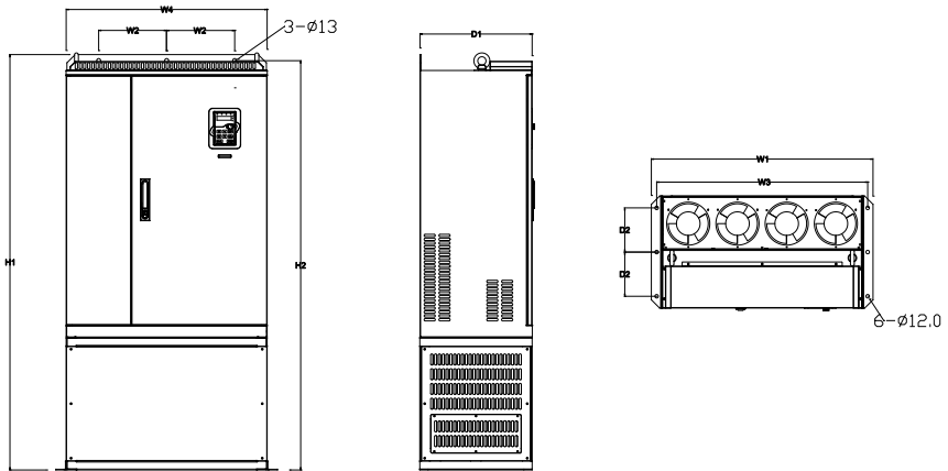
图 B.8 380V 220-315kW 落地安装示意图
