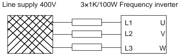
图 10.1 380V 驱动装置充电电路示例
