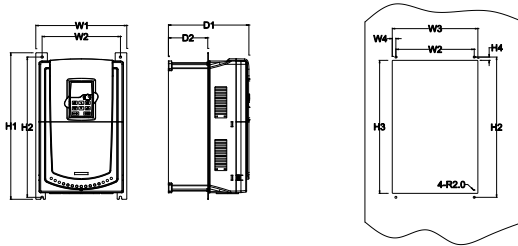
图 B.5 380V 1.5-30kW 法兰安装示意图
