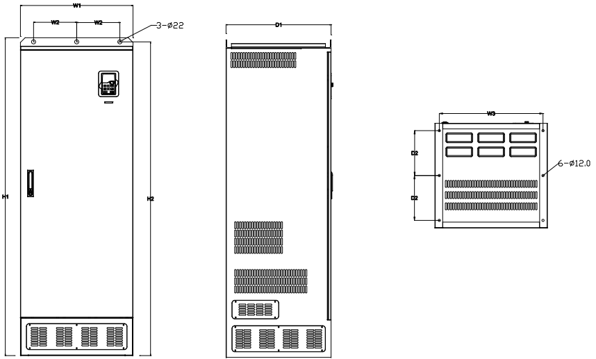
图 B.16 660V 400-630kW 落地安装示意图
