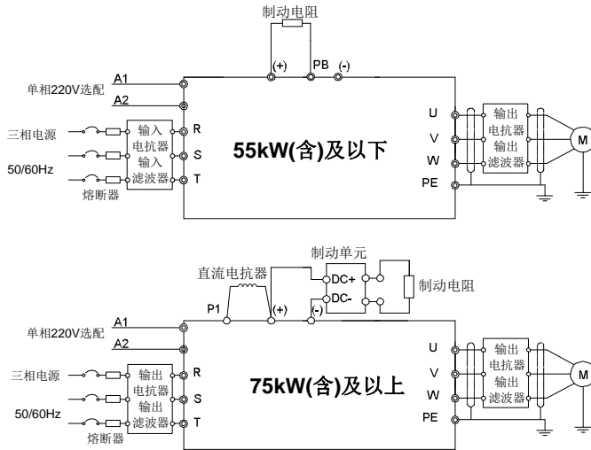
图 4.7 380V 主回路接线图
