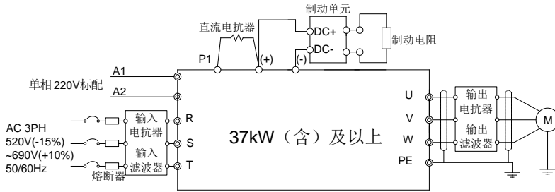
图 4.8 660V 主回路接线图
