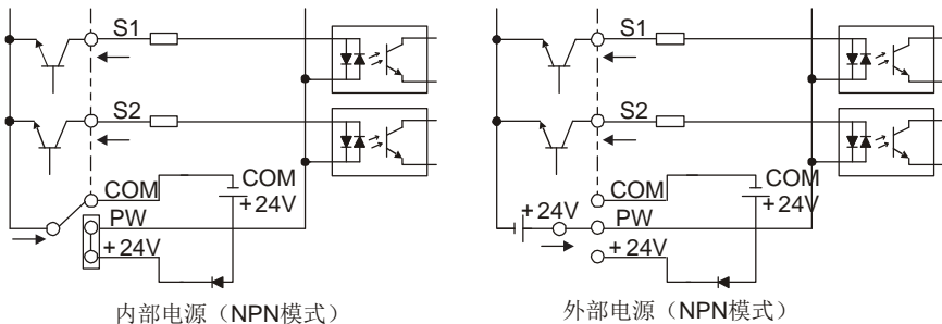
图 4.24 NPN 模式示意图
