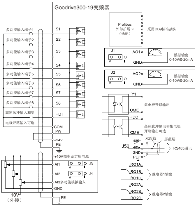
图 4.21 控制回路接线图
