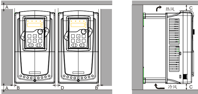
图 4.4 并行安装
