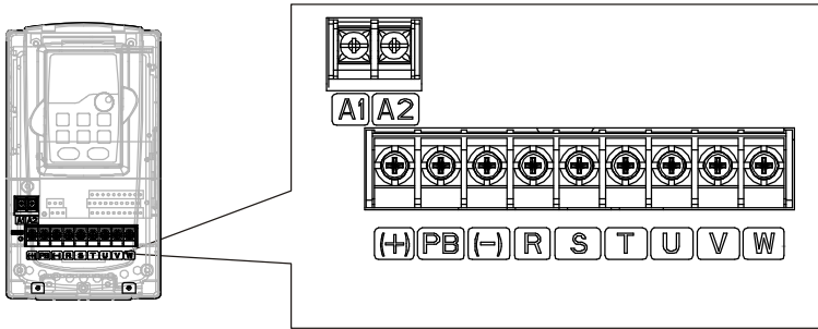
图 4.10 380V 4~5.5 kW 主回路端示意图
