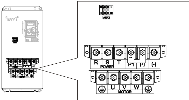
图 4.16 380V 75~110kW、660V 55~132kW 主回路端子示意图
