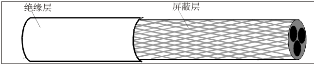
图 C.2 电缆剖面
