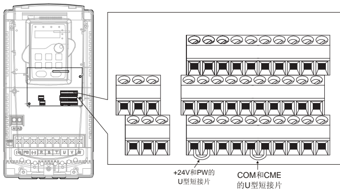
图 4.23 U 型短接位置示意图
