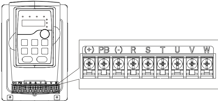
图 4.9 380V 1.5~2.2kW 主回路端子示意图
