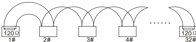
图 11.2 菊花接法现场接线图
