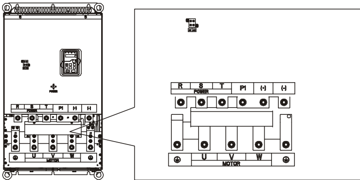
图 4.17 380V 132~200kW、660V 160~220kW 主回路端子示意图
