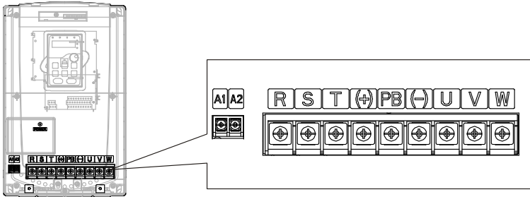
图 4.13 380V 22~30kW 主回路端示意图
