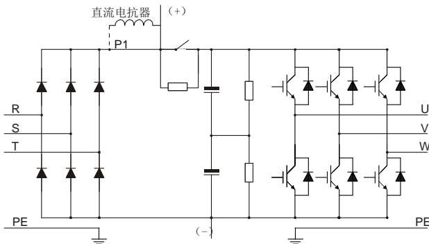
图 3.1 380V（大于 75kW（含））主回路简图
