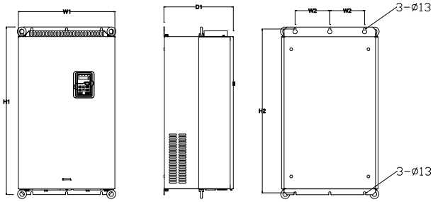
图 B.11 660V 160-220kW 壁挂安装示意图
