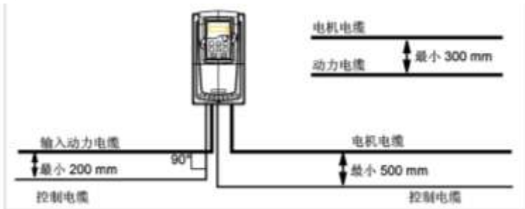
图 C.4 布线距离
