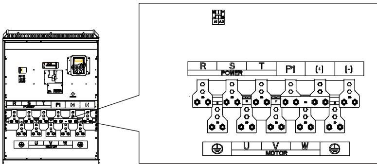
图 4.18 380V 220~315kW、660V 250~350kW 主回路端子示意图
