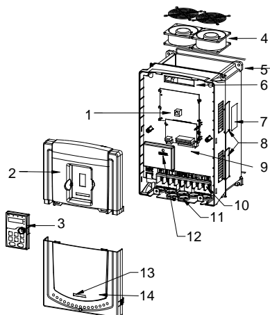
图 3.6 产品结构示意图
