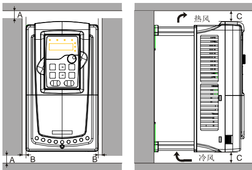
图 4.3 单台安装
