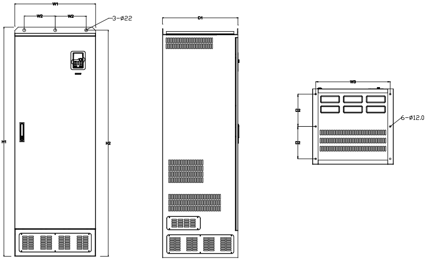
图 B.9 380V 350-500kW 落地安装示意图
