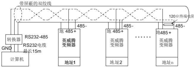
图 11.4 菊花接法运用图
