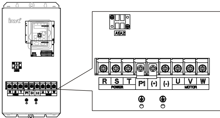
图 4.15 660V 22~45kW 主回路端示意图
