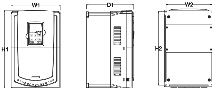
图 B.1 380V 1.5-30kW 壁挂安装示意图
