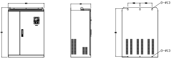
图 B.12 660V 250-350kW 壁挂安装示意图
