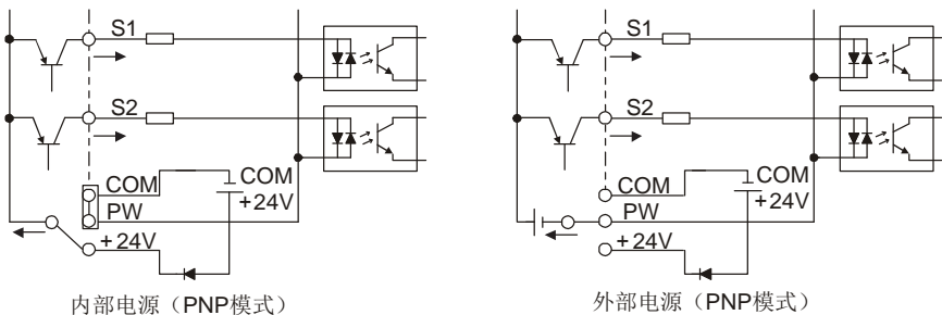
图 4.25 PNP 模式示意图
