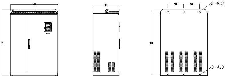
图 B.4 380V 220-315kW 壁挂安装示意图
