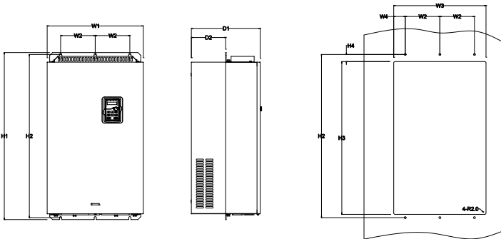
图 B.7 380V 132-200kW 法兰安装示意图
