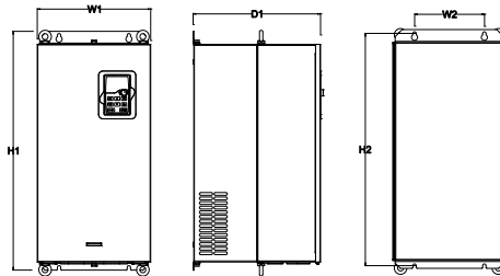
图 B.10 660V 22-132kW 壁挂安装示意图
