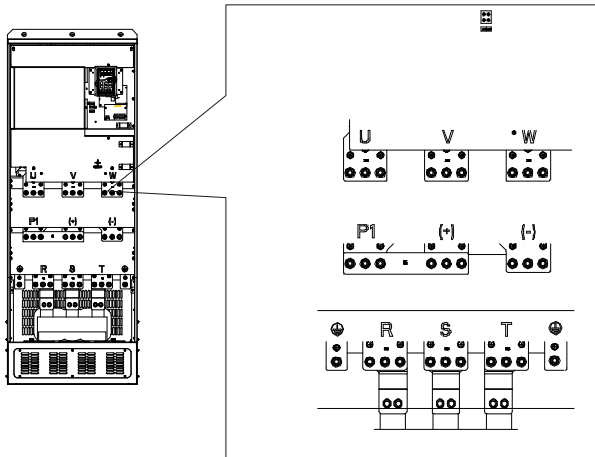
图 4.19 380V 350~500kW、660V 400~630kW 主回路端子示意图
