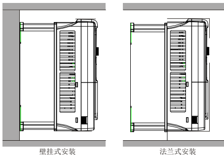
图 4.2 安装方式
