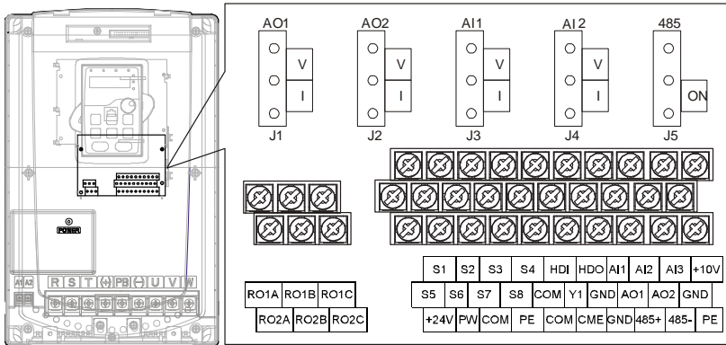
图 4.22 控制端子示意图
