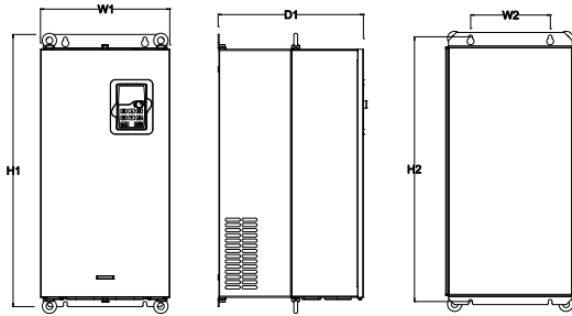
660V 22-132kW 壁挂安装示意图
