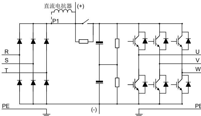
图 3-2 380V ( \geq 37\text{kW} ) 主回路简图
