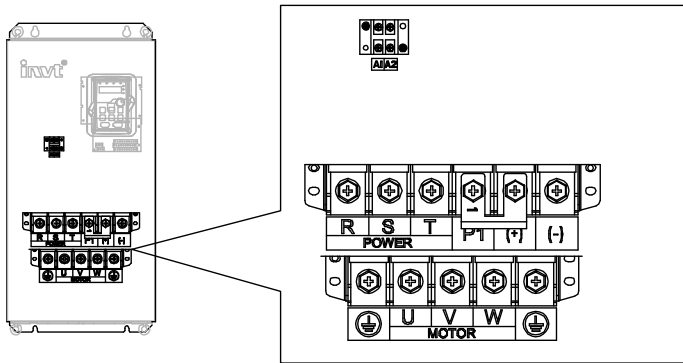
图 4-16 380V 75~110kW、500V 75kW 和 660V 55~132kW 主回路端子示意图
