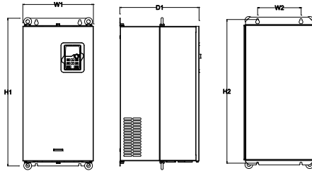
380V 37-110kW 壁挂安装示意图
