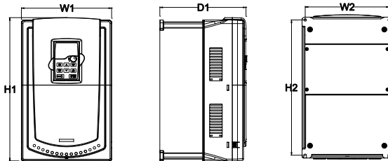
380V 1.5-30kW 壁挂安装示意图
