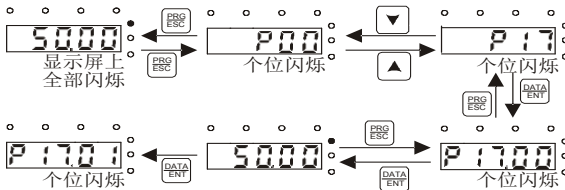
图 5-5 查看参数示意图
