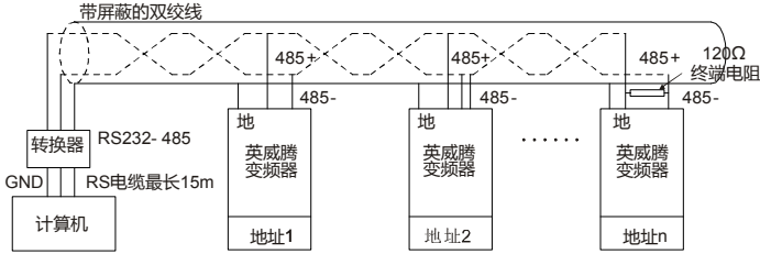
图 11-4 菊花接法运用图
