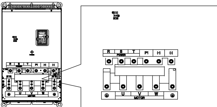
图 4-17 380V 132~200kW 和 660V 160~220kW 主回路端子示意图
