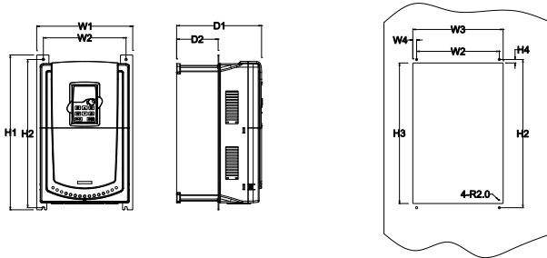
380V 1.5-30kW 法兰安装示意图
