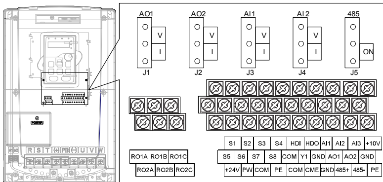
图 4-22 控制端子示意图
