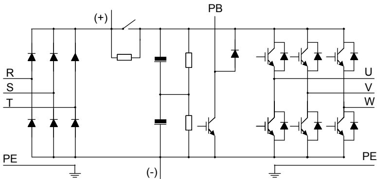
图 3-1 380V ( \leq 30\text{kW} ) 主回路简图
