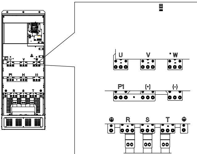
图 4-19 380V 350~500kW 和 660V 400~630kW 主回路端子示意图
