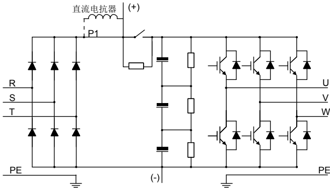
图 3-5 660V 主回路简图
