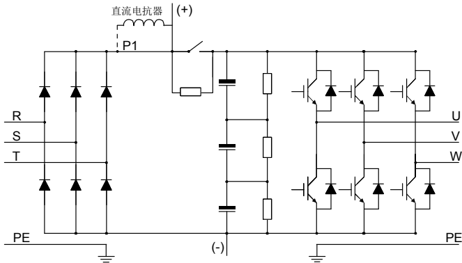
图 3-4 500V ( \geq 22\text{kW} ) 主回路简图
