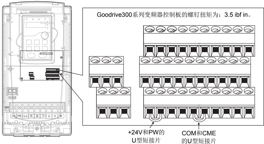
图 4-23 U 型短接位置示意图
