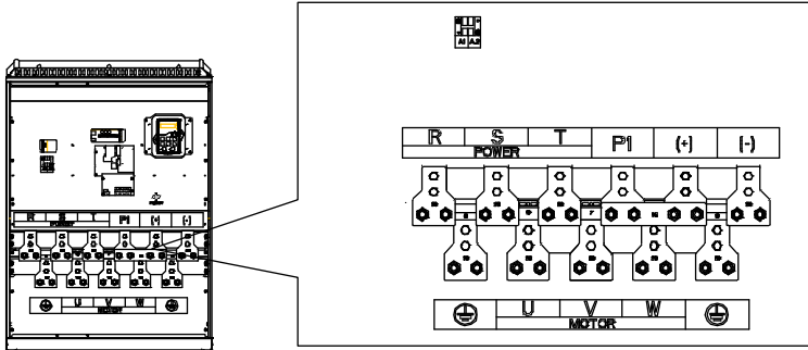
图 4-18 380V 220~315kW 和 660V 250~350kW 主回路端子示意图
