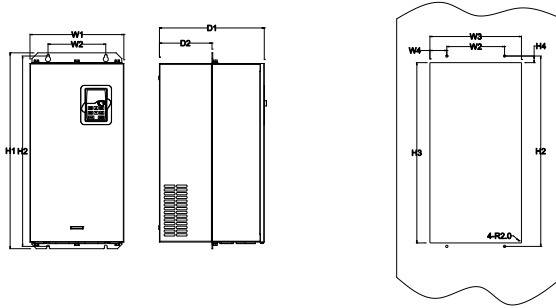
660V 22-132kW 法兰安装示意图
