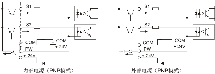
图 4-25 PNP 模式示意图
