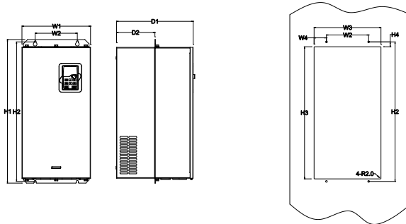
380V 37-110kW 法兰安装示意图
