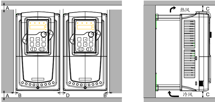
图 4-4 并行安装
