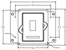
键盘转接支架
