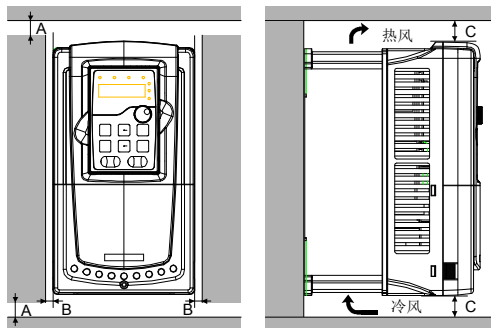
图 4-3 单台安装
