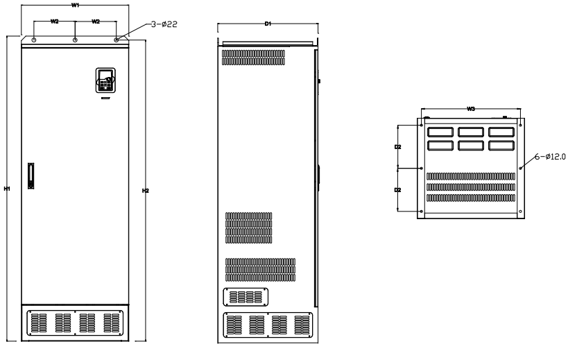
380V 350-500kW 落地安装示意图
