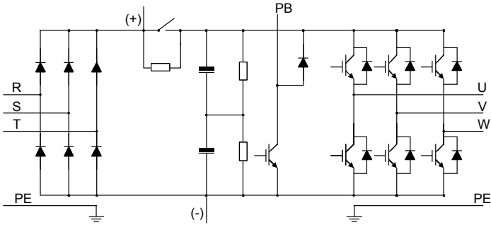
图 3-3 500V ( \leq 18.5\text{kW} ) 主回路简图
