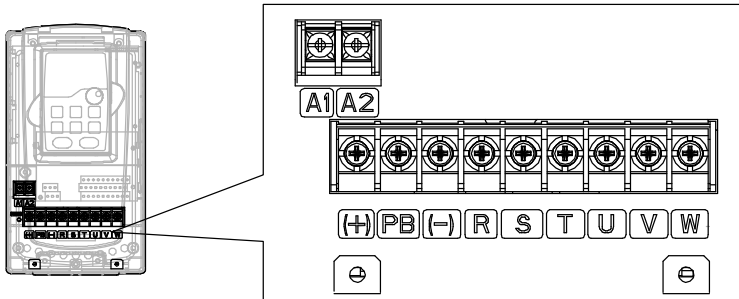
图 4-11 380V 4~5.5 kW 主回路端子示意图
