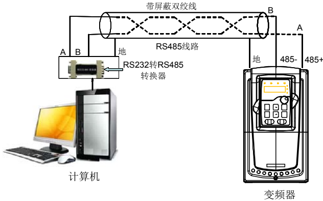
图 11-1 RS485 单机应用时的物理接线图
