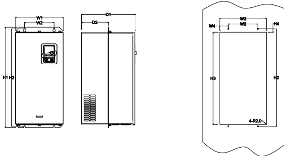
500V 22-75kW 法兰安装示意图
