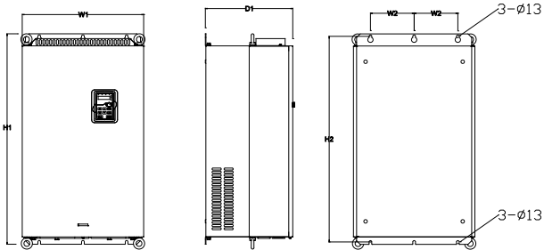
660V 160-220kW 壁挂安装示意图
