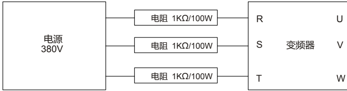
图 10-1 380V 驱动装置充电电路示例
