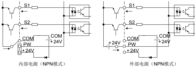
图 4-24 NPN 模式示意图
