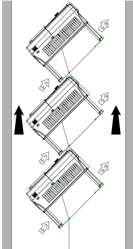
图 4-6 倾斜安装
