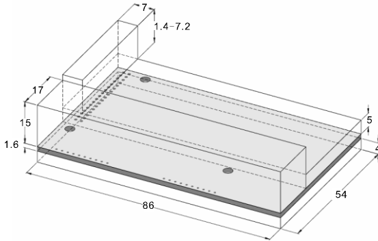
EC-TX-103 通讯卡外形尺寸图（单位：mm）
