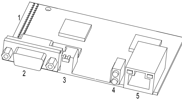
EC-TX-103 通讯卡外形图
