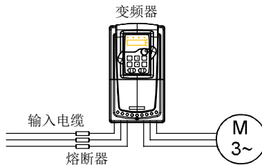
图 4-26 熔断器配置图
