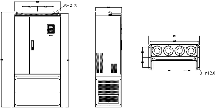
660V 250-350kW 落地安装示意图
