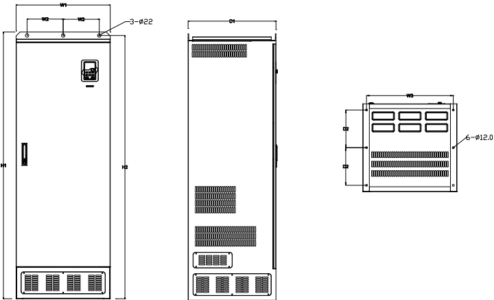
660V 400-630kW 落地安装示意图
