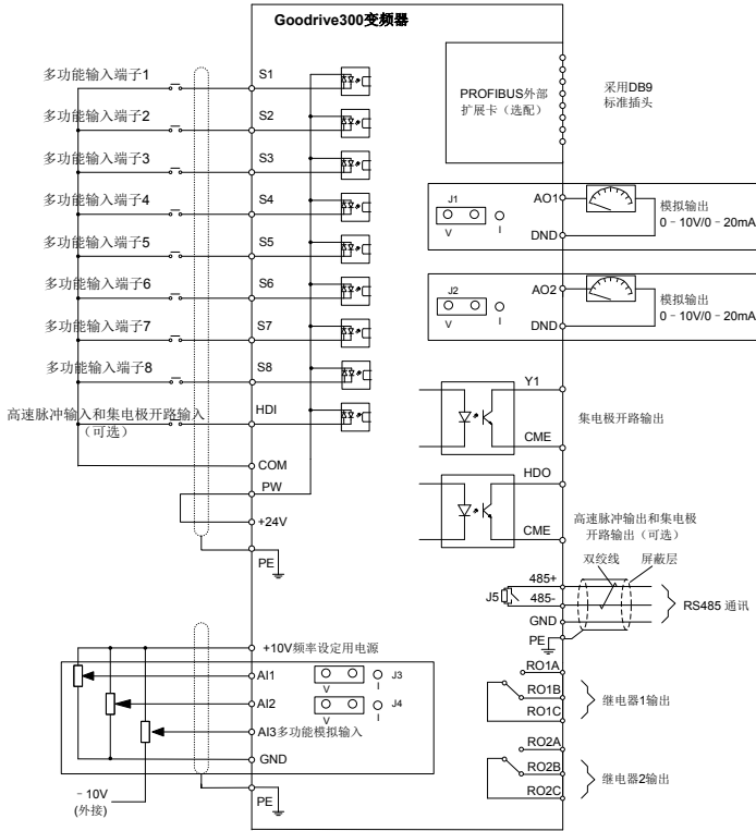
图 4-21 控制回路接线图
