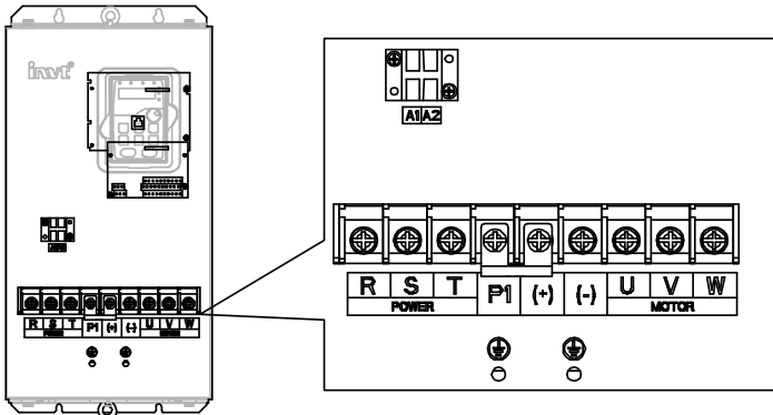
图 4-15 380V 37~55kW、500V 22~55kW 和 660V 22~45kW 主回路端子示意图
