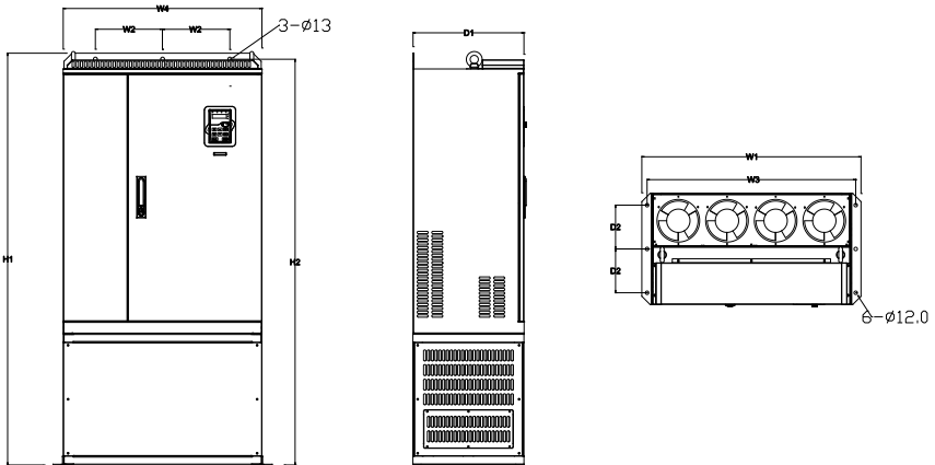
380V 220-315kW 落地安装示意图
