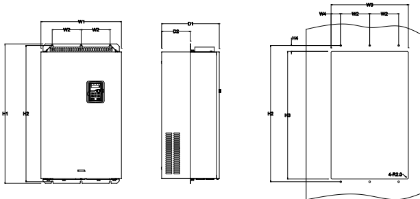
380V 132-200kW 法兰安装示意图
