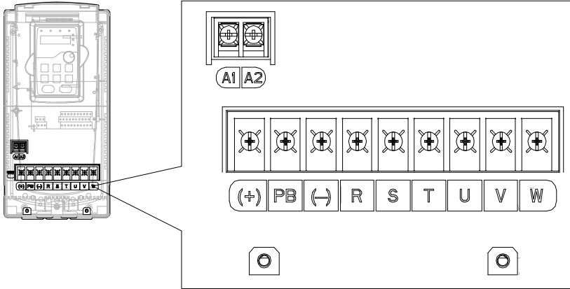
图 4-12 380V 7.5~11kW 和 500V 4~18.5kW 主回路端子示意图
