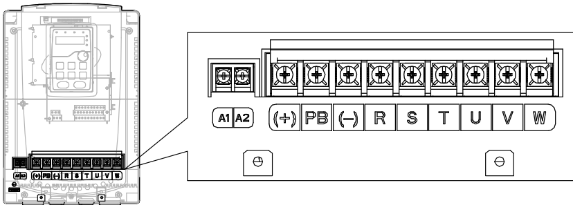
图 4-13 380V 15~18kW 主回路端子示意图
