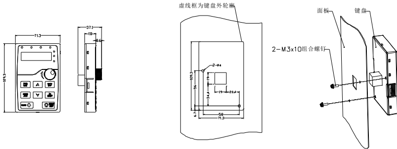
键盘无支架安装开孔尺寸及示意图
