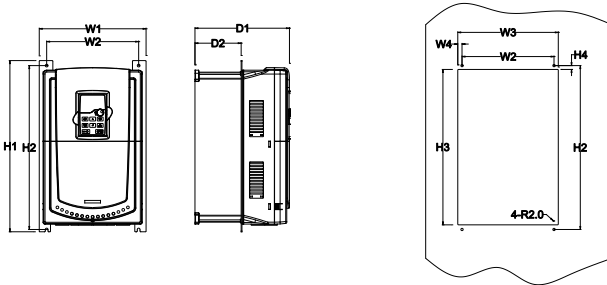
500V 4-18.5kW 法兰安装示意图
