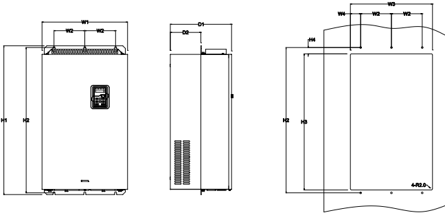
660V 160-220kW 法兰安装示意图
