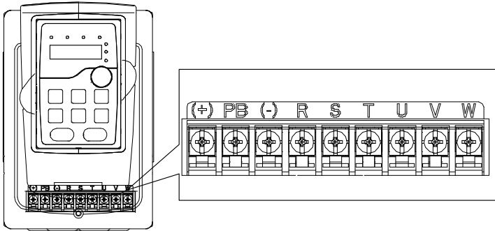
图 4-10 380V 1.5~2.2kW 主回路端子示意图
