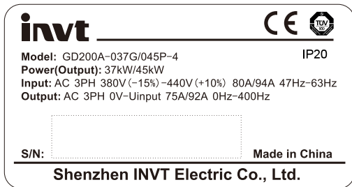
图 3.3 产品铭牌
