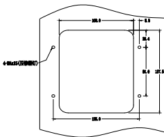
图 B.2 037G/045P~500G 键盘安装架（标配）
