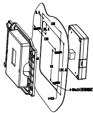
客户安装尺寸
