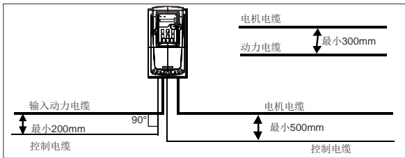
图 C.4 布线距离
