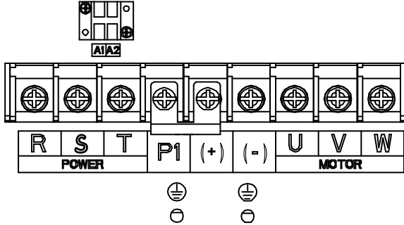
图 4.13 037G/045P~055G/075P 主回路端子示意图
