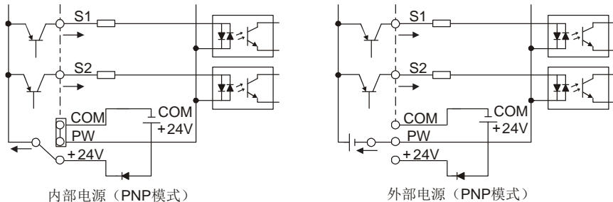
图 4.24 PNP 模式示意图
