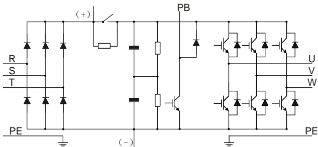
图 3.1 030G/037P 及以下主回路简图
