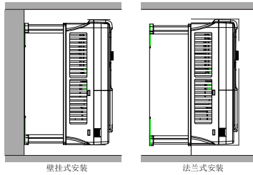
图 4.2 安装方式
