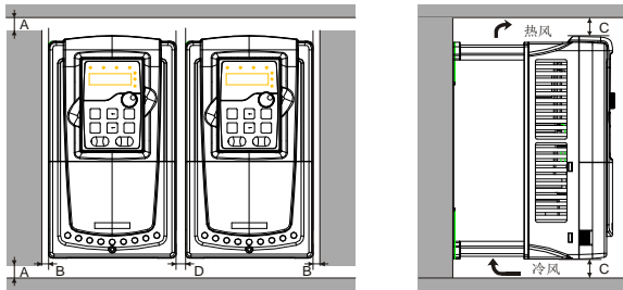
图 4.3 并行安装
