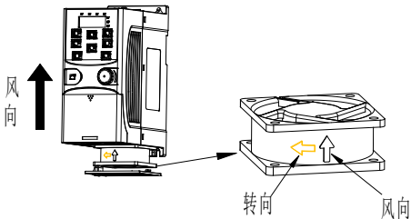
图 6.1 单相 220V 2.2kW（含）以下机器风扇维护示意图
