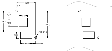
图 B.2 键盘无支架开孔示意图
