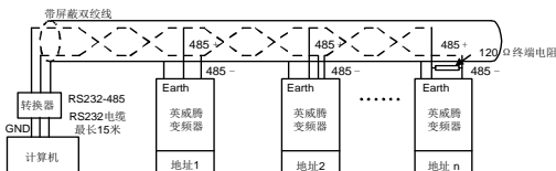
图 7.2 菊花接法运用图
