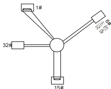
图 7.3 星形接法
