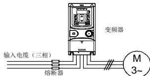
图 3.14 熔断器配置图
