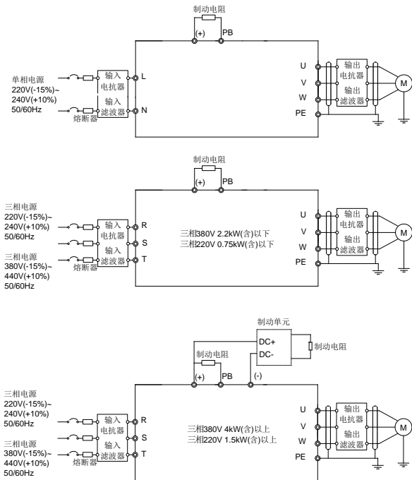
图 3.3 主回路接线图
