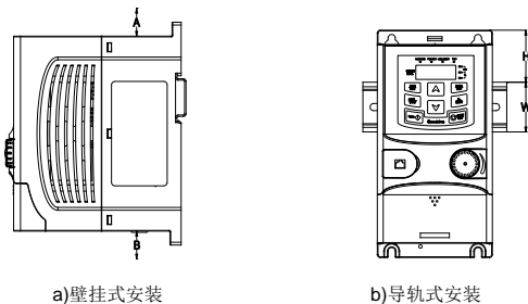
图 3.1 安装方式
