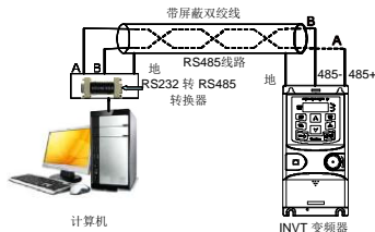
图 7.1 RS485 单机应用时的物理接线图
