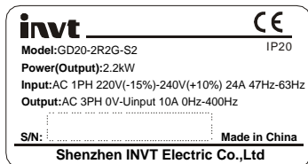
图 2.1 产品铭牌
