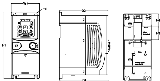
图 B.5 单相 220V/三相 380V 2.2kW(含)/ 三相 220V 0.75 kW (含)以下以下导轨安装示意图
