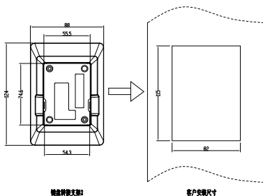
图 B.3 外形尺寸与安装尺寸图
