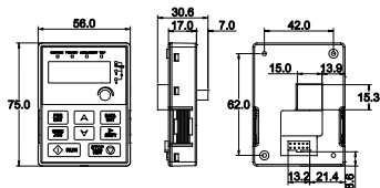
图 B.1 键盘外形图
