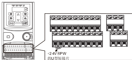
图 3.11 U 型短接位置示意图
