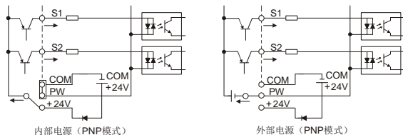
图 3.9 PNP 模式示意图
