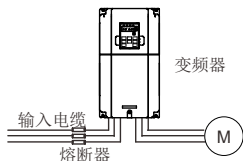
图 3.10 熔断器配置图
