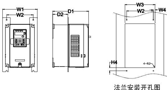
图 B.5 法兰式尺寸图
