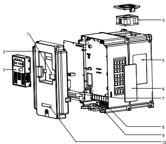
图 2.3 产品结构示意图
