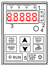
图 4.1 键盘示意图
