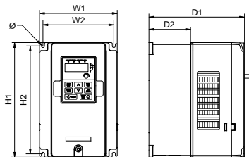
图 B.3 37kW 以下壁挂式尺寸图
