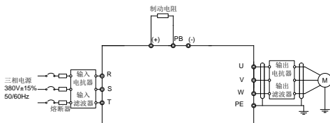
图 3.3 主回路接线图
