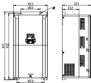
图 B.4 45~55kW 壁挂式尺寸图
