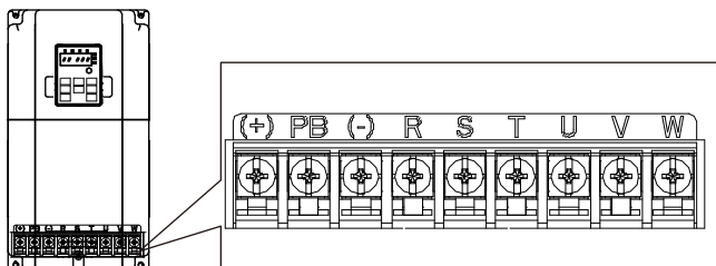
图 3.4 主回路端子示意图
