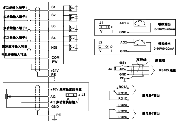
图 3.5 控制回路接线图
