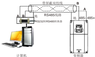
图 7.1 RS485 单机应用时的物理接线图
