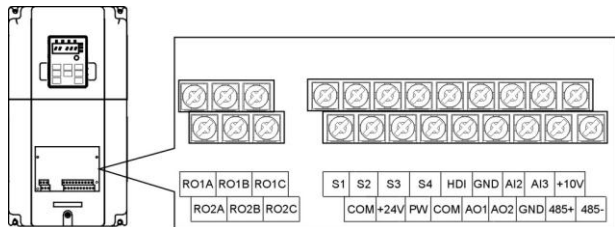
图 3.6 控制端子示意图
