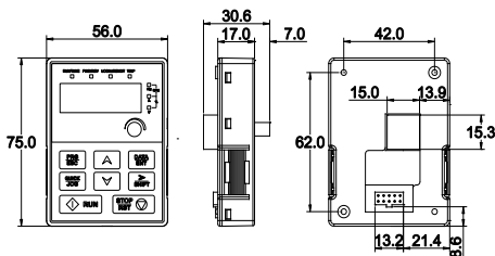
图 B.1 键盘外形图
