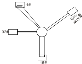
图 7.3 星形接法
