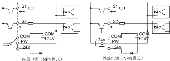
图 3.8 NPN 模式示意图
