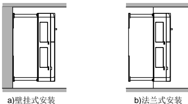
图 3.1 安装方式
