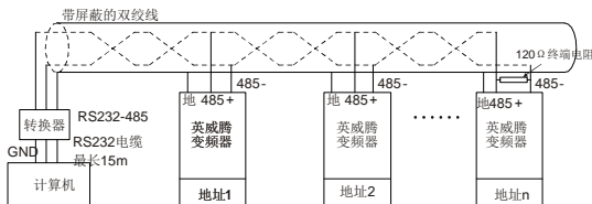
图 7.2 菊花接法运用图
