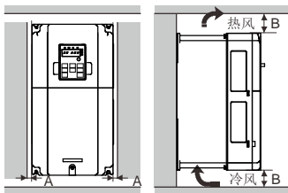
图 3.2 安装间距
