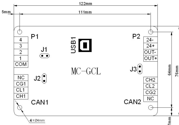
图 9-8 MC-GCL 外形尺寸图
