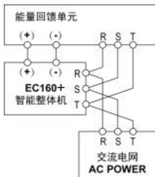
图 4-6 能量回馈单元连接图
