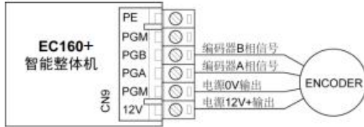
图 4-7 异步主机编码器接线图
