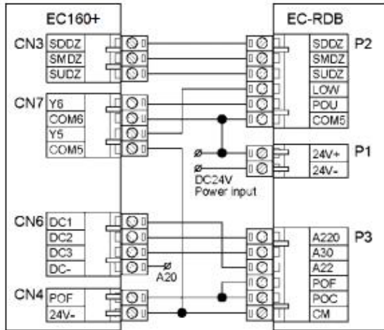
图 9-13 EC-RDB 与外围接口连接示意图
