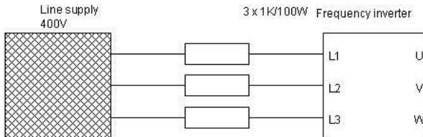
图 10-1 380V 驱动装置充电电路示例
