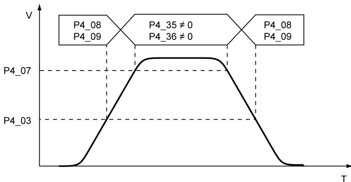
图 6-3 电流环切换示意图
