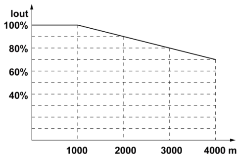
图 3-2 安装海拔高度与 EC160+电梯智能整体机降额曲线
