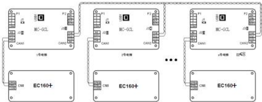
图 9-9 GCL CAN 通讯连接示意图
