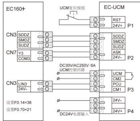
图 9-15 EC-UCM 与外围接口连接示意图
