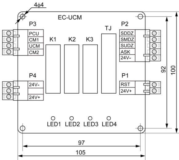
图 9-14 EC-UCM 外形尺寸图
