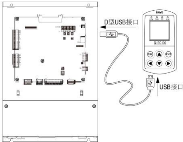
图 5-1 手持操作器的接口与 EC160+的连接图
