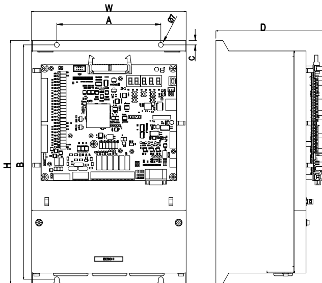
图 4-1 EC160+电梯智能整体机安装尺寸示意图
