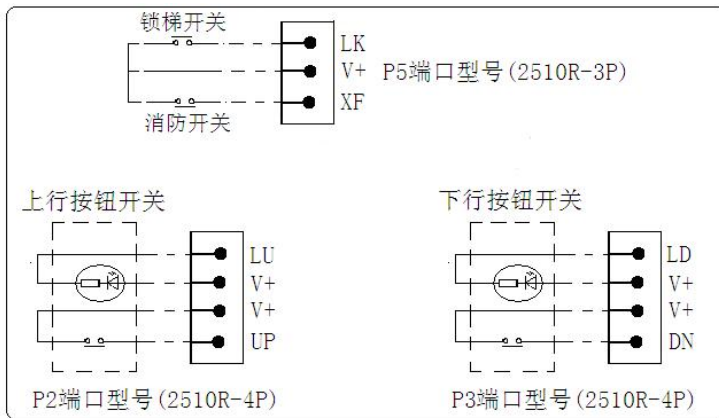
图 9-7 呼梯显示板开关连接图
