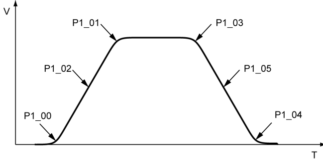
图 6-1 直接停靠 S 曲线调整参数图
