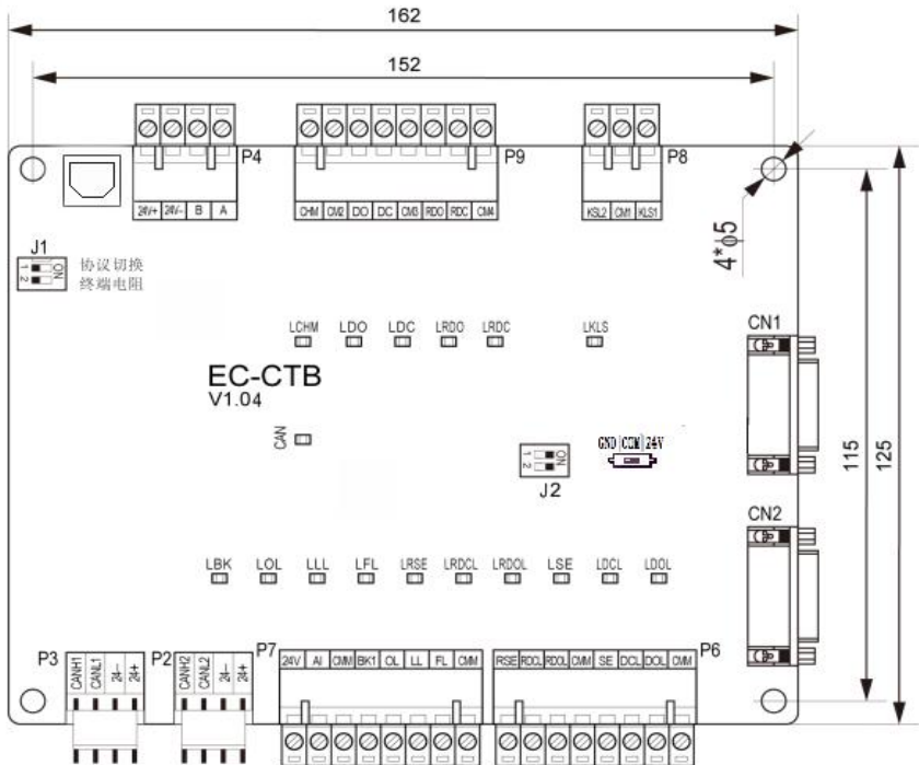
图 9-1 顶板安装尺寸
