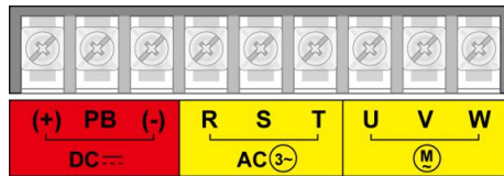
图 4-3 EC160+电梯智能整体机主回路端子排的布局(4kW~15kW)
