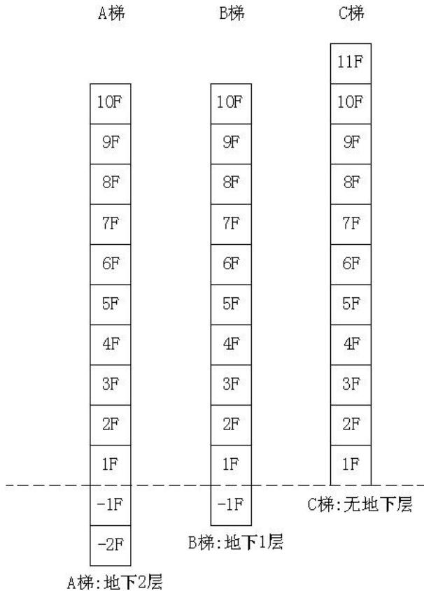
图 9-11 群控偏置楼层分布图
