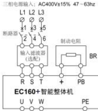
图 4-5 制动电阻和制动单元连接图
