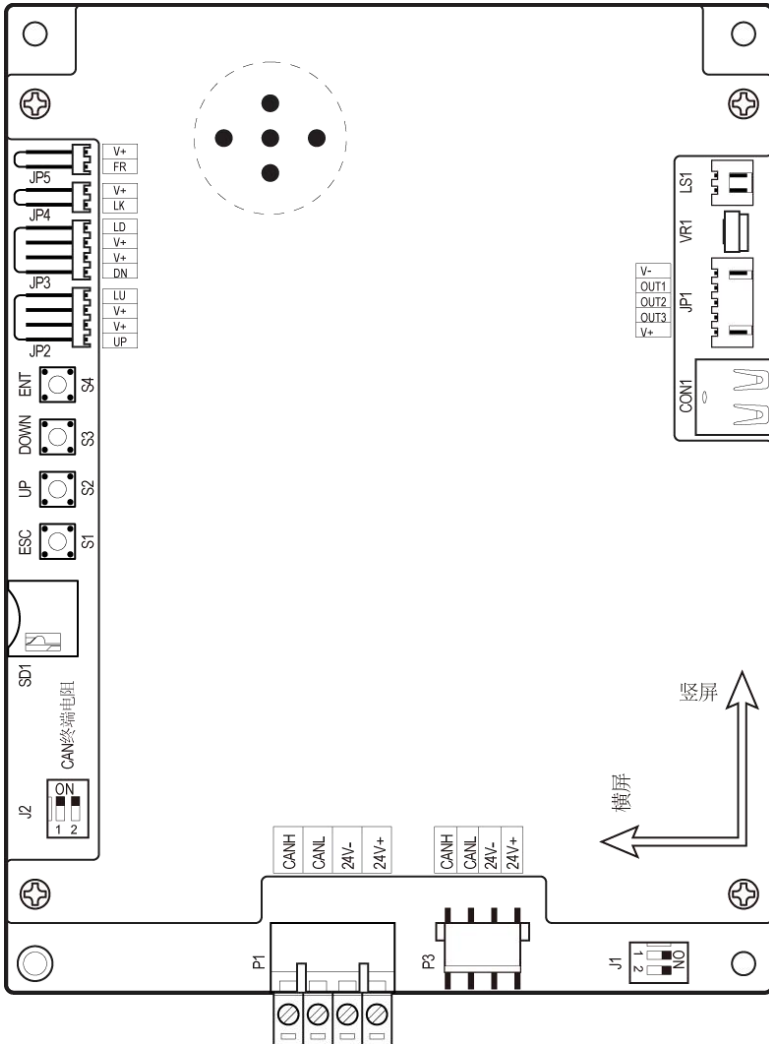
图 9-17 LM21-070 背面端口示意图
