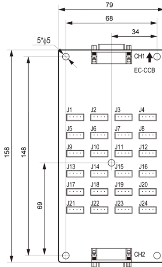
图 9-2 指令板安装尺寸
