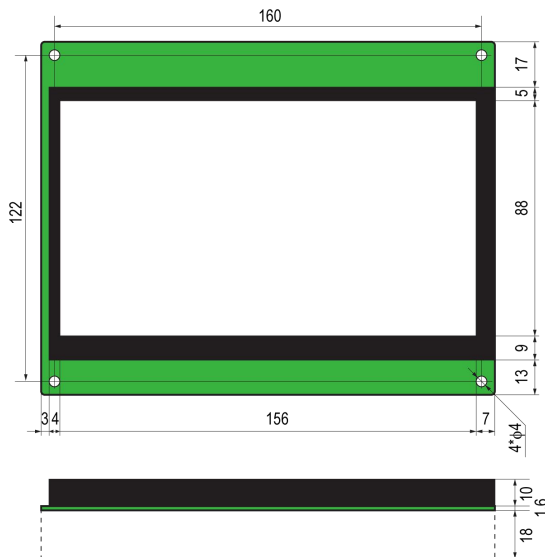
图 9-16 LM21-070 外形尺寸图
