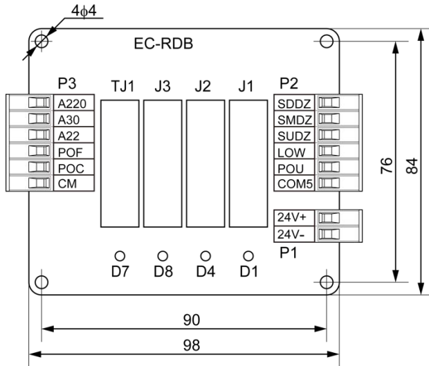
图 9-12 EC-RDB 外形尺寸图
