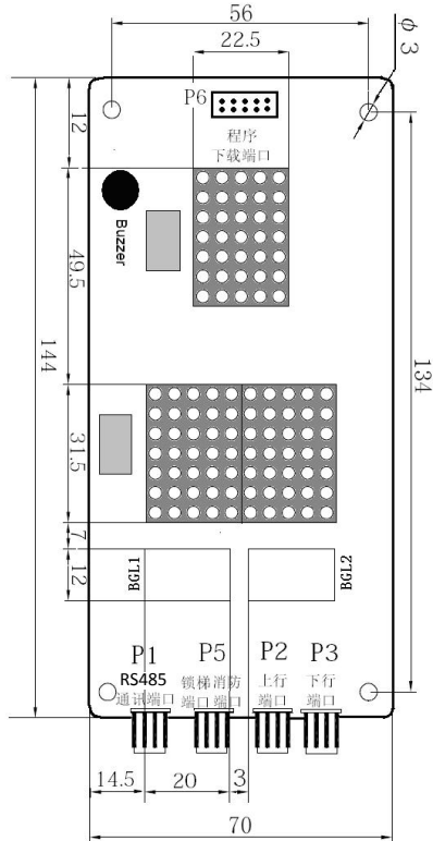
图 9-6 显示板安装尺寸
