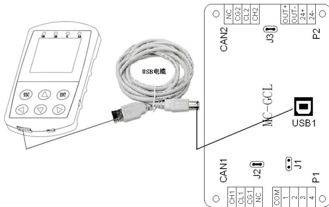
图 9-10 手持操作器的接口与 MC-GCL 的连接图
