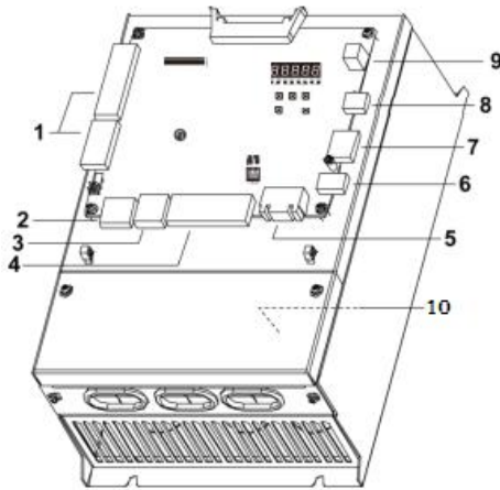
图 4-2 EC160+电梯智能整体机端口
