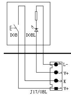
图 9-4 开门按钮及指示灯接线图
