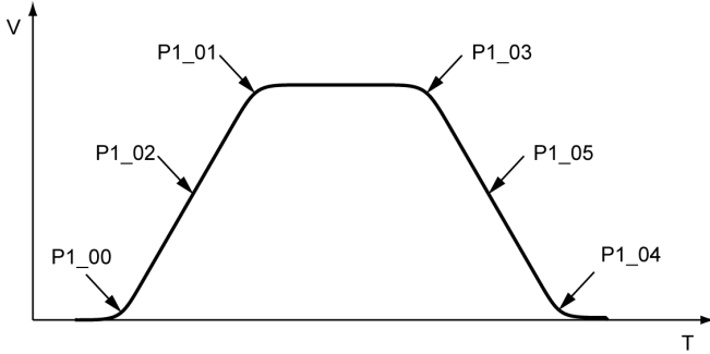
图 8-1 S 曲线调整示意图
