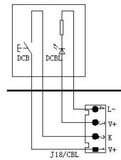
图 9-5 关门按钮及指示灯接线图
