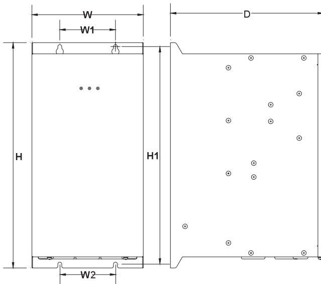
图 3 320A-400A 尺寸图
