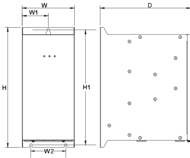
图 2 110A-220A 尺寸图
