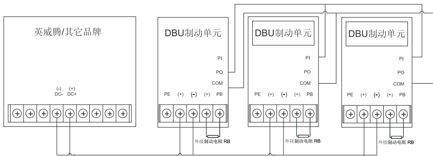
图 7 制动单元并联运行与变频器连线图
