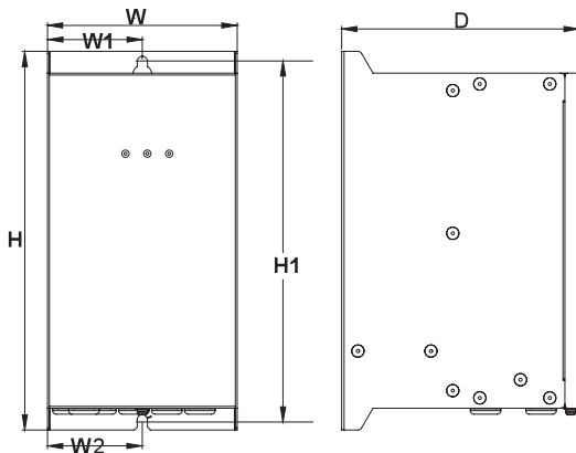
图 1 60A 尺寸图
