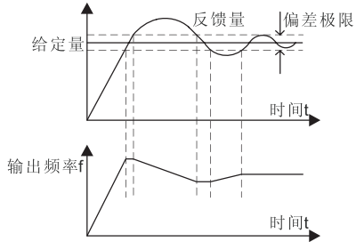
图 6-23 偏差极限与输出频率的对应关系
