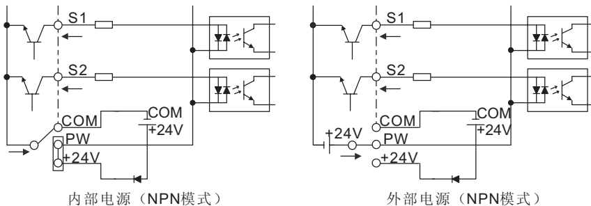
图 4-17 共发射极模式
