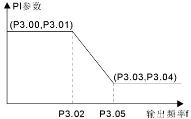
图6-5 PI参数示意图
