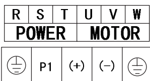
图 4-6 主回路接线端子图 (132~315kW)
