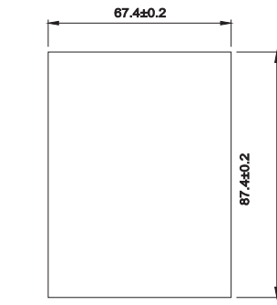
图 A-10 外引键盘（小）的开口尺寸
