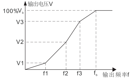
图6-8 V/F曲线设定示意图
