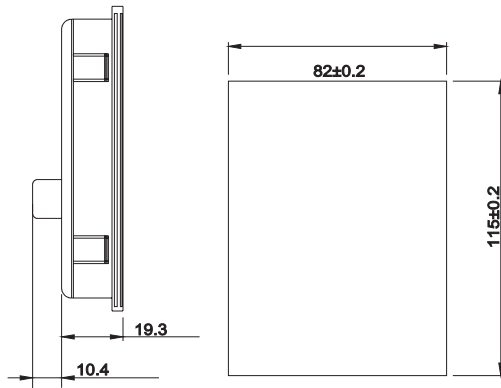
图 A-12 外引键盘 (大) 的开孔尺寸
