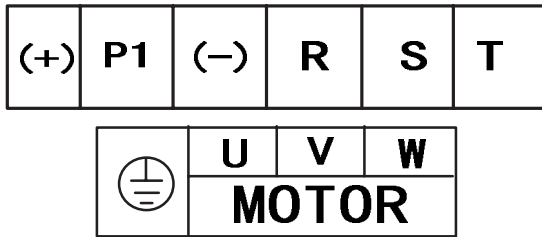
图 4-11 主回路接线端子图（22kW 以上，为上进出结构）
