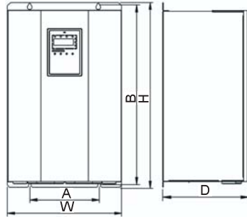
图 A-5 11kW~18.5kW 机型外形尺寸 (230V)
