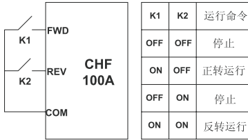
图 6-10 两线式控制（使能与方向分离）
