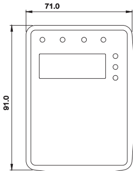
图 A-9 外引键盘（小）的安装尺寸
