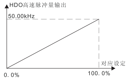
图 6-15 给定量与高速脉冲量输出的对应关系
