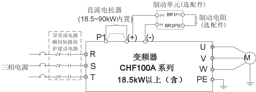
图 4-14 18.5kW以上（含）主回路接线图
