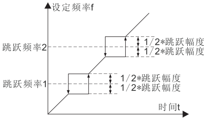
图6-17 跳跃频率示意图
