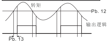
图 6-30 过转矩控制示意图
