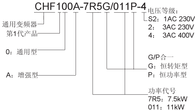
图 1-1 变频器铭牌说明
