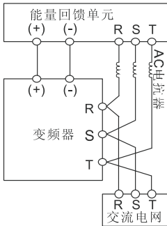
图 4-21 能量回馈单元连接图
