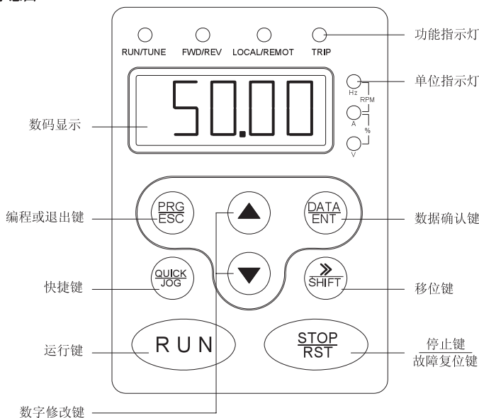
图 5-1 键盘示意图
