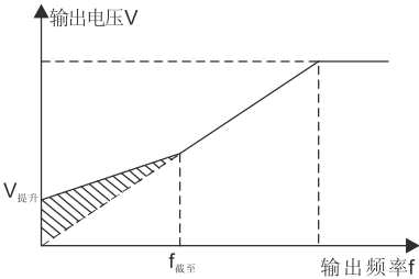
图6-7 手动转矩提升示意图
