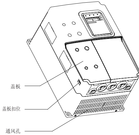
图 1-2 15kW 及以下变频器各部件名称
