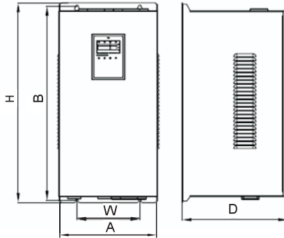
图 A-6 22~55kW 机型的外形尺寸 (230V)
