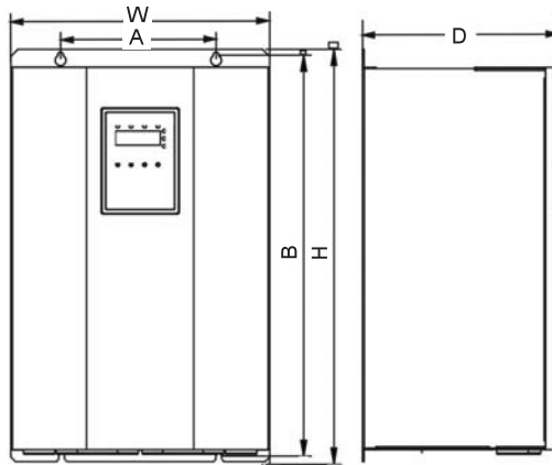
图 A-2 18.5~110kW 机型外形尺寸（400V）
