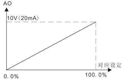
图 6-14 给定量与模拟量输出的对应关系
