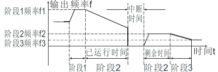
图6-26 简易PLC启动方式1
