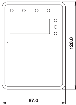
图 A-11 外引键盘 (大) 的安装尺寸
