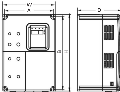
图 A-5 15kW 及以下机型的外形尺寸
