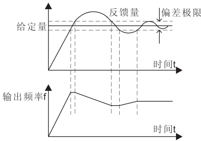
图6-19 偏差极限与输出频率的对应关系
