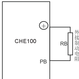
图 B-1 制动电阻的安装
