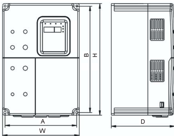
图 A-6 7.5kW 及以下机型的外形尺寸
