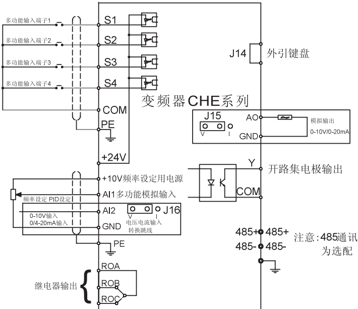
图 4-19 控制回路接线图
