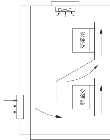
图 A-14 多台变频器的安装
