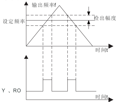
图6-17 频率到达检出幅值示意图
