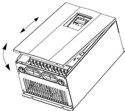
图 A-16 钣金盖板的拆卸和安装示意图
