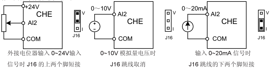
图 4-24 单相 0.4~0.75kW 控制端子连线说明图
