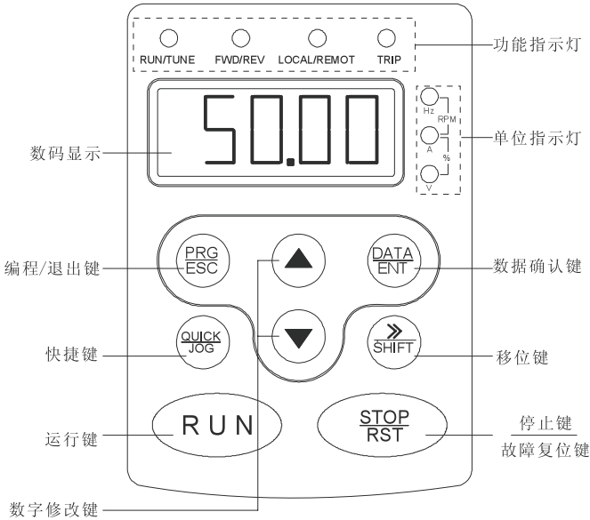
图 5-1 键盘示意图
