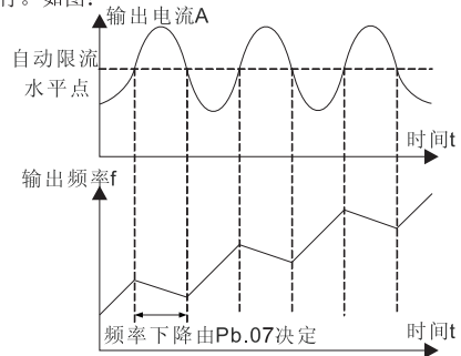
图6-23 过流失速功能
