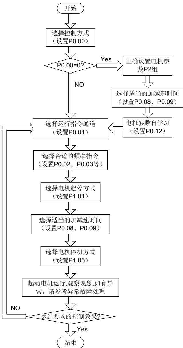
图 5-6 快速调试流程图
