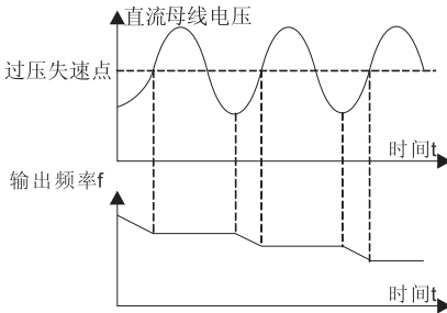
图6-22 过压失速功能
