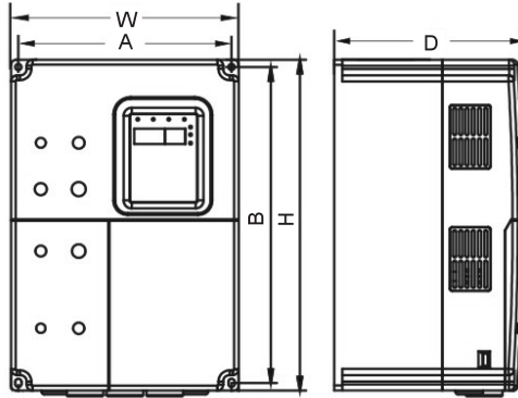
图 A-1 15kW 及以下机型的外形尺寸
