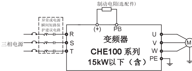
图 4-17 15kW以下（含）主回路接线图
