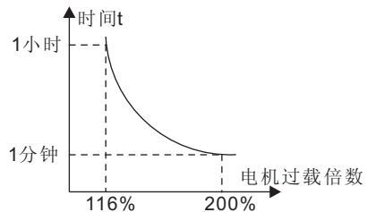
图6-21 电机过载保护系数设定
