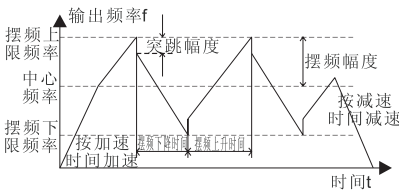
图6-15 摆频运行示意图
