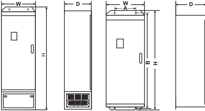
图 A-3 132kW~500kW 机型(无底座)外形尺寸
