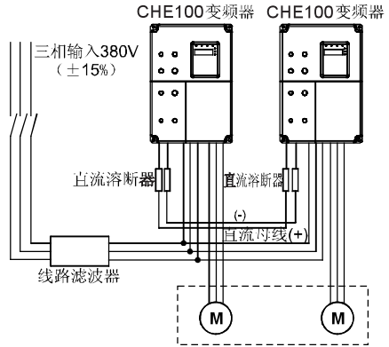
图 4-23 共直流母线的连接
