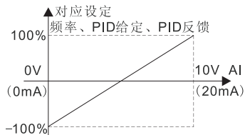
图6-12 模拟给定与设定量的对应关系
