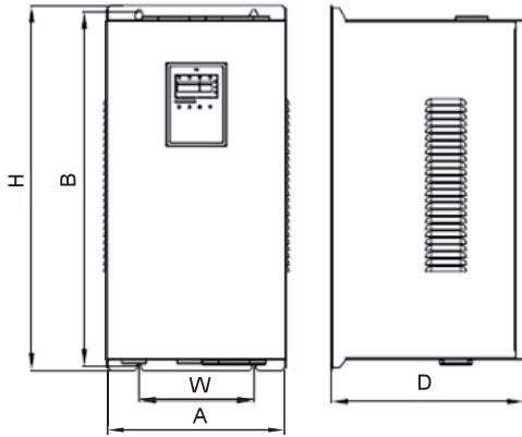
图 A-8 22~55kW 机型的外形尺寸
