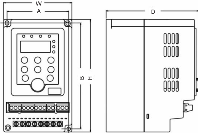
图 A-4 0.4~0.75kW 标准外形尺寸
