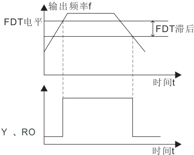
图6-16 FDT电平示意图
