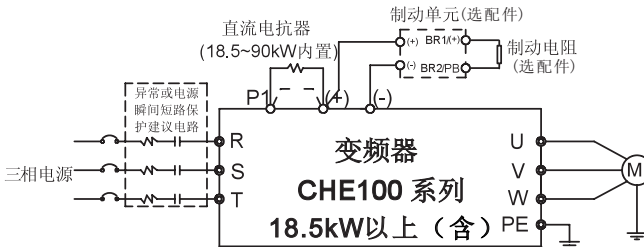
图 4-18 18.5kW以上（含）主回路接线图
