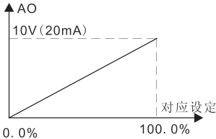
图6-13 给定量与模拟输出对应关系
