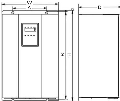
图 A-2 18.5kW~110kW 机型外形尺寸
