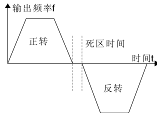
图6-4 正反转死区时间示意图
