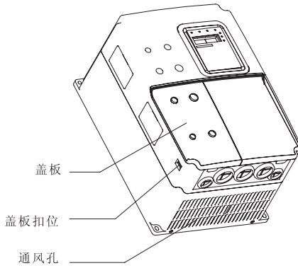
图 1-2 15kW 及以下变频器各部件名称
