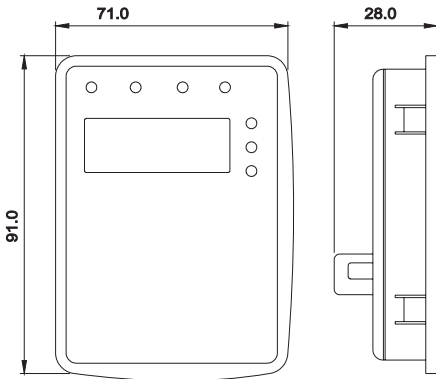
图 A-9 外引键盘（小）的安装尺寸
