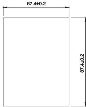
图 A-10 外引键盘（小）的开孔尺寸
