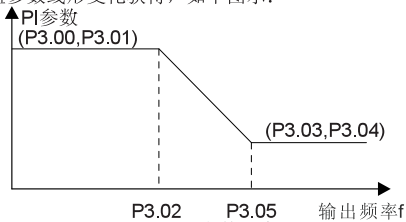
图 6-5 PI 参数示意图
