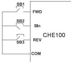
图 6-11 三线式控制模式 2
