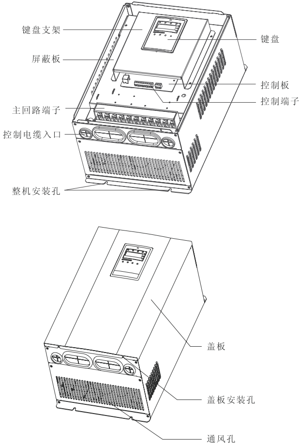
图 1-3 18.5kW~110kW 变频器各部件名称
