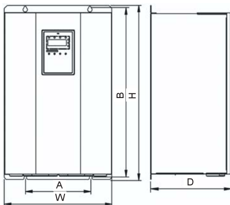
图 A-7 11kW~18.5kW 机型外形尺寸
