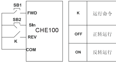
图 6-10 三线式控制模式 1
