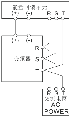
图 4-22 能量回馈单元连接图
