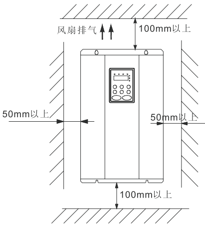
图 A-13 安装的间隔距离
