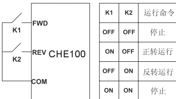
图 6-8 两线式控制 1（使能与方向合一）
