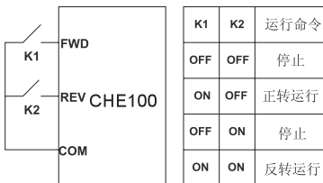
图 6-9 两线式控制 2（使能与方向分离）
