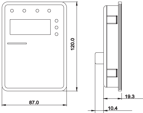
图 A-11 外引键盘（大）的安装尺寸
