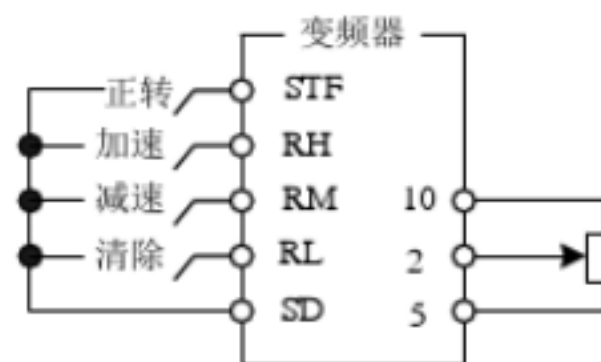
远端控制设定的接线图示例
