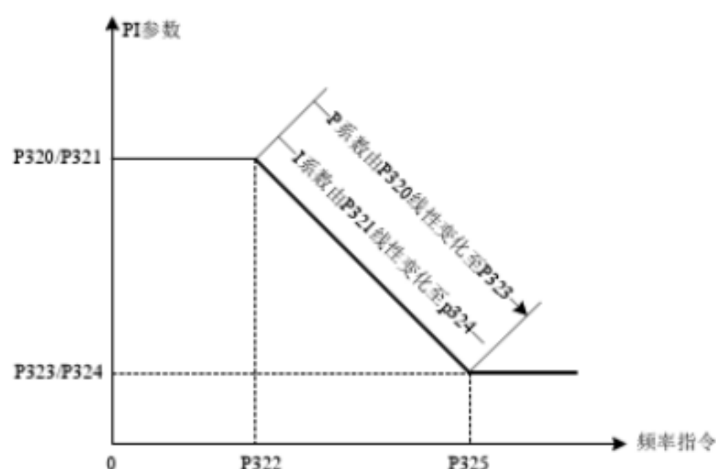
两组 PI 参数变化示意图
