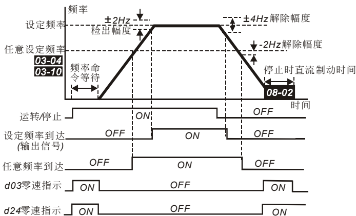
多机能端子与频率到达输出时序图
