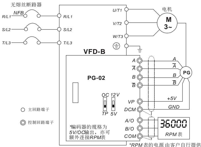
PG-02与编码器的连接
