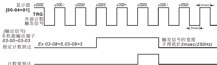
外部计数端子与计数到达时序图
