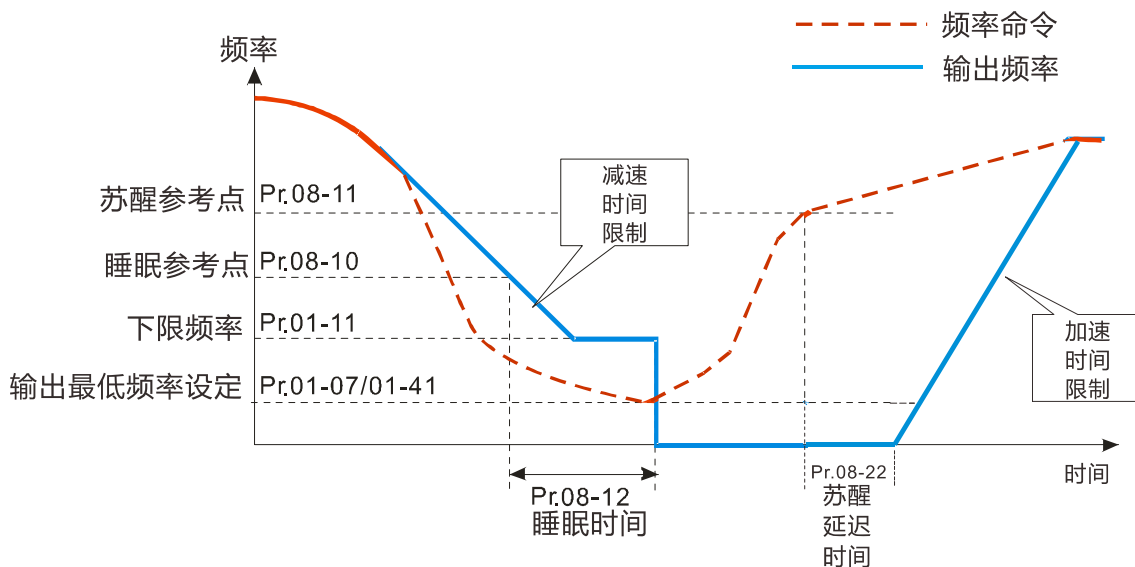
内部PID计算频率命令
