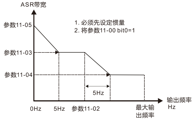
ASR调整-自动增益
