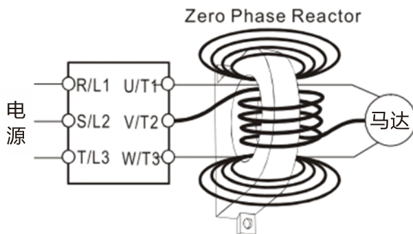
图 B 零相电抗器多匝安装示意图
