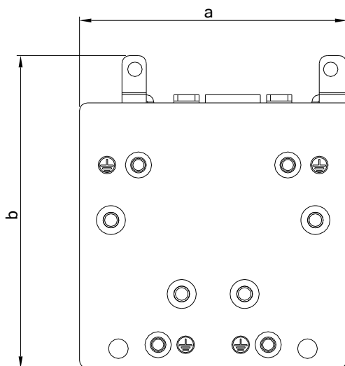
EMC 接地铁板 外观尺寸
