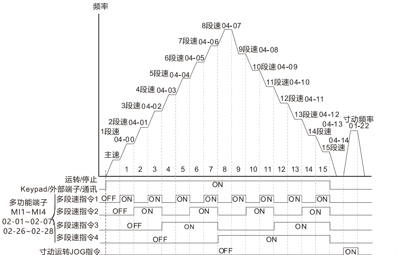
多段速与外部端子动作时序图
