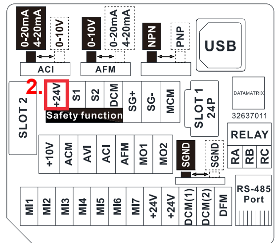
控制端子各端子位置图
