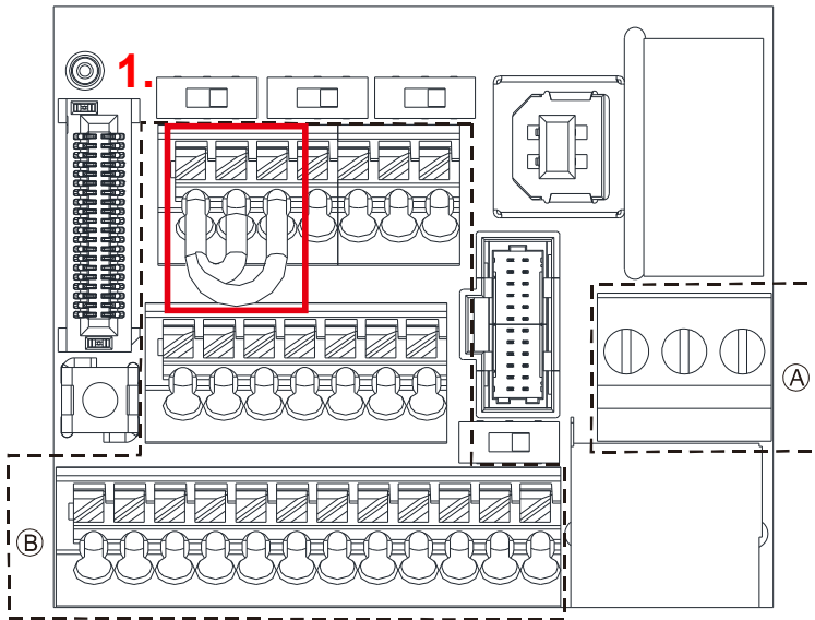
控制端子分布图
