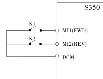
图 6-8 两线式运转模式2
