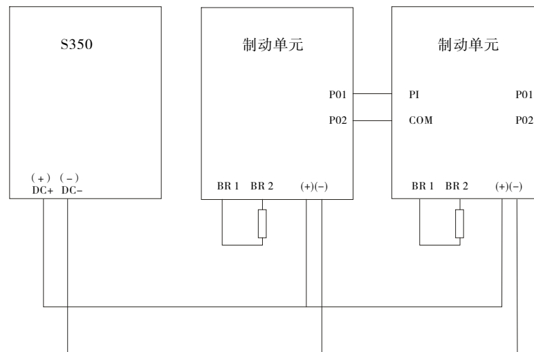
图1-4 制动单元的并联连接
