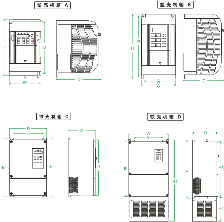
7.5KW(含7.5KW) 以下的外形尺寸表
