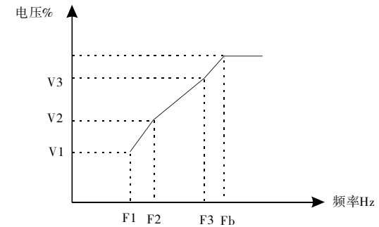
图6-5 V/F曲线设定示意图
