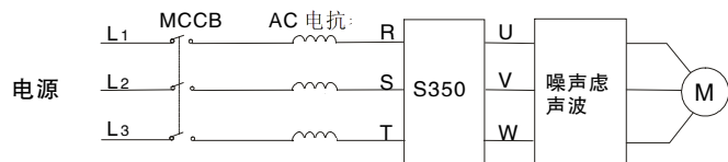
图3-5 主回路电机侧连接图
