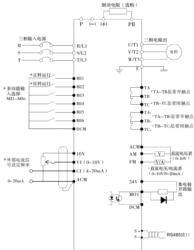
图3-4 标准接线图
