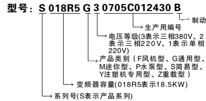
图1-1 变频器铭牌说明
