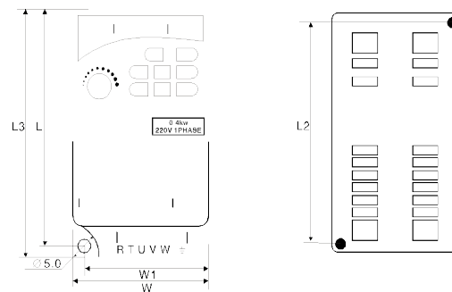
附录D: 机箱及键盘尺寸 塑壳机箱
