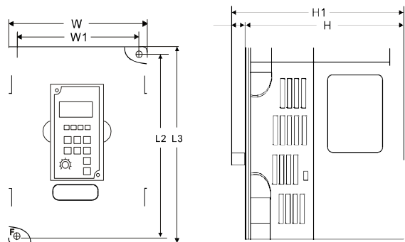
附录C: 机箱及键盘尺寸 塑壳机箱
