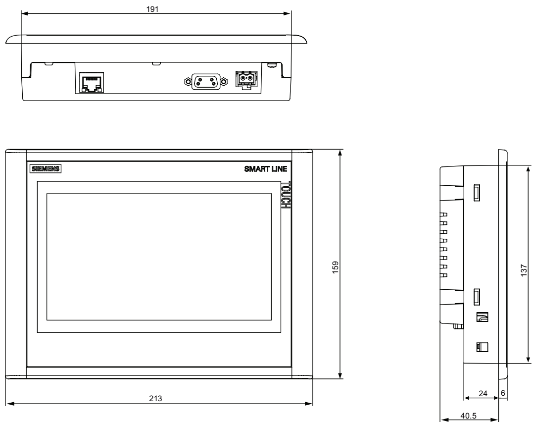
图 3-1 Smart 700 IE 的尺寸设计 (mm)
