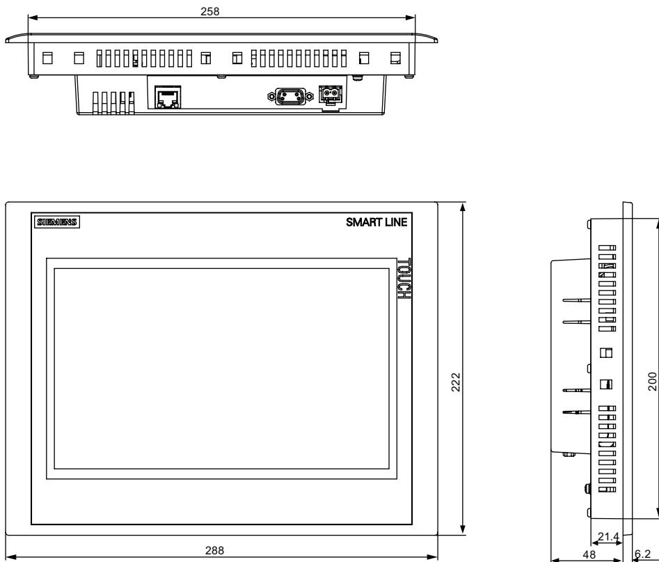
图 3-2 Smart 1000 IE 的尺寸设计 (mm)
