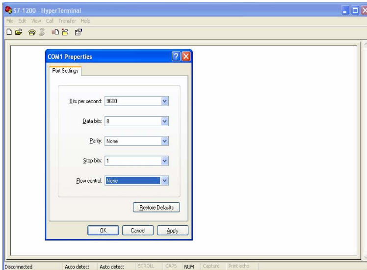
图 21：超级终端的端口设置
