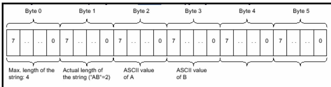
图 11: String 存储格式
