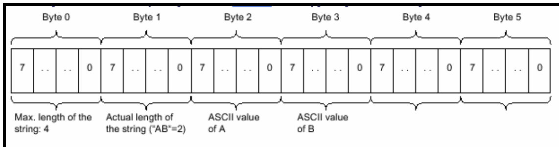
图 19: String 存储格式
