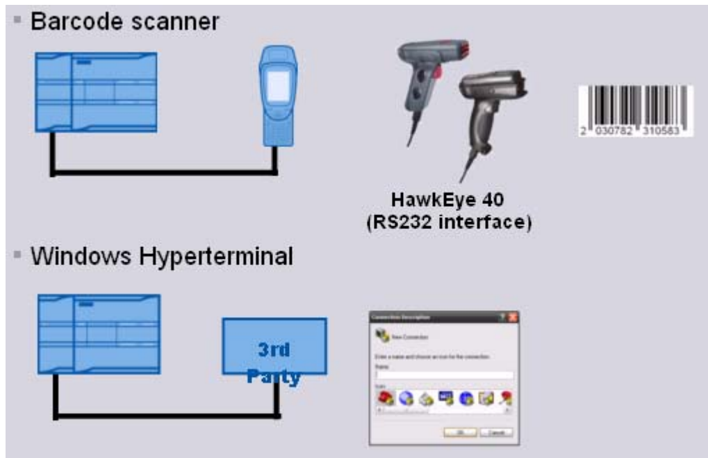
图 1:控制系统原理
