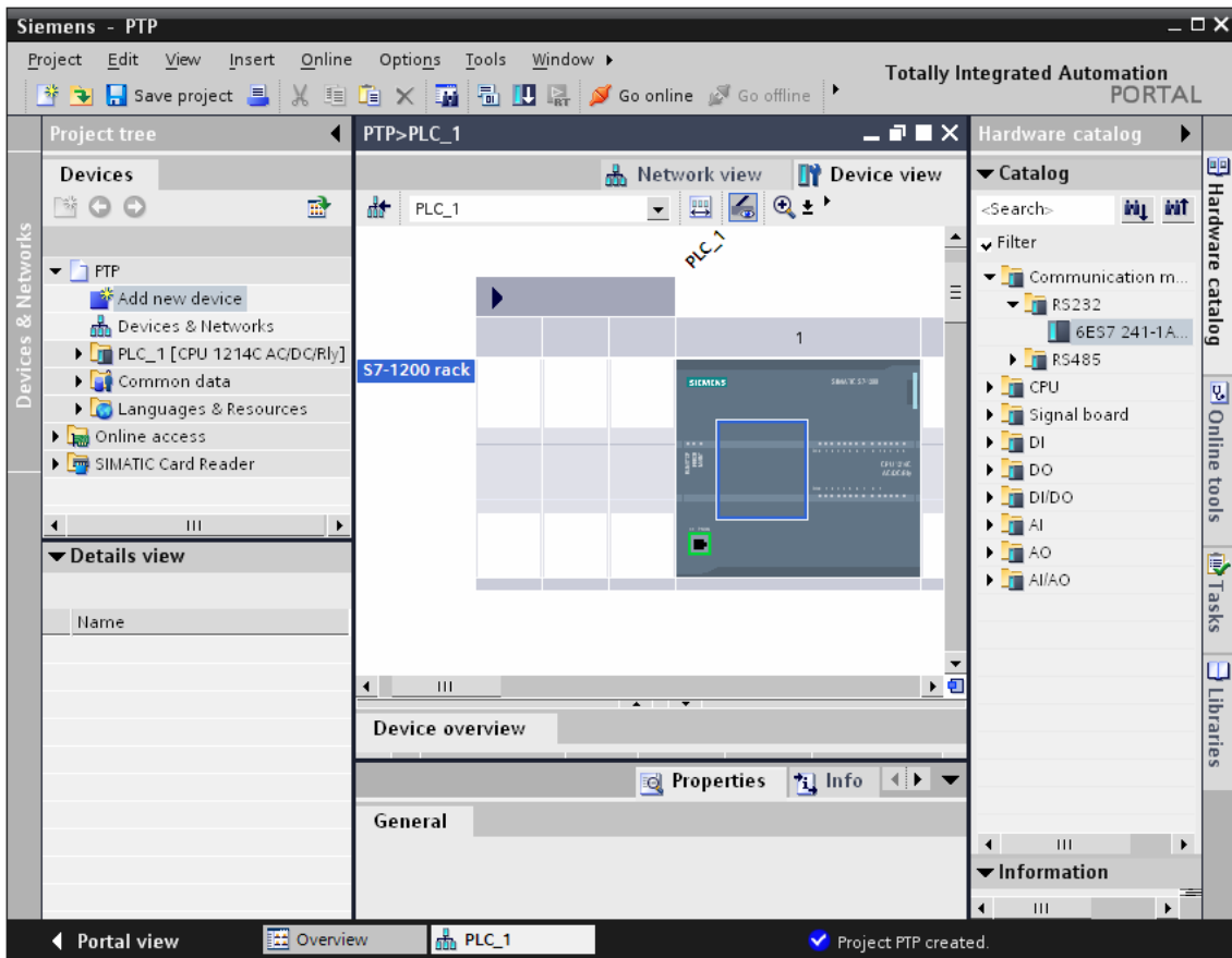
图 5： PLC 硬件组态
