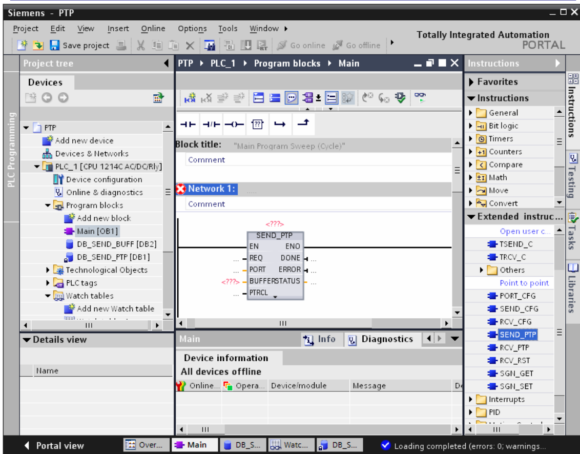
图 7： 调用发送功能块
