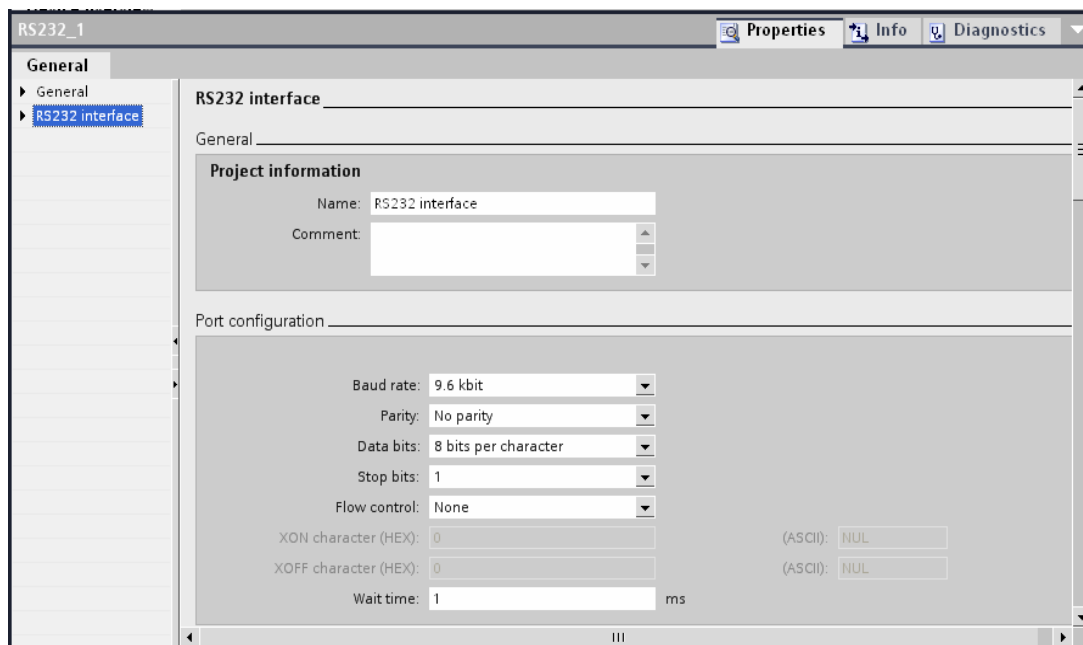
图 6: RS232 接口配置
