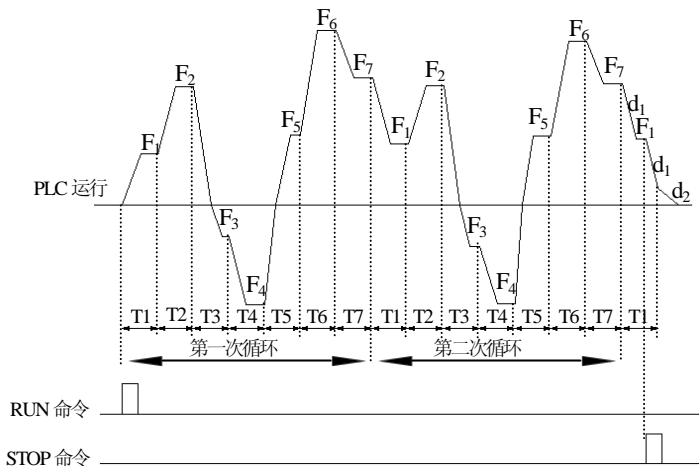
图 6-42 PLC 连续循环方式
