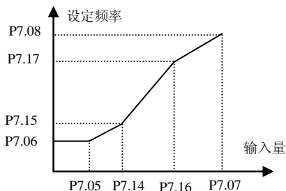
图 6-36 拐点有效时的设定频率 1
