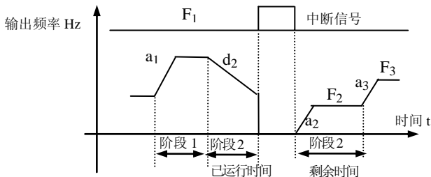
图 6-43 PLC 起动方式 1
