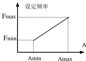
(1)正作用特性
