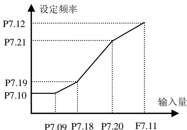
图 6-38 拐点有效时的设定频率 2
