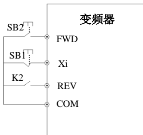
图 6-24 三线式运转模式 2
