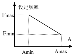
(2)反作用特性
