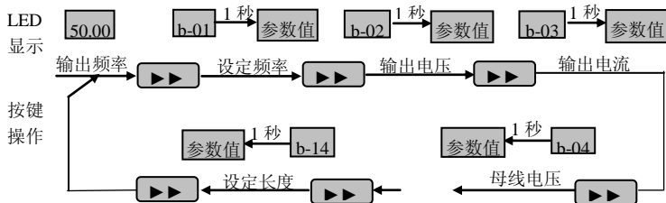
图 4-6 运行状态参数显示操作示例
