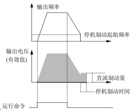
图 6-12 减速停车+直流制动示意图
