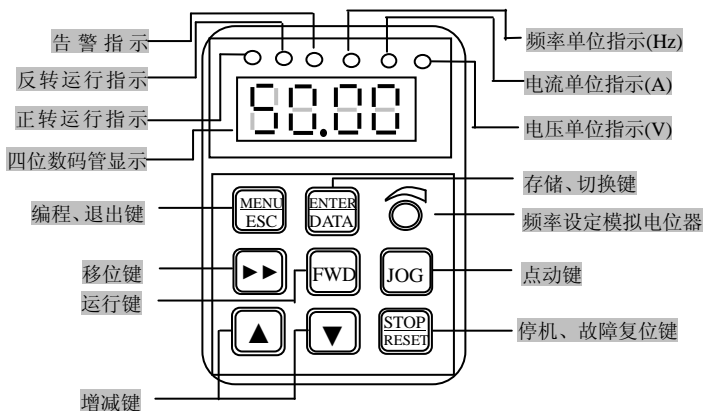
图 4-2 操作键盘示意图
