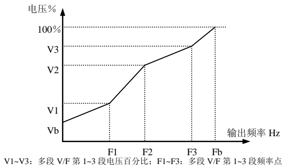
图 6—8 用户定义 V/F 曲线
