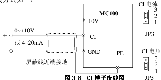
图 3-8 CI 端子配线图
