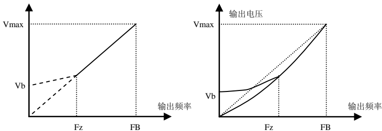
(a) 恒转矩曲线转矩提升示意图
