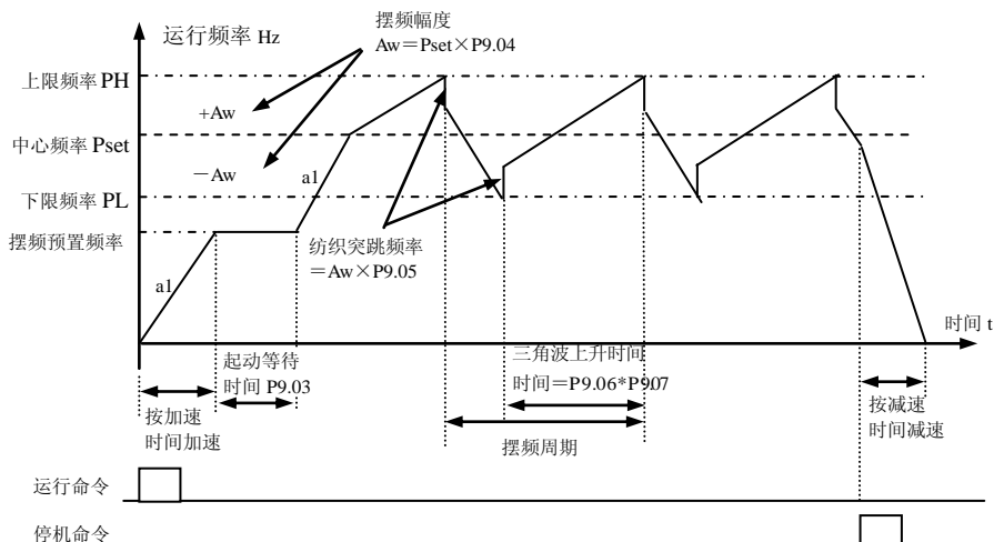
图 6-44 摆频运行示意图
