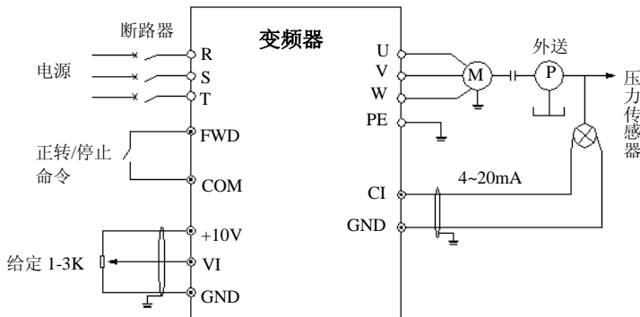
图 6-32 内置 PI 模拟反馈控制系统示意图
