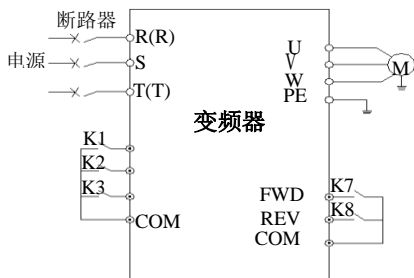
图 6-19 多段速运行接线图
