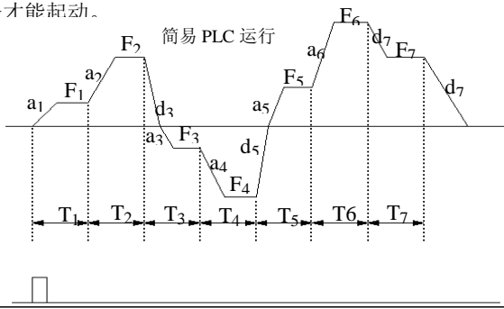
图 6-40 PLC 单循环后停机方式
