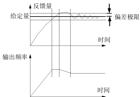
图 6-33 偏差极限示意图
