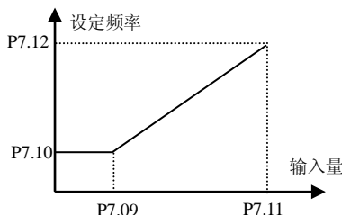
图 6-37 拐点无效时的设定频率
