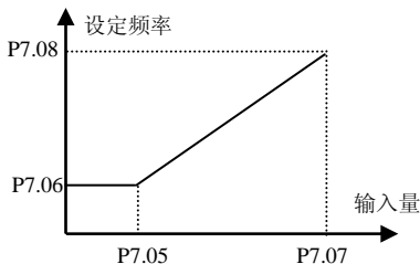
图 6-35 拐点无效时的设定频率 1
