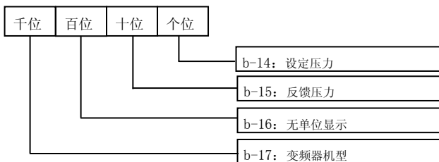
图 6-17 显示参数选择 2 示意图
