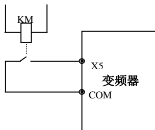
图 6-20 外部设备故障输入示意图
