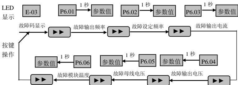
图 4-10 故障状态查询操作示例
