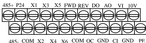
图 3-7 控制板端子排列顺序图
