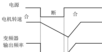
图 6-9 转速跟踪再启动示意图
