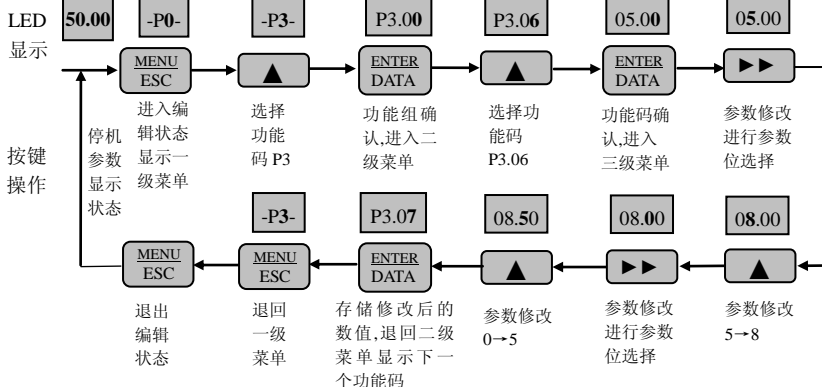
图 4-7 参数编辑操作示例
