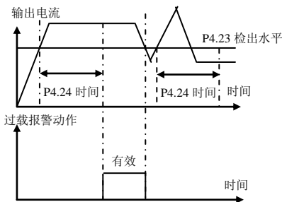
图 6-29 过载报警
