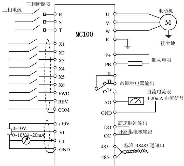
图 3-5 基本配线图
