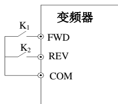
图 6-21 两线式运转模式 1
