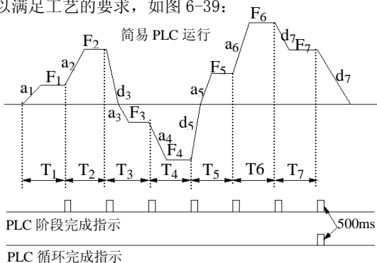
图 6-39 简易 PLC 运行图
