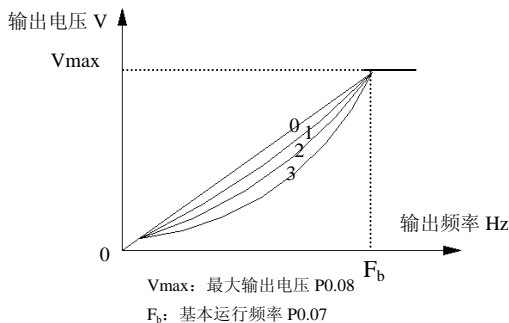
图 6—7 V/F 曲线
